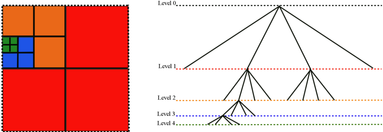
Figure 5-1 : Discretisation quadtree et la structure logique correspondante
