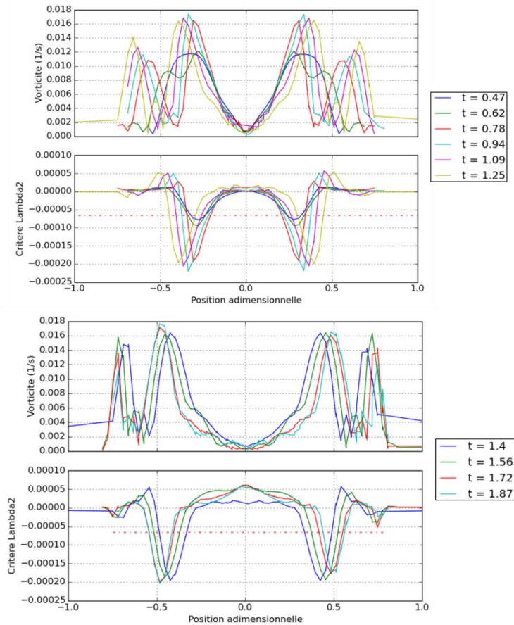
Figure 8-36 : Valeurs de vorticit  de l'anneau de vortex (Haut) et la valeur correspondante au crit re \lambda_2 (bas)   diff rents instants de temps pour un We = 4.45
