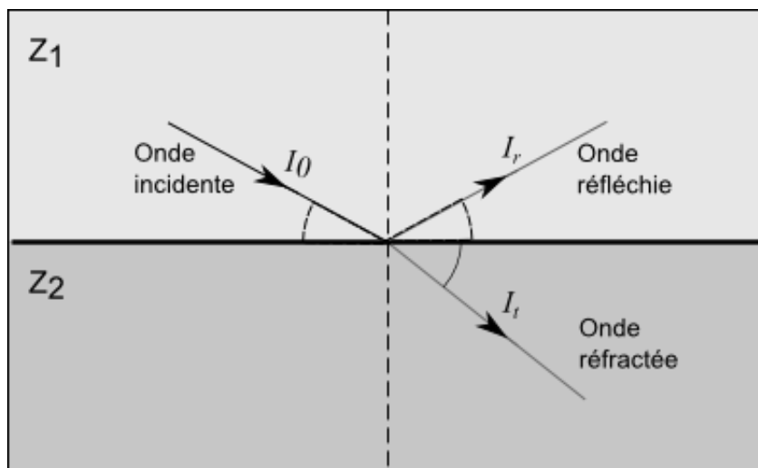
Figure 29 - Illustration des principes de réflexion et de réfraction de l'onde ultrasonore. A l'interface entre les deux milieux, une onde incidente d'intensité I_0 est réfléchie en une onde I_r et réfractée en une onde I_t , d'après [84].
