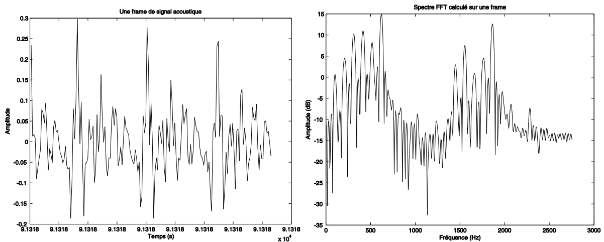
Figure 13 - Une trame de signal et le spectre calculé sur cette trame.
