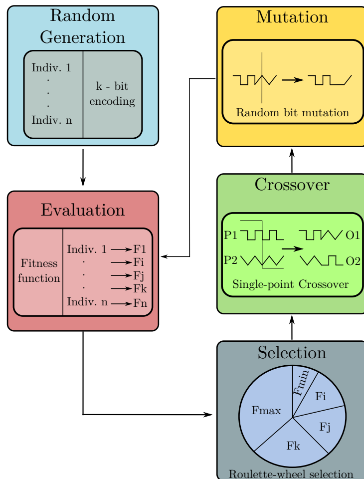
Figure 1.4: Algorithme génétique
