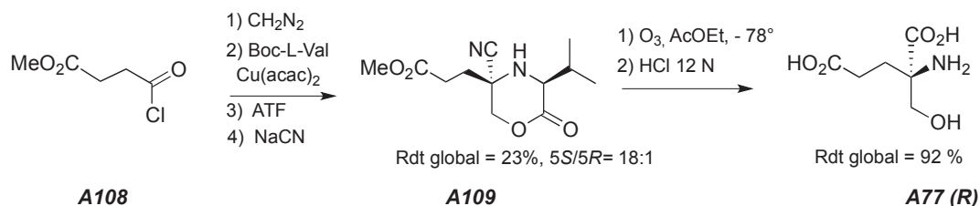
Schéma 1-36 : Synthèse de l'acide (2R)-α-hydroxyméthyl glutamique par réaction de Strecker
