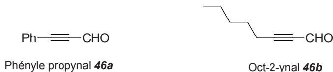
Schéma 4-33 : Ynals testés
