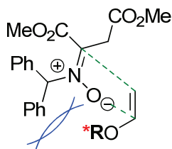
Schéma 2-42 : Facteurs défavorisant l'approche endo
