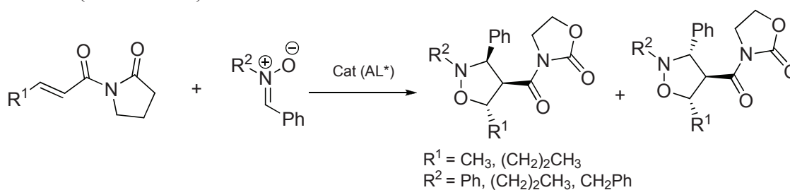
Schéma 4-1 : CD-1,3 de 3-alcénoyle-2-oxazolidinones avec des nitrones catalysée par des complexes de Ti
