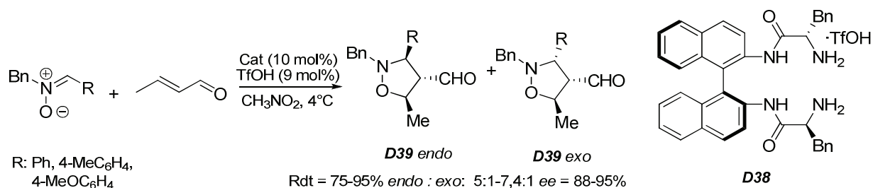
Schéma 4-10 : CD-1,3 énantiosélective entre les diaryls aldonitrones et le (E) crotonaldéhyde en présence du catalyseur D38
