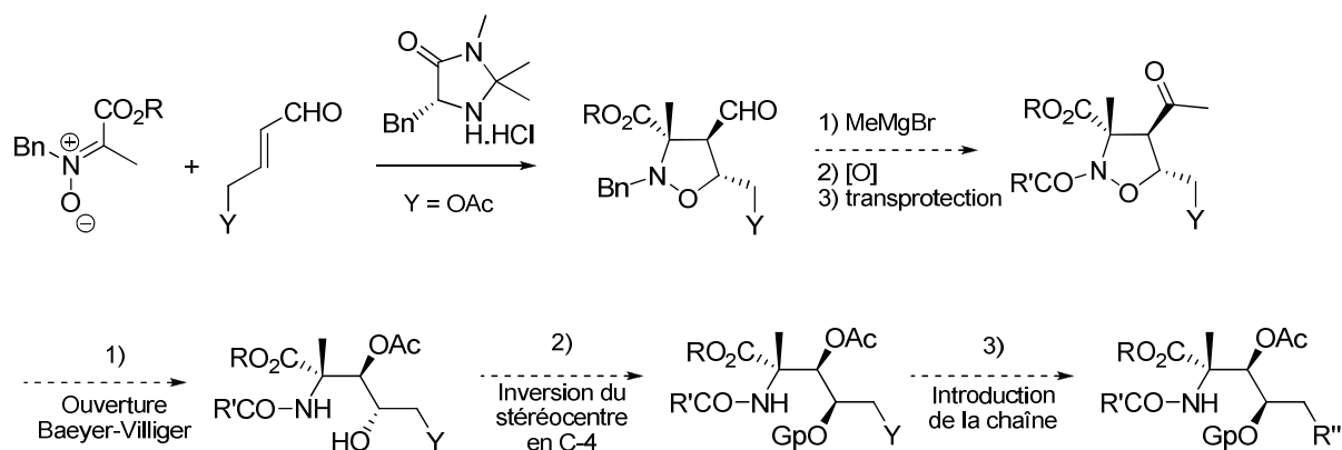
Schéma 5-19 : Schéma de synthèse global envisagé pour la nor-hydroxy myriocine
