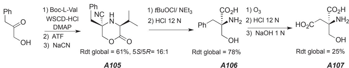
Schéma 1-35 : Synthèse de l'α-carboxyméthyl sérine A107 par réaction de Strecker
