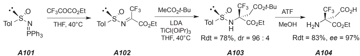
Schéma 1-34 : Synthèse asymétrique du mono ester (S) α-trifluorométhyl aspartique
