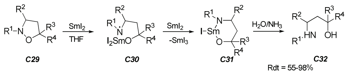
Schéma 3-8 : Rupture de la liaison N-O par \text{SmI}_2
