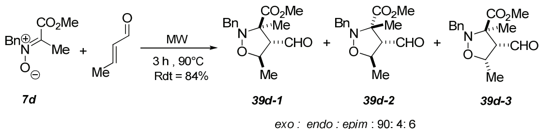
Schéma 4-18 : CD-1,3 entre la nitrone 7d et le ( E ) crotonaldéhyde en conditions thermiques
