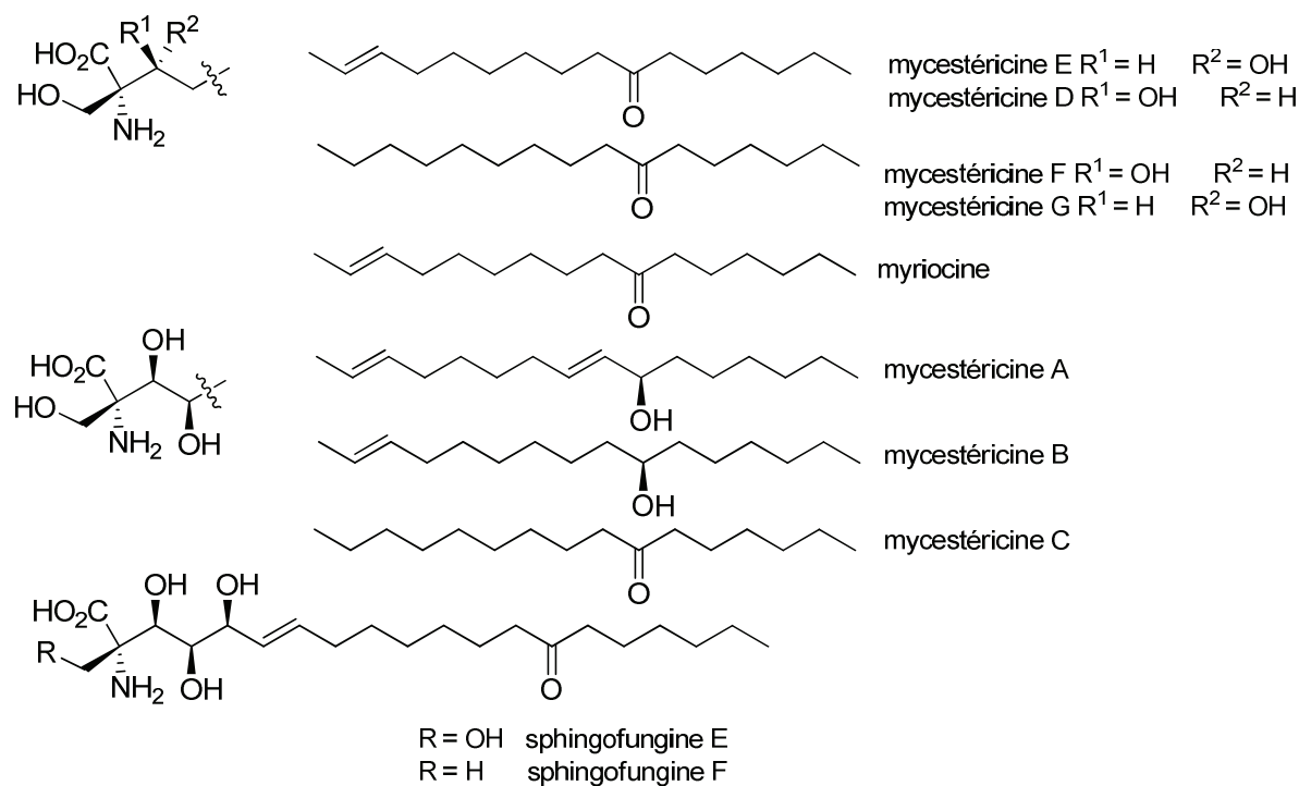
Schéma 5-1 : Acides aminés \alpha -disubstitués présentant une chaîne polyhydroxylée
