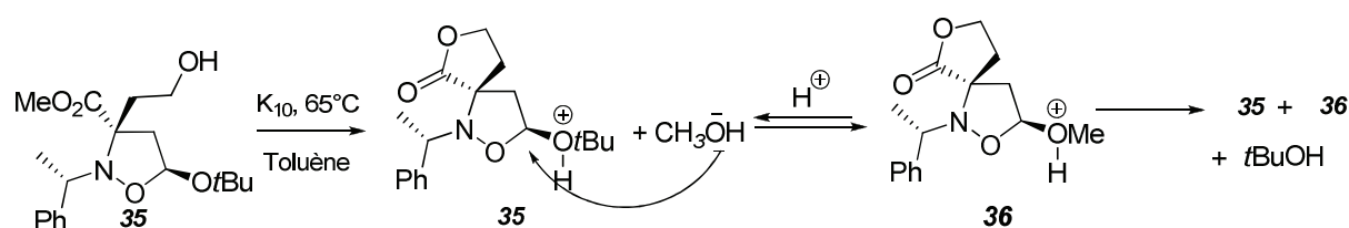
Schéma 3-37 : Mécanisme de formation de 36 à partir de 35 (via l'oxonium)
