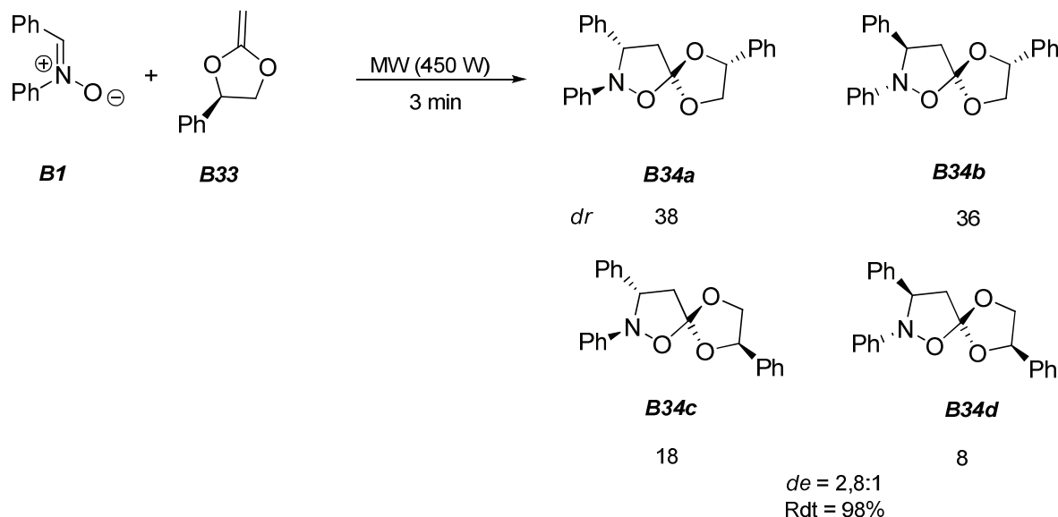
Schéma 2-20 : CD-1,3 entre l'aldonitron C,N diaryls et l'acétal de cétène chiral
