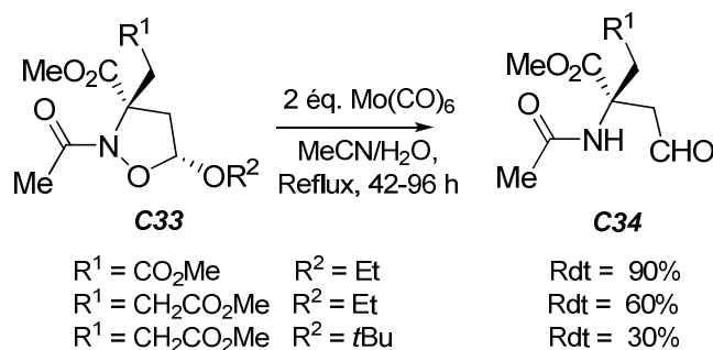
Schéma 3-9 : Synthèse d'alpha-aminoaldéhyde par \text{Mo}(\text{CO})_6
