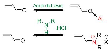
Schéma 2-2 : Mode d'activation du groupement carbonyle
