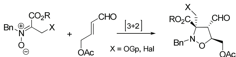
Schéma 5-20 : Synthèse des précurseurs des acides aminés dihydroxylée par la CD-1,3
