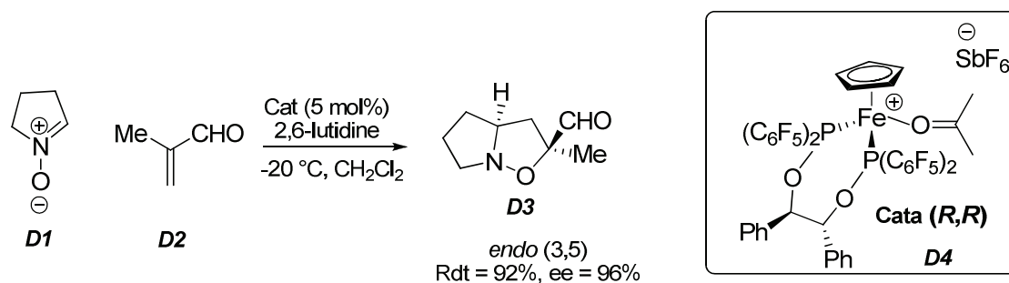
Schéma 4-2 : CD-1,3 entre les nitrones cycliques et la méthacroléine catalysée au fer
