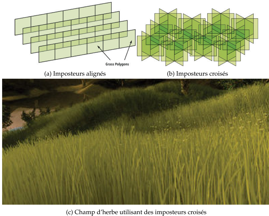
FIGURE 1.5 – Imposteurs géométriques par Pelzer [Pel04]
