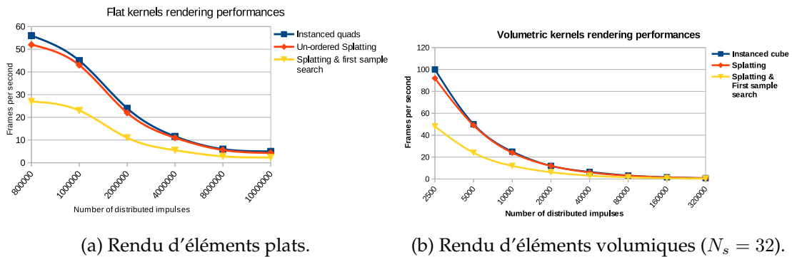
FIGURE 3.10 – Comparatif de performances des méthodes de rendu d'ordre objet sans ordonnancement. Les performances de l'instanciation d'objets et de la projection de noyaux non ordonnés sont similaires mais ces méthodes laissent apparaître de nombreux artéfacts. Au prix d'une division par deux de la vitesse de rendu, notre méthode permet un rendu de bien meilleure qualité.
