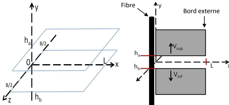
Figure VI-35 : Schématisation des bords de fissures par deux plaques parallèles de surface B*L (extension latérale*profondeur)
