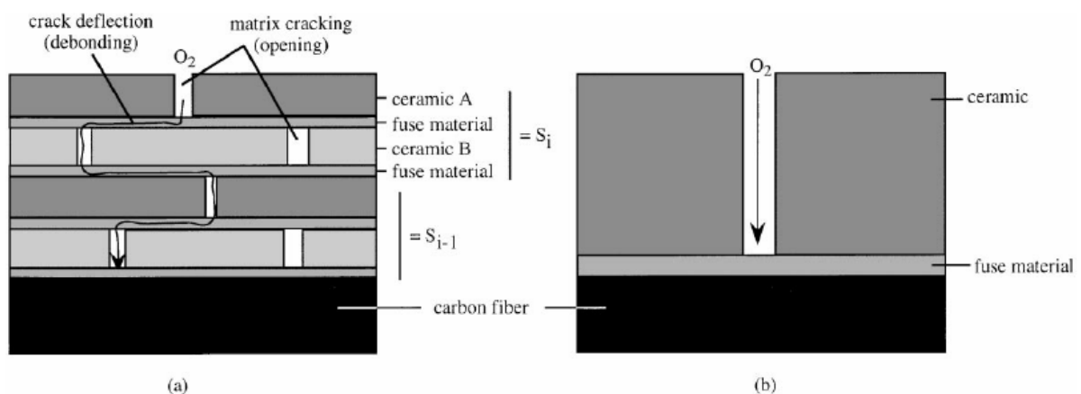
Figure I-1 : Représentation du réseau de fissuration et de la diffusion d'oxygène dans un (a) CMC à matrice multi-séquencee et (b) un CMC à matrice monocouche [Lamouroux-1999]
