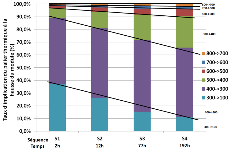
Figure V-7 : Répartition entre chaque palier thermique de son implication dans la hausse du module entre celui à 800°C et celui à 100°C (essai avec plateaux thermiques 156 MPa, 222h, air ambiant, Cerasep®A40C)
