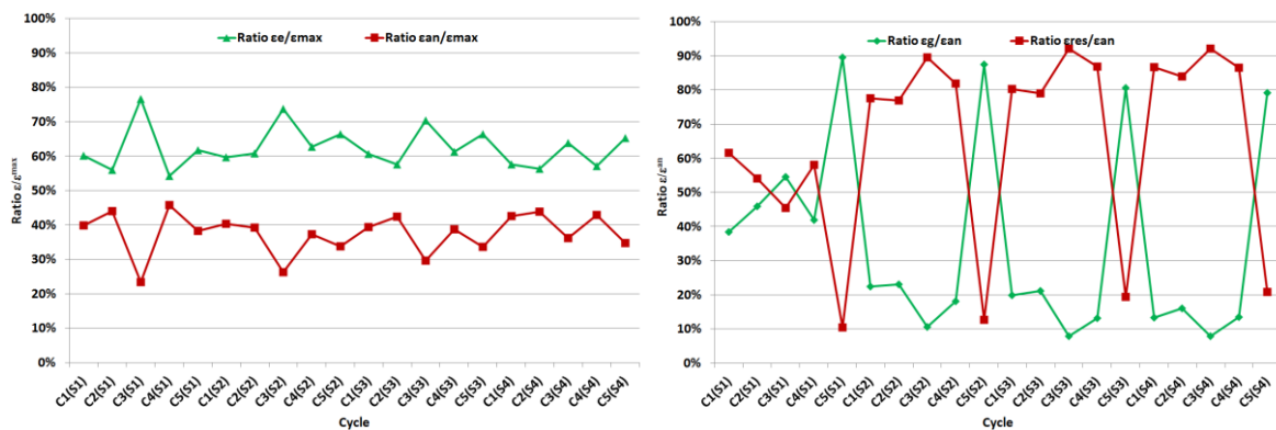
Figure IV-25 : Part de déformation (A) anélastique et élastique au sein des déformations maximales (B) résiduelle et anélastique réversible au sein des déformations anélastiques au cours de l'ensemble des cycles de caractérisations durant l'essai à 800°C et 72 MPa, 225h, sous air ambiant, Cerasep®A40C
