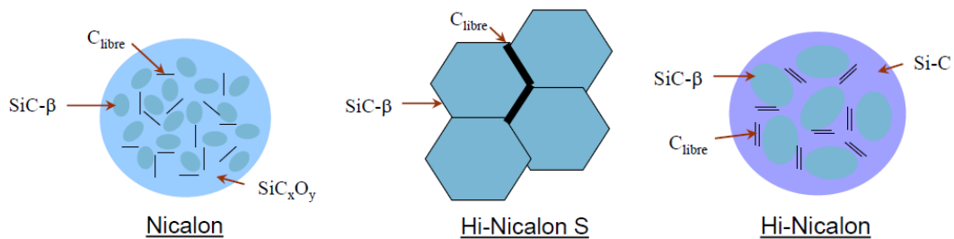
Figure I-7 : Structure des 3 générations de fibre SiC-Nicalon. [Gauthier-2006]
