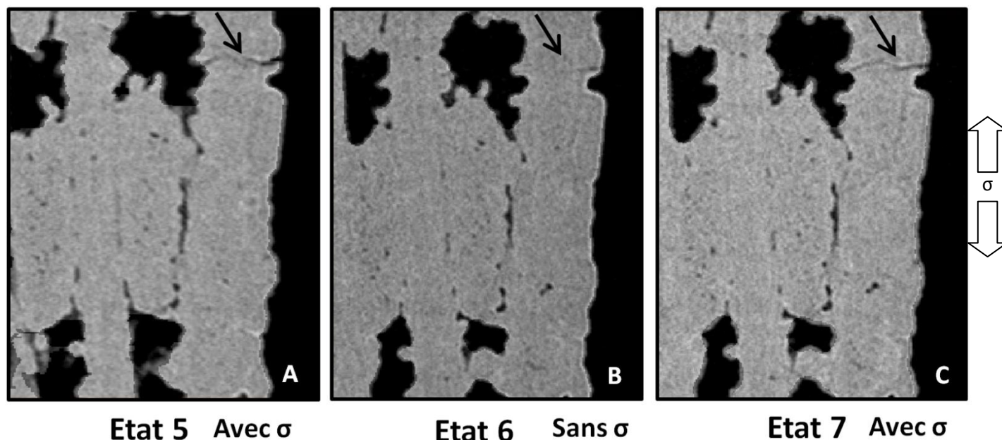
Figure IV-49 : Coupe au sein de la reconstituions du matériau à la suite de la tomographie (A) Etat 5 (B) Etat 6 (C) Etat 7
