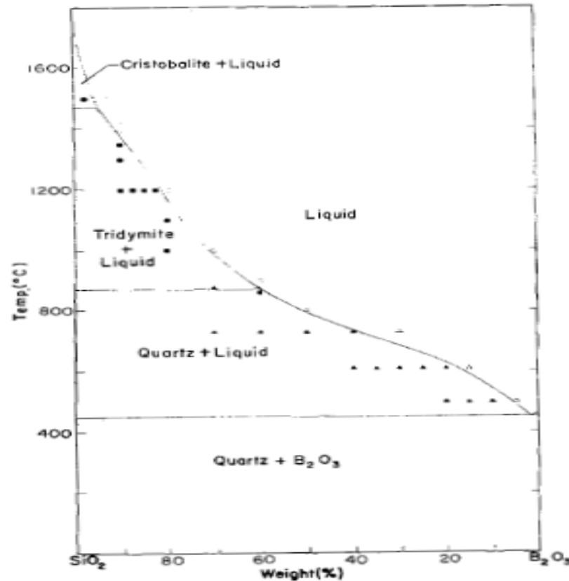
Figure I-5 : Diagramme binaire de SiO_2-B_2O_3 [Rockett-1965]
