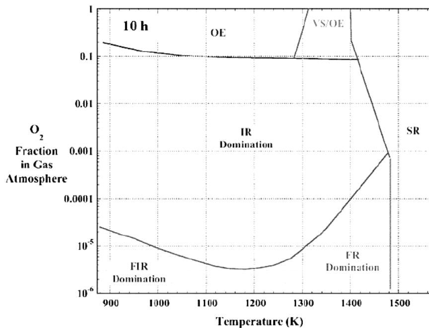
Figure I-31 : Mécanisme de propagation sous critique de fissure au sein d'un SiC/C/SiC en fonction de la température et de la pression partielle en \text{O}_2 (FR : Fiber relaxation by thermal, FIR : Fiber relaxation by irradiation, SR : Fiber stress-rupture, IR : Interface removal by oxidation, OE : Oxidation embrittlement, VS : Viscous sliding) [Jones-2005]
