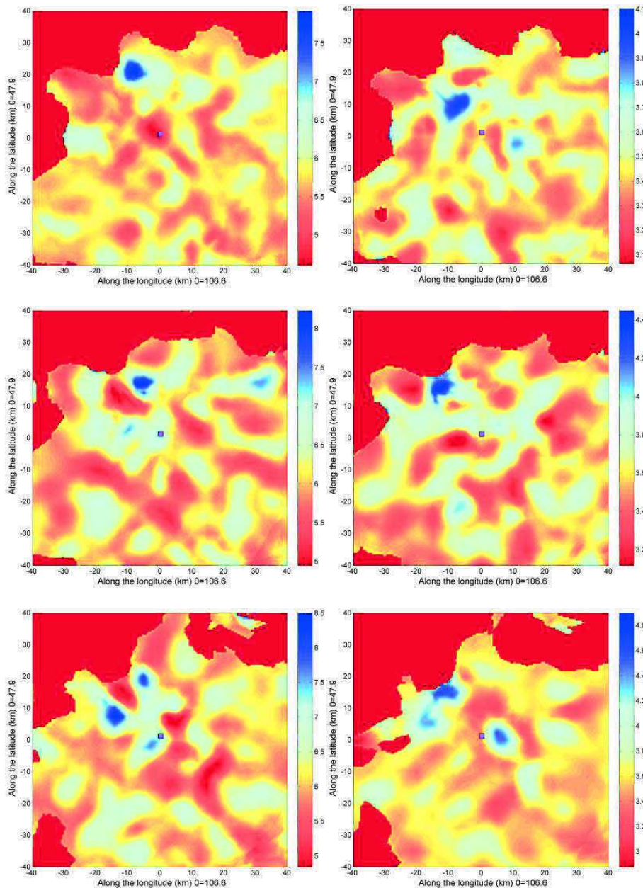
Figure A18: Coupe horizontale du modèle pour le WAM (gauche) et WAMS (droite) à 5, 10 et 15km de profondeur (haut vers le bas). La zone brune au NO marque la région avec un DWS<50. Le carré violet correspond à la position de la tranchée d'Emeelt.
