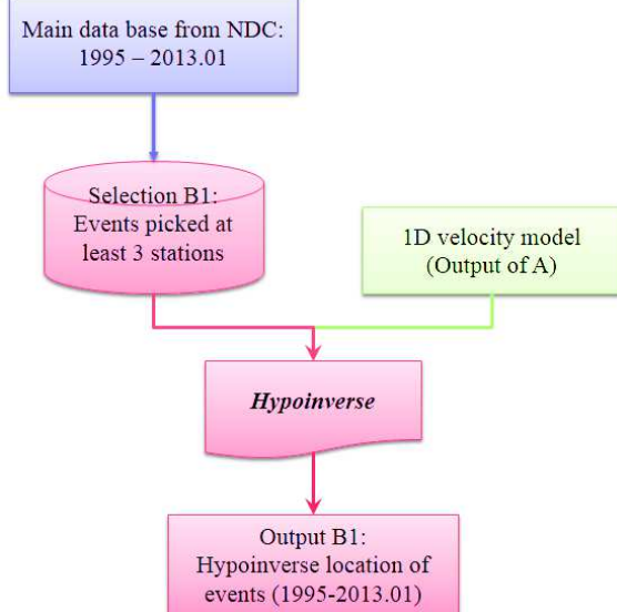
Figure A14: Résumé de la procédure "Hypoinverse" appliquée (Procédure B1).
