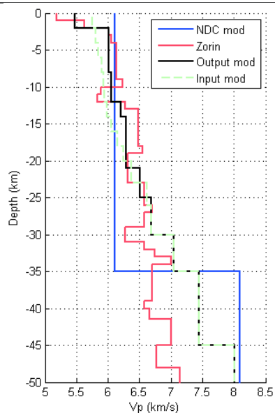
Figure A13: Nouveau modèle de vitesse 1D (Output) comparé à des modèles soit publiés (Zorin et al., 2002) soit utilisés au NDC
