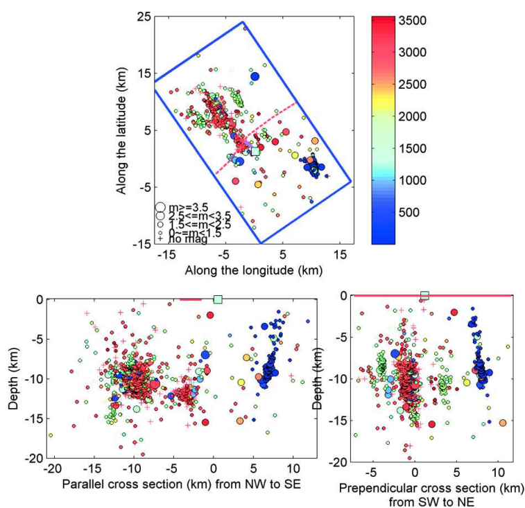
Figure A27: Localisation finale des séismes de la zone d'Emeelt via TomoDD. L'échelle de couleurs indique le nombre de jours depuis le 2005.01.01. En violet= zone des rupture de surface identifiées, carré bleu = tranchée, rouge = position de la faille Mésozoïque en surface.
