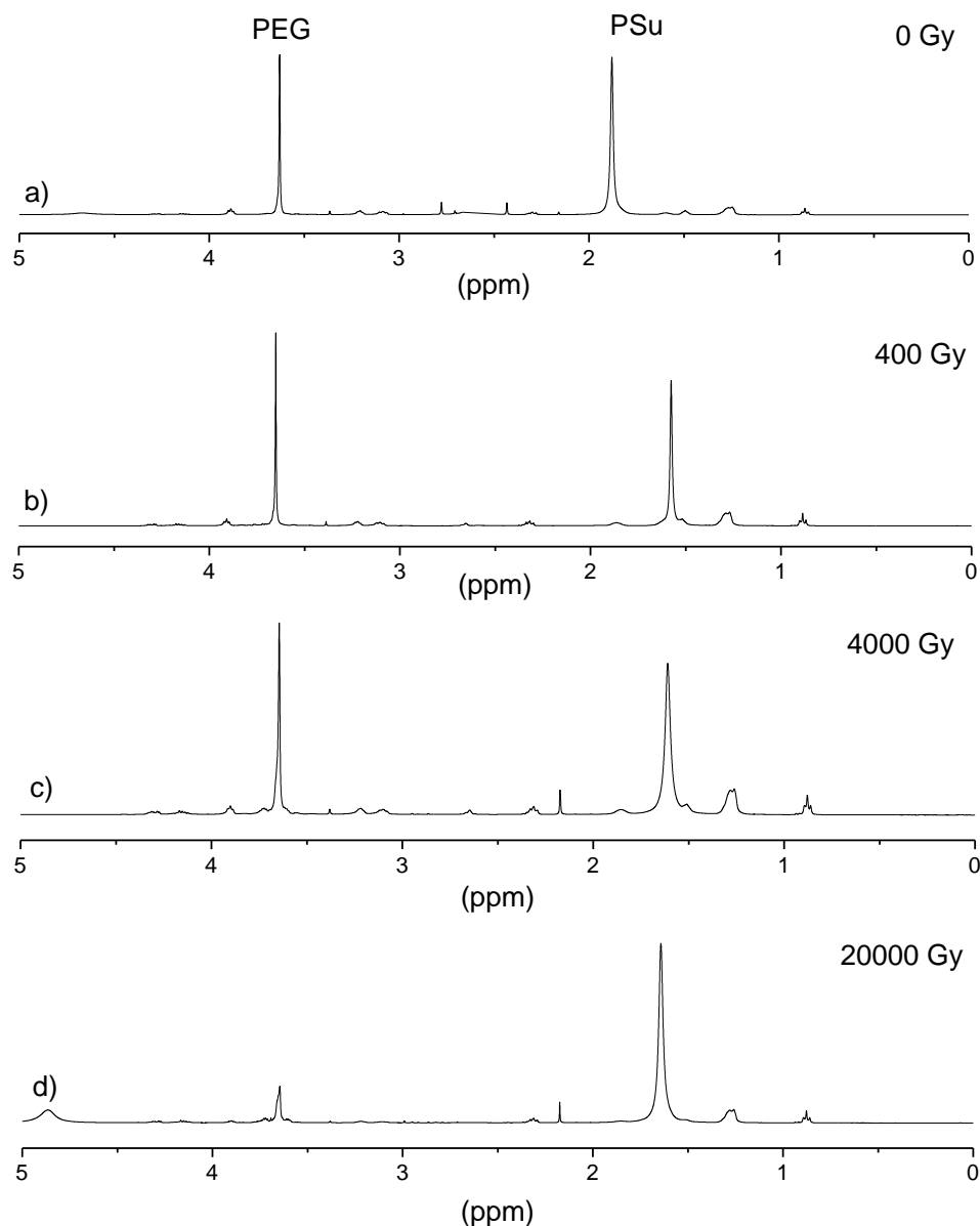
Figure III.18 : Spectres RMN ^1\text{H} dans le \text{CDCl}_3 des copolymères PEG- b -PSu après irradiation en milieu oxygéné
