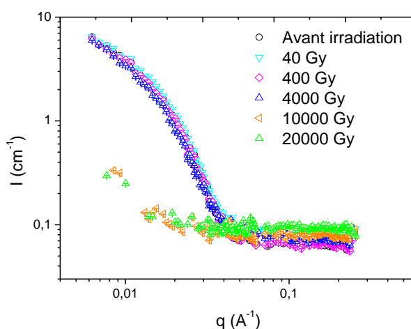
Figure III.7 : Spectres DNPA des micelles PEG- b -PMA t Bu après irradiation en milieu oxygéné
