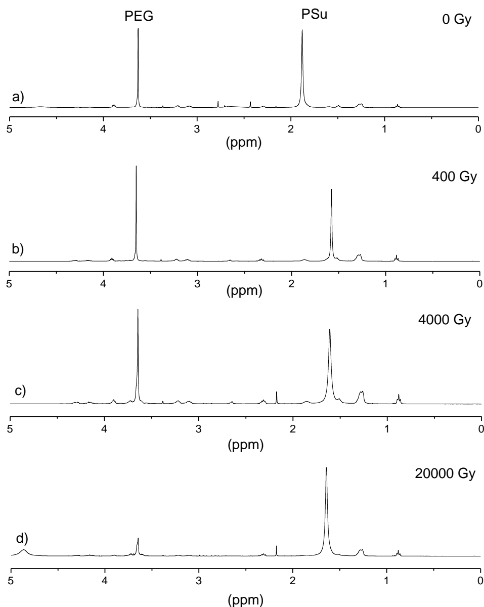
Figure III.18 : Spectres RMN 1 H dans le CDCl 3 des copolymères PEG- b -PSu après irradiation en milieu oxygéné
