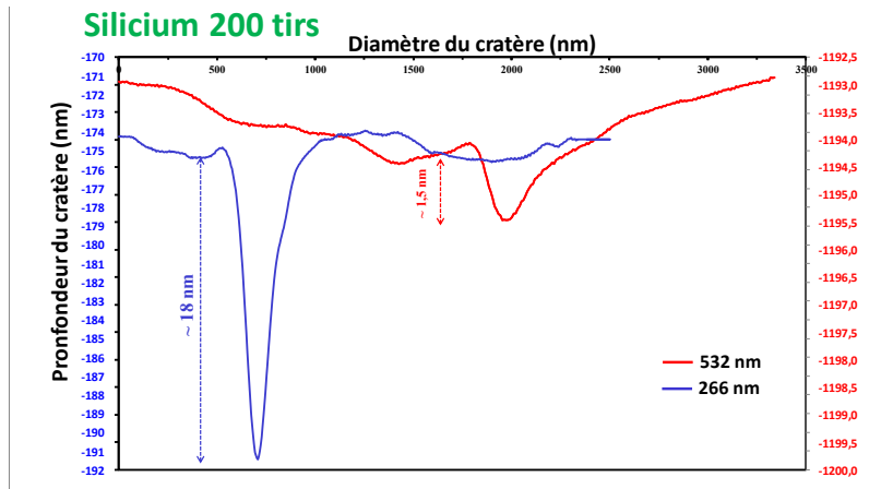
Figure IV-27 : Cratères obtenus sur un échantillon de silicium après 200 tirs laser pour les deux longueurs d'onde 266 et 532 nm.
