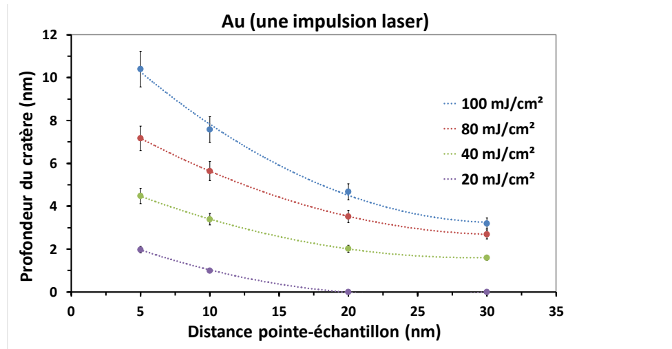
Figure IV-6 : Variation de la profondeur du cratère sur un échantillon d'or en fonction de la distance pointe-échantillon et pour différentes fluences laser. L'incertitude sur la mesure à un niveau de confiance de 95% est de 8% pour 6 mesures différentes.
