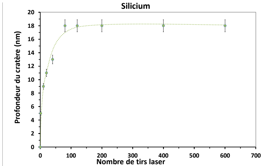
Figure IV-11 : Variation de la profondeur des cratères sur un échantillon de silicium en fonction du nombre de tirs lasers (distance pointe-échantillon 5 nm, fluence 80 mJ/cm 2 ). L'incertitude sur la mesure à un niveau de confiance de 95% est de 5% pour 4 mesures différentes.
