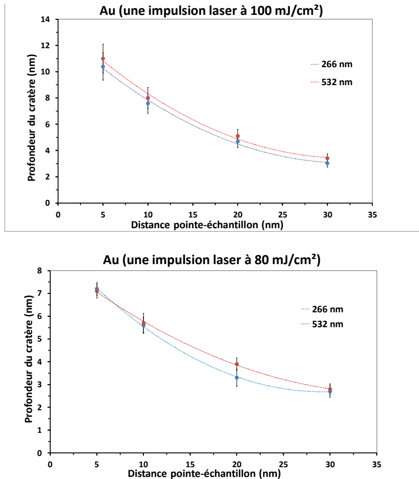
Figure IV-20 : Comparaison de la profondeur du cratère obtenu sur un échantillon d'or en fonction de la distance pointe-échantillon et de la longueur d'onde du laser : a) fluence laser 100 mJ/cm 2 b) fluence laser 80 mJ/cm 2 . L'incertitude sur la mesure à un niveau de confiance de 95 % est de 8 % pour 6 mesures différentes.
