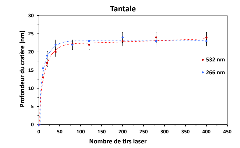
Figure IV-23 : Comparaison de la profondeur des cratères obtenus sur un échantillon de tantale en fonction du nombre de tirs laser et pour deux longueurs d'onde (distance pointe-échantillon 5 nm,
