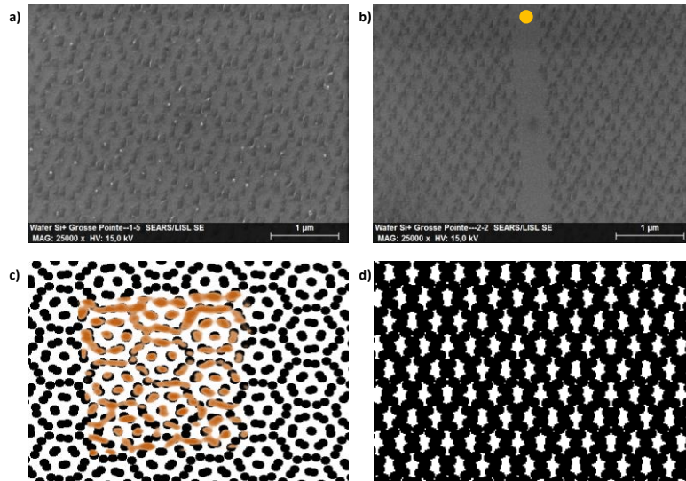
Figure IV-3 : Répartition des cratères sur la surface du silicium; F_{laser} = 5 Hz et vitesse de balayage 2 ln/s : a) distribution expérimentale, c) distribution théorique F_{laser} = 10 Hz et vitesse de balayage 2 ln/s : b) distribution expérimentale, d) distribution théorique
