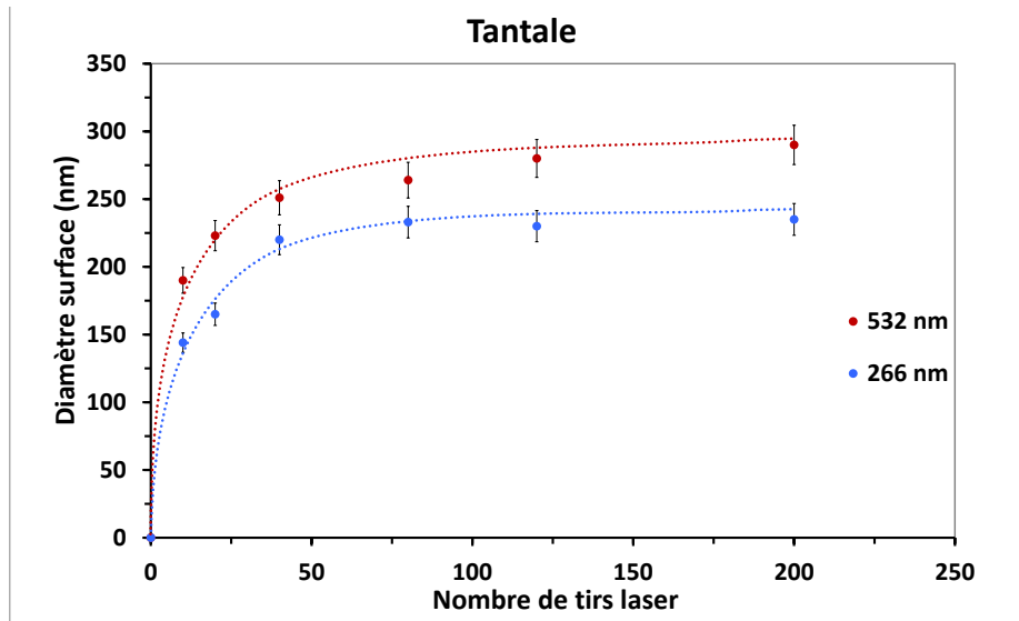
Figure IV-24 : Comparaison du diamètre en surface des cratères obtenus sur un échantillon de tantale en fonction du nombre de tirs laser et pour deux longueurs d'onde (distance pointe-échantillon 5 nm, fluence 80 \text{ mJ/cm}^2 ). L'incertitude sur la mesure à un niveau de confiance de 95 % est de 5 % pour 4 mesures différentes.
