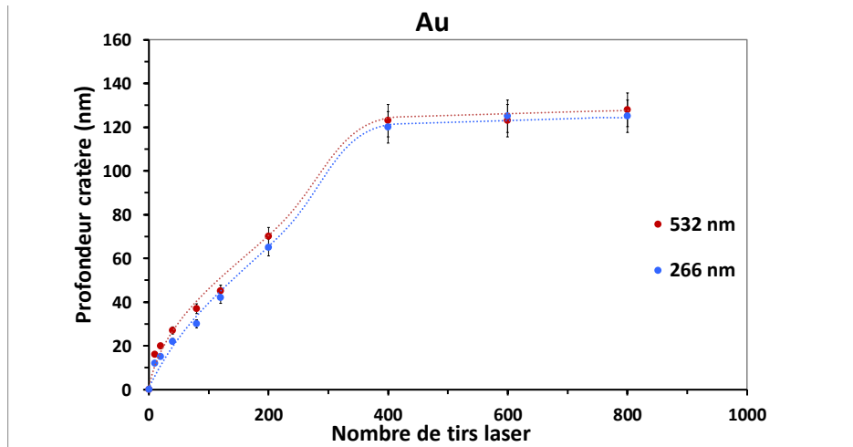
Figure IV-21 : Comparaison de la profondeur des cratères obtenus sur un échantillon d'or en fonction du nombre de tirs laser et pour deux longueurs d'onde (distance pointe-échantillon 5 nm, fluence 80 mJ/cm 2 ). L'incertitude sur la mesure à un niveau de confiance de 95% est de 5% pour 4 mesures différentes.
