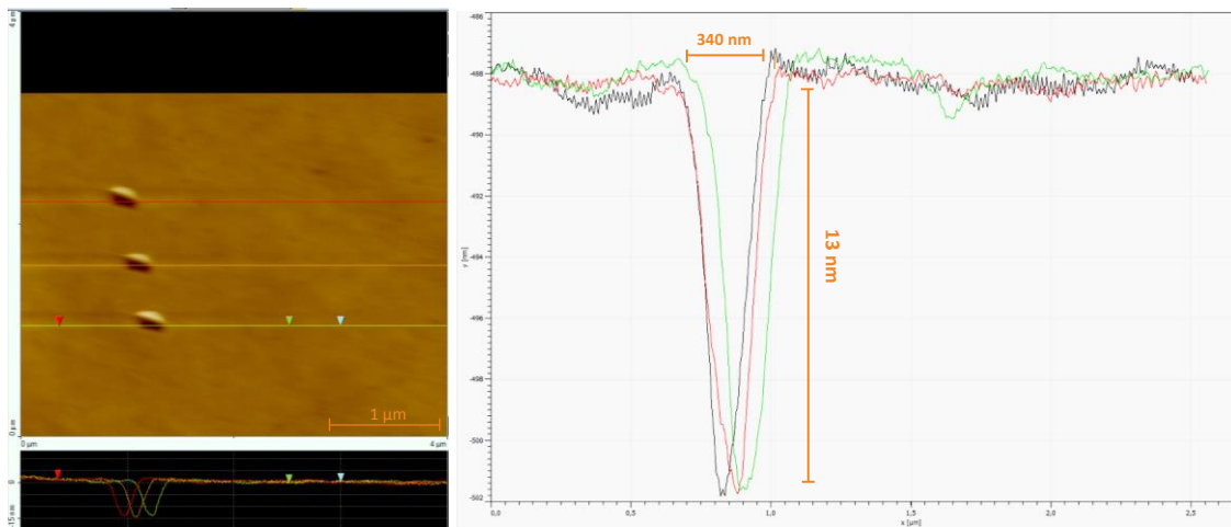
Figure IV-13 : Exploitation des cratères pour 40 tirs laser sur un échantillon de silicium par le logiciel Gwyddion
