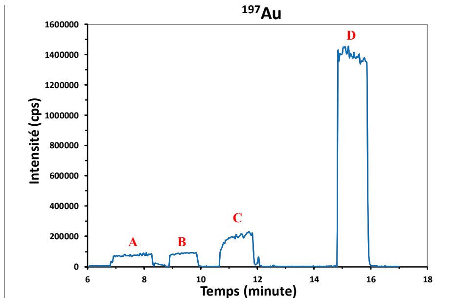
Figure V-4 : Intensité du signal d'or en l'ICPMS
