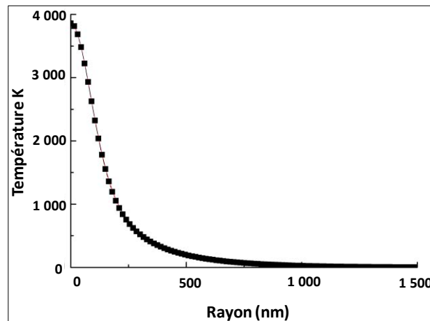
Figure IV-17 : Distribution de la température de chauffage induite par le champ proche. La pointe est en silicium revêtue de diamant, rayon de courbure 100 nm, échantillon d'or.
