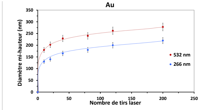
Figure IV-22 : Comparaison du diamètre à mi-hauteur des cratères obtenus sur un échantillon d'or en fonction du nombre de tirs laser et pour deux longueurs d'onde (distance pointe-échantillon 5 nm, fluence 80 mJ/cm 2 ). L'incertitude sur la mesure à un niveau de confiance de 95% est de 5% pour 4 mesures différentes.
