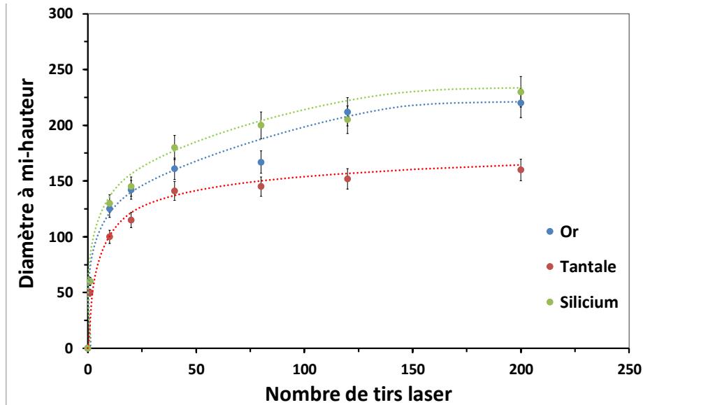
Figure IV-16 : Variation du diamètre à mi-hauteur des cratères sur des échantillons d'or, de tantale et de silicium en fonction de nombre de tirs lasers (distance pointe-échantillon 5 nm, fluence 80 mJ/cm 2 ). L'incertitude sur la mesure à un niveau de confiance de 95% est de 5% pour 4 mesures différentes.
