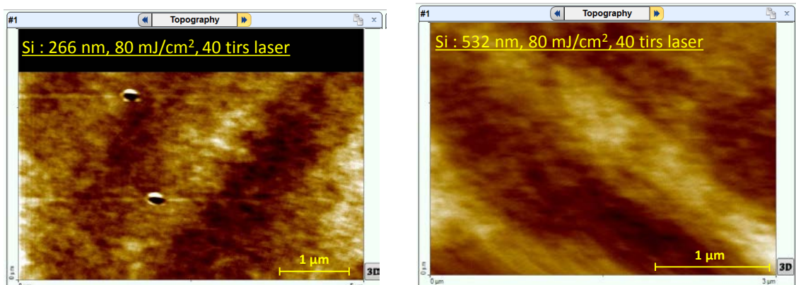
Figure IV-26 : Comparaison des cratères à 40 tirs cumulés sur un échantillon de silicium pour deux longueurs d'onde différentes 266 et 532 nm (distance pointe-échantillon 5 nm).
