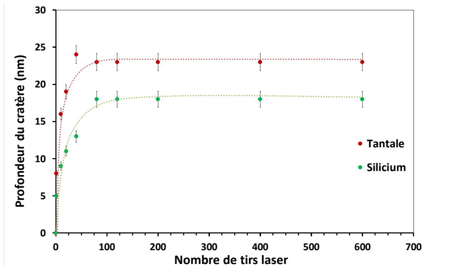
Figure IV-14 : Variation de la profondeur des cratères sur des échantillons de tantale et de silicium en fonction de nombre de tirs lasers (distance pointe-échantillon 5 nm, fluence 80 mJ/cm 2 ). L'incertitude sur la mesure à un niveau de confiance de 95 % est de 4 % pour 4 mesures différentes.
