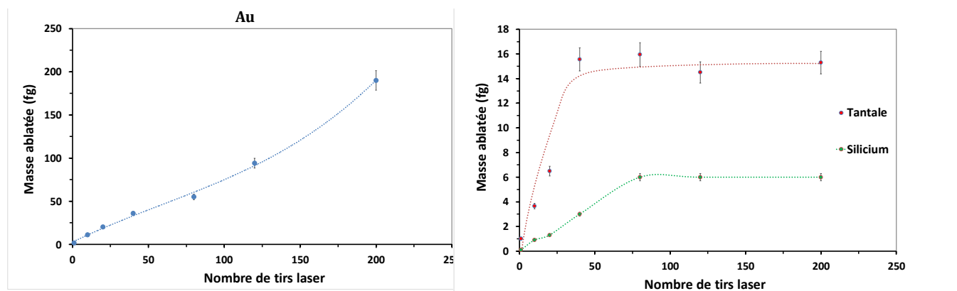
Figure IV-19 : Variation de la masse ablatée (fg) en fonction de nombre de tirs appliqués sur l'or, le tantale et le silicium (distance pointe-échantillon 5 nm, fluence 80 mJ/cm 2 ). L'incertitude sur la mesure à un niveau de confiance de 95 % est de 8 % pour 4 mesures différentes.
