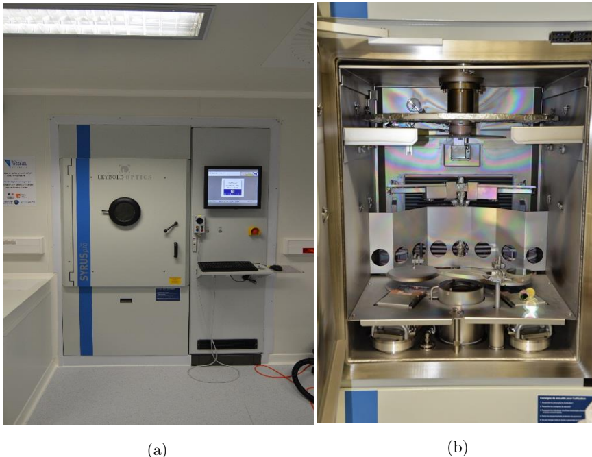
Figure 2-1 : Leybold Optics SYRUSpro 710 en environnement salle blanche (Espace Photonique) : (a) l'interface du bâti, (b) son intérieur (canons à électrons et assistance plasma, porte-substrats...)
