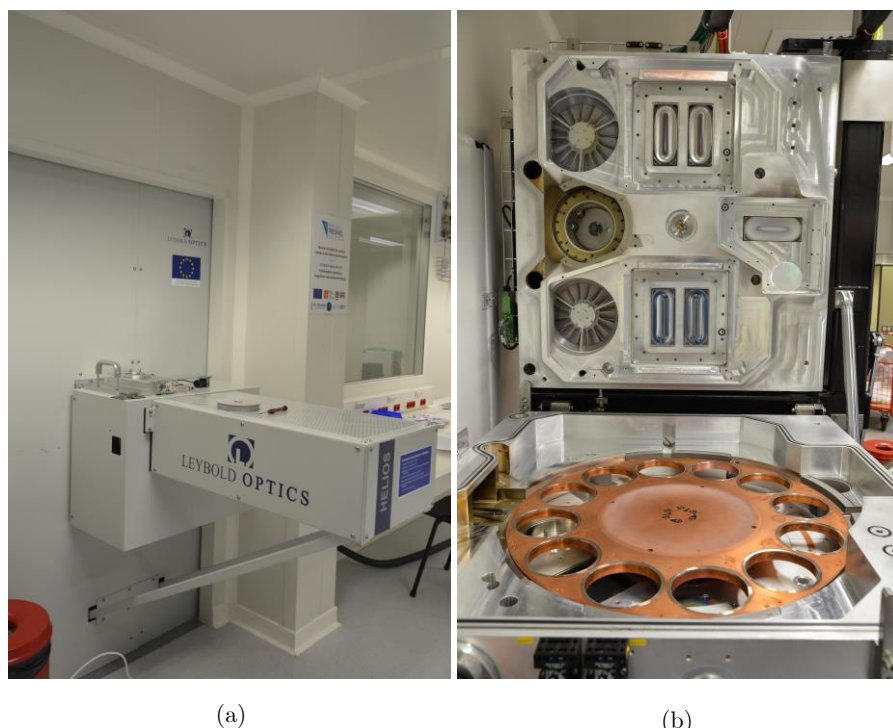
Figure 2-2 : Leybold Optics HELIOS : (a) sas de chargement en salle blanche, (b) intérieur du bâti dans le doigt gris (magnétrons, source plasma, plateau porte substrats...)
