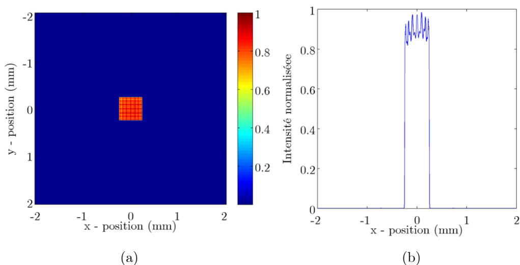
Figure 5-9 : Simulation de la distribution d'intensité dans le plan focale d'une lentille après mise en forme de faisceau avec l'élément décrit par la carte des phases de la Figure 5-8: (a) profil d'intensité 2D et (b) profil d'intensité 1D en y=0
