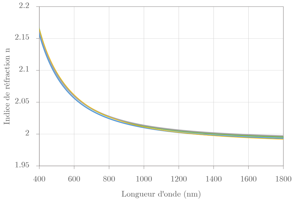
Figure 3-9 : Dépendance spectrale (dispersion) de l'indice de réfraction du Ta_2O_5 mesurée sur un ensemble de quatre échantillons de \sim 150 nm d'épaisseur
