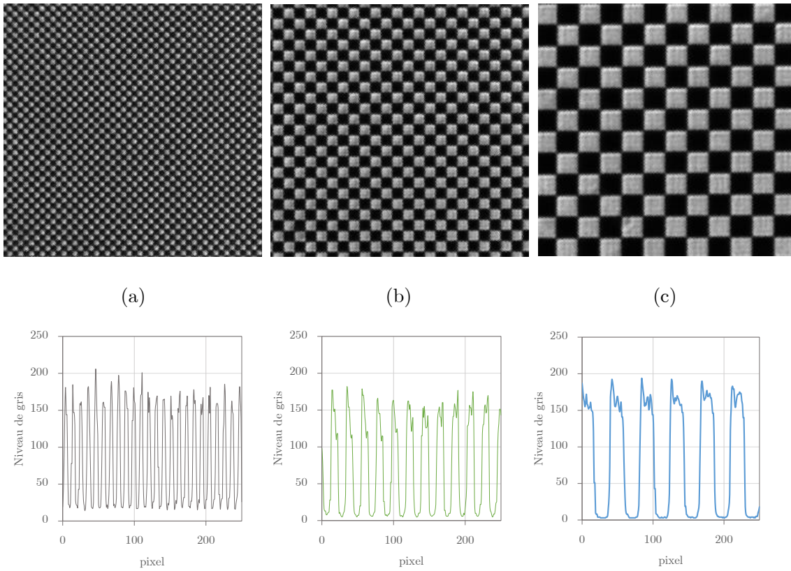
Figure 5-13 : Image et profil d'intensité des différents damiers générés par la matrice de micro-miroirs dans le plan focal du montage 4-f : (a) damier 2 \times 2 pixels, (b) damier 4 \times 4 pixels, et (c) damier 8 \times 8 pixels
