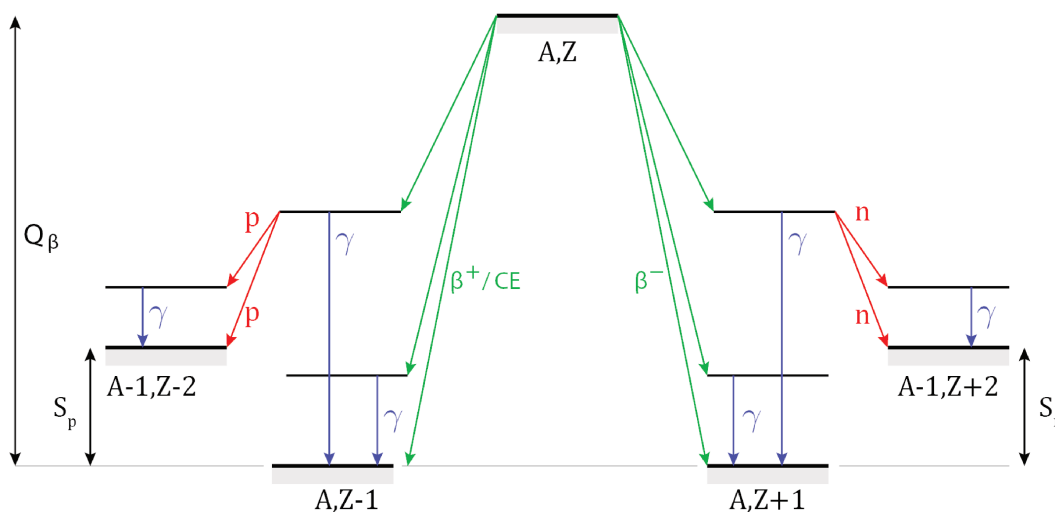
FIGURE 2.2 – Schéma des décroissances \beta ( \beta^+ , CE et \beta^- ) suivies de décroissances \gamma et/ou émission neutron/proton retardée.
