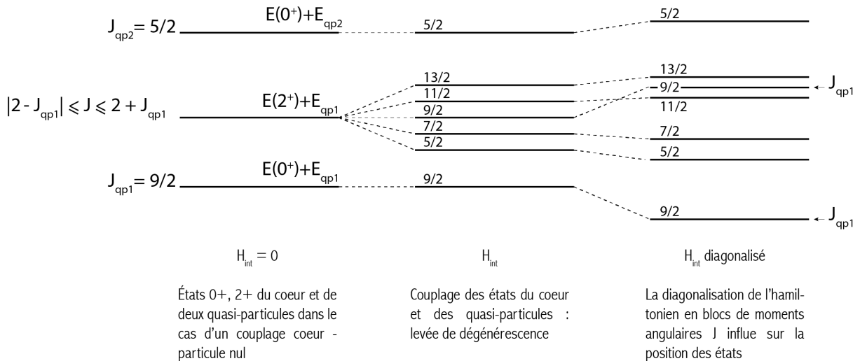
FIGURE 6.2 – Levée de dégénérescence lors du couplage cœur - particule.
