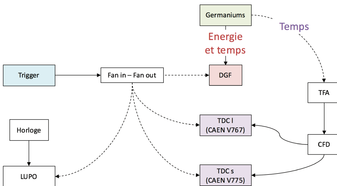
FIGURE 4.5 – Électronique de l'acquisition de EURICA.
