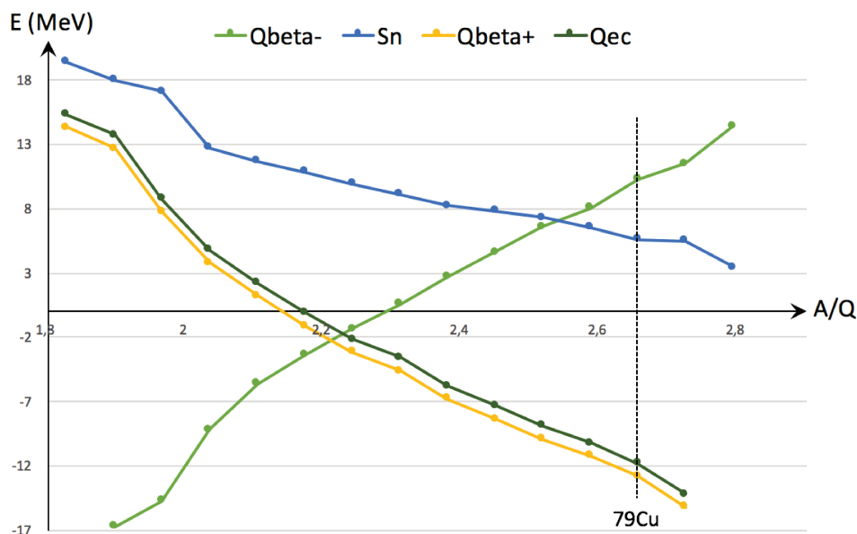
FIGURE 2.1 – Systématique des énergies Q_{\beta^-} (énergie disponible lors de la décroissance \beta^- ), S_n (énergie de séparation d'un neutron), Q_{\beta^+} (énergie disponible lors de la décroissance \beta^+ ) et Q_{EC} (énergie disponible lors de la capture électronique) pour les isotopes pair-impairs du cuivre.
