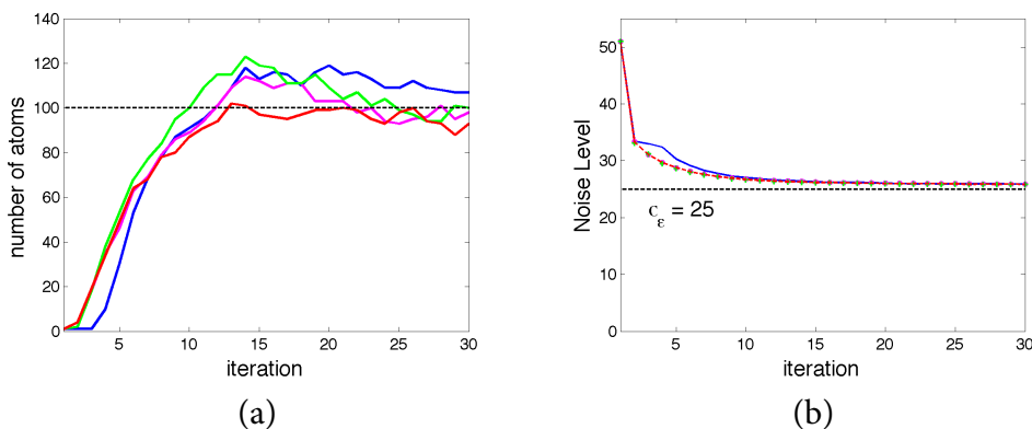
FIGURE 8.7 – (a) Evolution du nombre d'atomes de dictionnaire au cours des itérations de IBP-DL sur Barbara pour 4 différentes réalisations avec \sigma_\epsilon = 25 . (b) Evolution du niveau de bruit échantillonné par IBP-DL au cours des itérations sur Barbara quand \sigma_\epsilon = 25 and \sigma_{init} = 51 .
