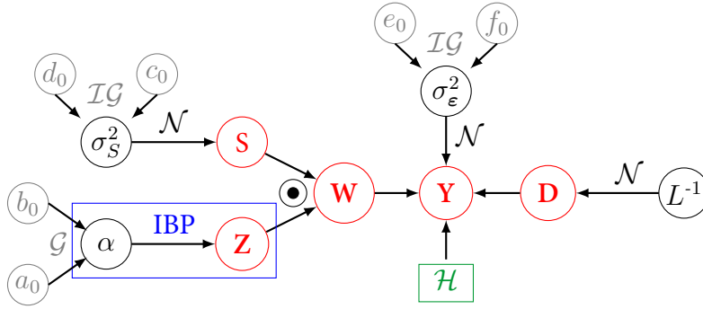
FIGURE 7.1 – IBP-DL pour les problèmes inverses linéaires avec un bruit gaussien.
