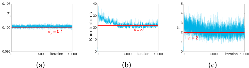
FIGURE 8.3 – Evolution des paramètres échantillonnés à travers les itérations de IBP-DL : (a) le niveau de bruit \sigma_\epsilon , (b) le nombre K d’atomes, (c) le paramètre \alpha de la loi a priori IBP.
