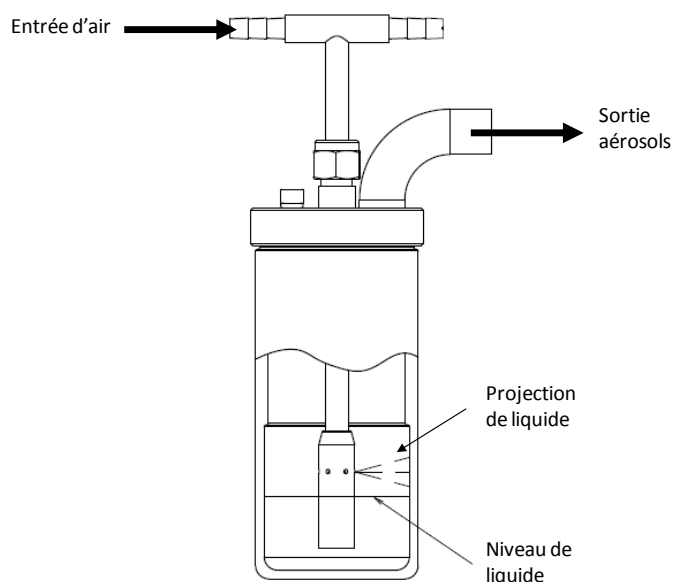
Figure 21 Schéma du nébuliseur Collison
