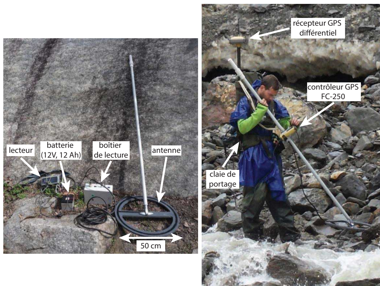
FIGURE 4.9 – Appareillage mobile pour le suivi des galets marqués par PIT.
