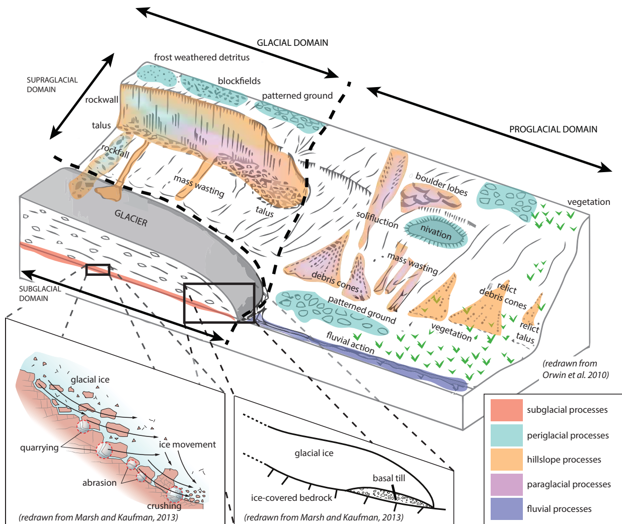
FIGURE 6 – Processus d'érosion dans un bassin versant partiellement englacé. Cette figure est assemblée à partir des figures proposées par Orwin et al. (2010) et Marsh and Kaufman (2013).
