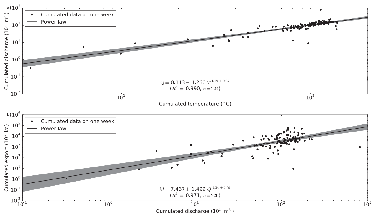
FIGURE 5.11 – Relation entre température, volume d’eau écoulé et export sédimentaire. a) Relation entre température, T , et volume d’eau de fonte, Q , cumulés sur une semaine ; b) relation entre volume d’eau de fonte écoulé, Q , et export sédimentaire cumulé sur une semaine, M . a-b) La zone grisée représente les limites de l’intervalle de confiance à 99%. Les lois puissances sont statistiquement significatives. Toutefois la relation entre débit de fonte et export sédimentaire (b) montre une dispersion sur trois ordres de grandeur pour les débits hebdomadaires cumulés de la saison de fonte.
