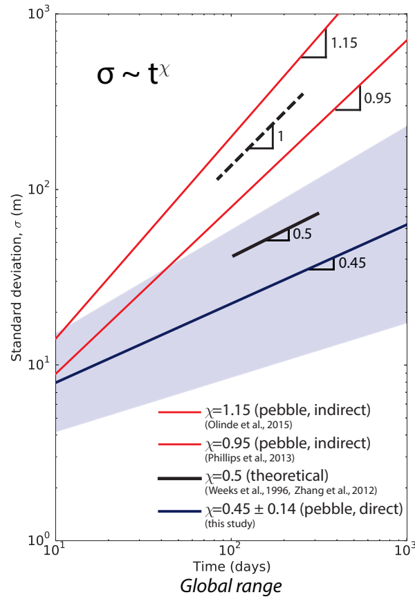
FIGURE 4.35 – Mode de diffusion de la charge de fond à long terme. L’estimation apportée par cette étude est représentée en bleu avec son intervalle de confiance à une déviation standard. Les estimations de Olinde and Johnson (2015) et Phillips et al. (2013) sont indiquées en rouge. L’évolution théorique de Weeks et al. (1996) et Zhang et al. (2012) est représentée en noir.
