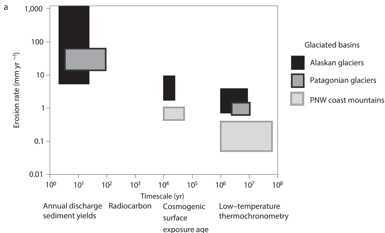
FIGURE 2 – Variation de l'ordre de grandeur de l'érosion glaciaire en fonction de l'intervalle de mesure considéré et de la situation géographique (Koppes and Montgomery, 2009). PNW : Pacific North West
