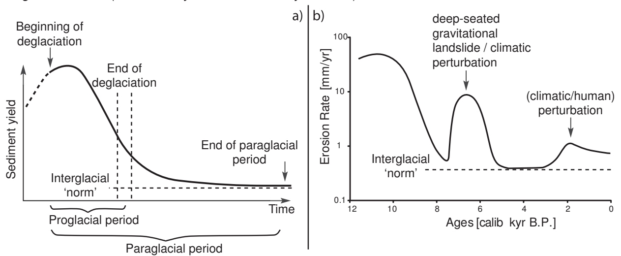
FIGURE 3 – Modèles conceptuels du cycle paraglaciaire. a) cycle paraglaciaire conceptuel de Church and Ryder (1972); b) Les observations acquises dans le bassin versant du Zielbach (Suisse) impliquent d'amender ce modèle pour inclure les perturbations liées aux événements de forte amplitude et à l'activité anthropique (à droite, modifiée d'après Savi et al., 2014b).
