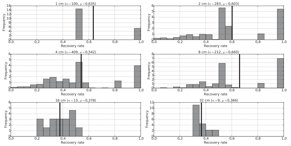
FIGURE 4.19 – Distribution des taux de récupération en fonction de la taille granulométrique des galets. Pour chaque classe granulométrique, la distribution des taux de récupération pour toutes les campagnes est représentée ainsi que la moyenne (ligne verticale noire). \mu : valeur moyenne ; n : nombre de galets dans la classe granulométrique considérée.
