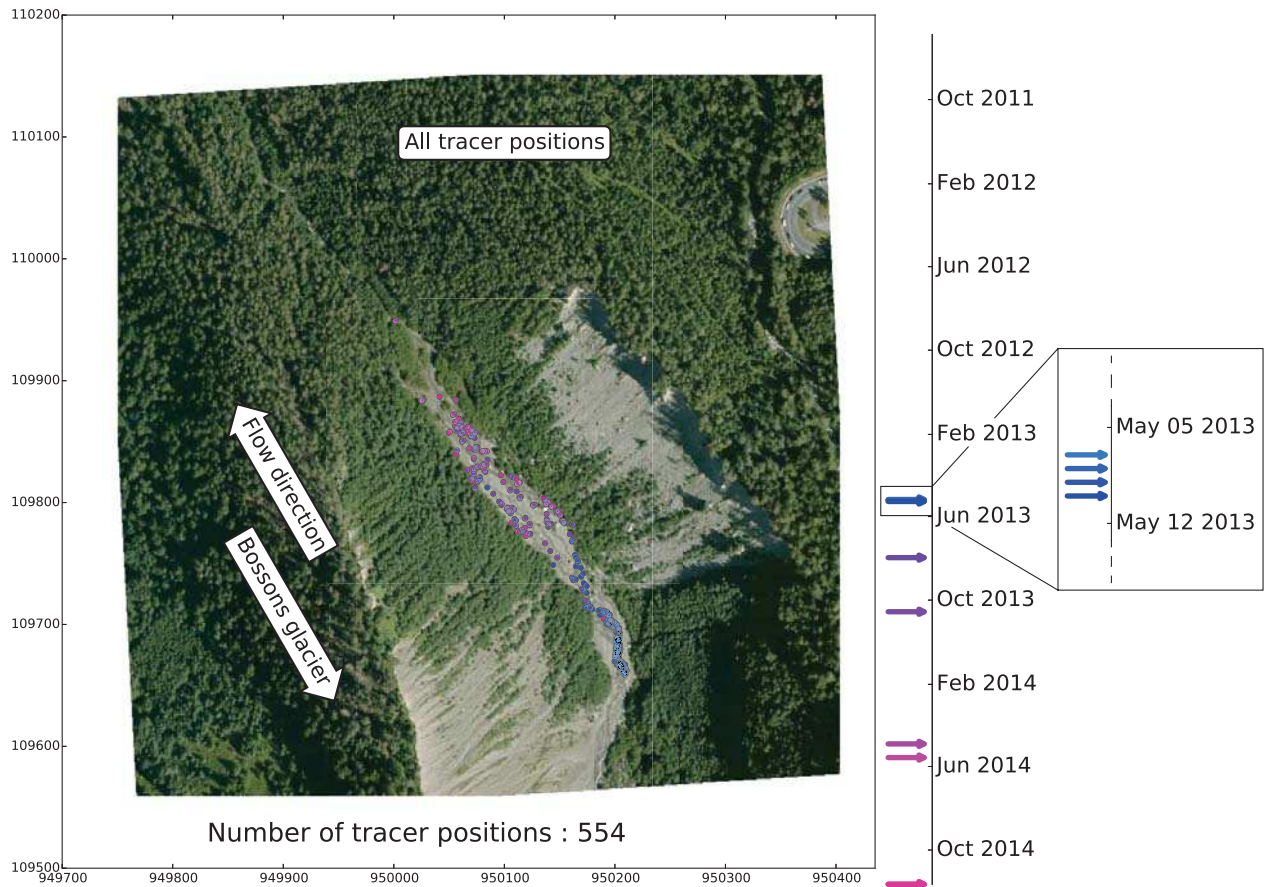
FIGURE 4.18 – Carte de l'évolution de la position des traceurs de l'expérience AA/AB lors de 6 campagnes de mesures successives. Seules les campagnes avec plus de 20 positions sont représentées. Les positions de ces campagnes sont décrites statistiquement sur la Fig. 4.33c. Coordonnées en Lambert II.
