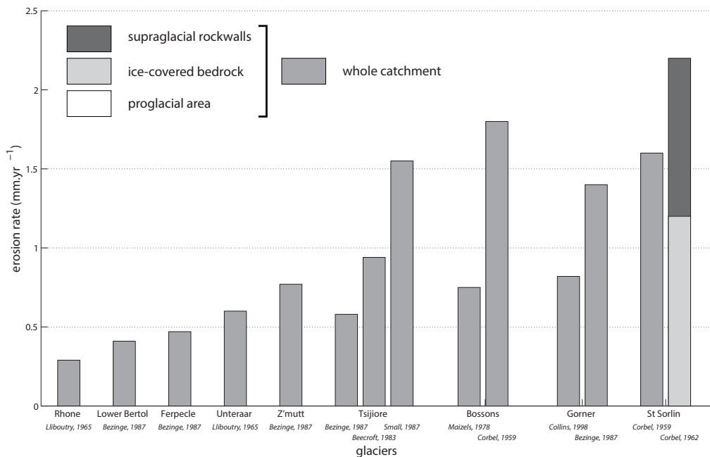
FIGURE 8 – Taux d'érosion de bassins versants englacés alpins. Le glacier des Bossons sur lequel porte cette thèse apparaît ici avoir une valeur moyenne par rapport aux autres glaciers alpins.
