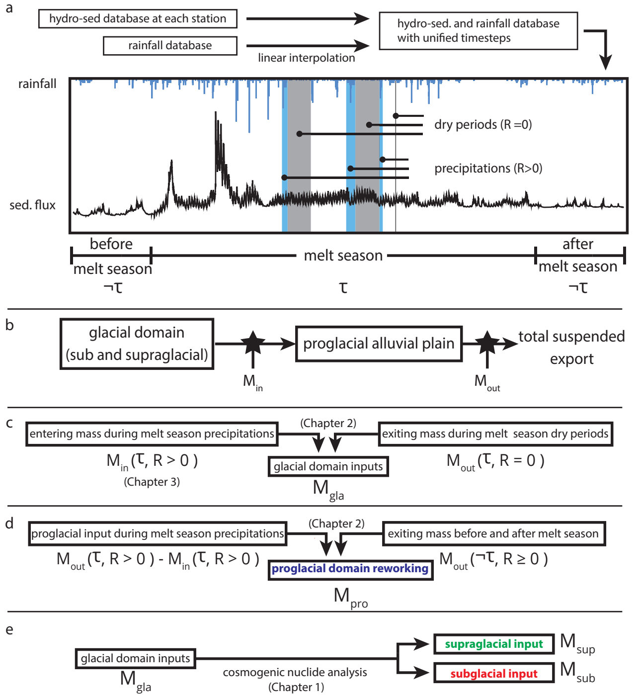
FIGURE 5.6 – Estimation des apports sédimentaires par domaine géomorphologique dans le bassin du glacier des Bossons. a) Établissement d'une base de données avec pas de temps unifié; b) Schéma conceptuel présentant les masses entrante, M_{in} et sortante, M_{out} de la plaine alluviale; c) Estimation de l'apport du domaine glaciaire, M_{gla} (Eq. 5.5); d) Estimation de l'apport du domaine proglaciaire, M_{pro} (Eq. 5.6); e) Estimation des apports des domaines supraglaciaire, M_{sup} (Eq. 5.7), et sous-glaciaire M_{sub} (Eq. 5.8).
