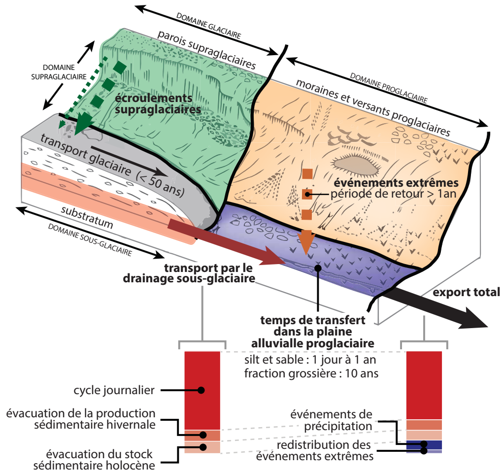
FIGURE 2 – Transfert de sédiments et stockage intermédiaire dans le bassin versant du glacier des Bossons (Mont-Blanc, France).
