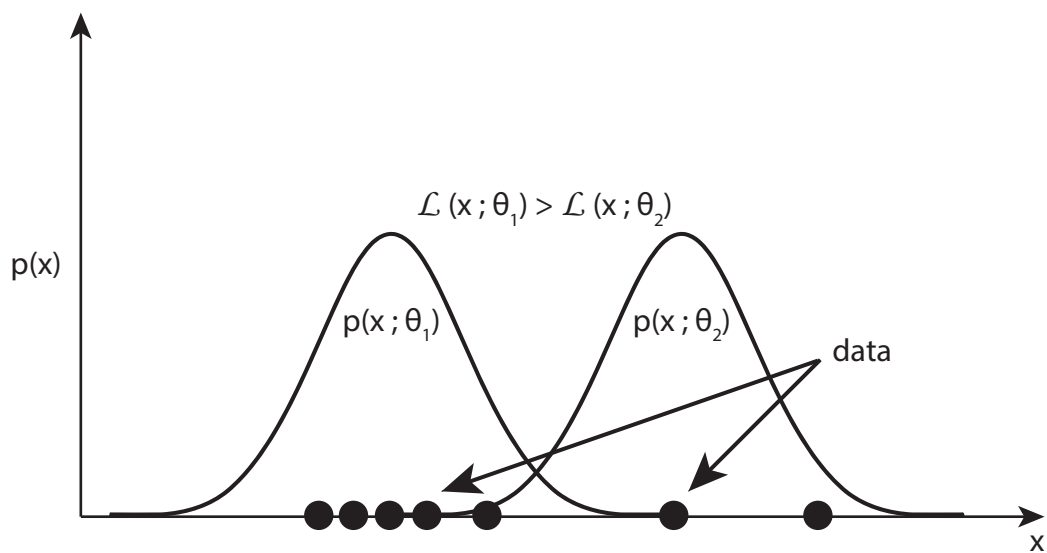
FIGURE C.3 – Méthode du maximum de vraisemblance (MLE).
