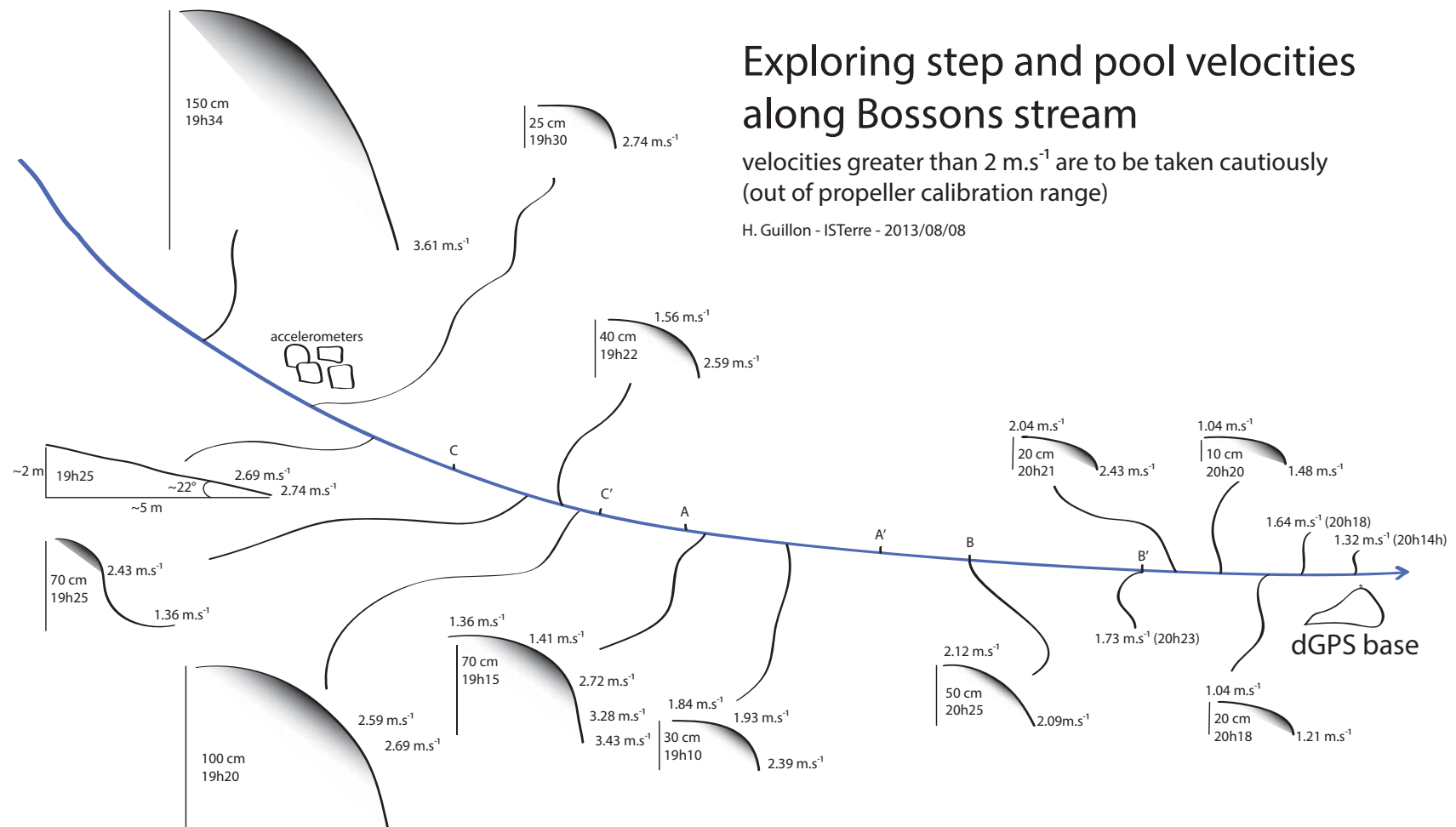
FIGURE D.1 – Vitesse d'écoulement du torrent des Bossons effectuée au moulinet en juillet 2013.
