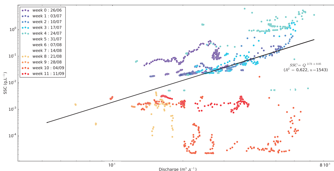
Figure 3.1 – Relation entre la concentration à la station BUS et le débit à la station BDS durant les précipitations de la saison de fonte 2013. Les données sont regroupées par semaine du début (violet) à la fin de la saison de fonte (rouge). La dispersion des données est importante et un débit donné engendre une réponse variant sur plusieurs ordres de grandeur.
