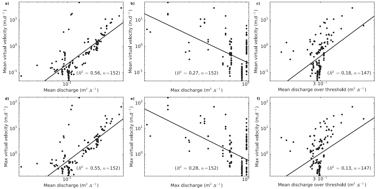
FIGURE 4.30 – Relation entre variables hydro-dynamiques et transport des traceurs. Vitesse virtuelle moyenne en fonction : a) du débit moyen; b) du débit maximal; c) du débit moyen supérieur à la limite d'initiation du transport ( 0.2 \text{ m}^3 \cdot \text{s}^{-1} ); vitesse virtuelle maximale en fonction : d) du débit moyen; e) du débit maximal; f) du débit moyen supérieur à la limite d'initiation du transport ( 0.2 \text{ m}^3 \cdot \text{s}^{-1} ).
