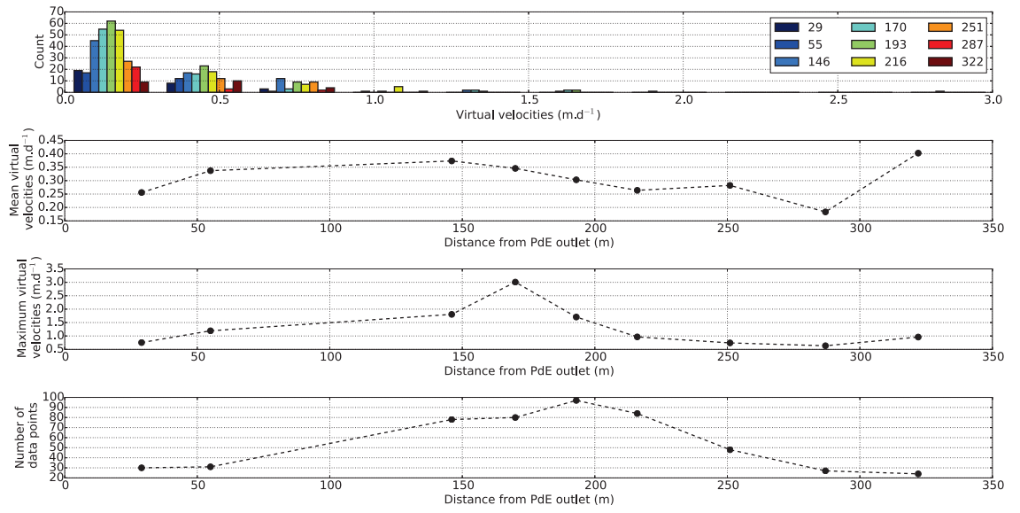
FIGURE 4.24 – Résultats du lâcher E. a) Distribution des vitesses virtuelles pour chaque profil situé de 29 à 322 m de la sortie du Plan des Eaux. b) Vitesse virtuelle moyenne en fonction de la distance à l'exutoire. c) Vitesse virtuelle maximale en fonction de la distance à l'exutoire. d) Nombre de paires de positions disponible pour chaque section.
