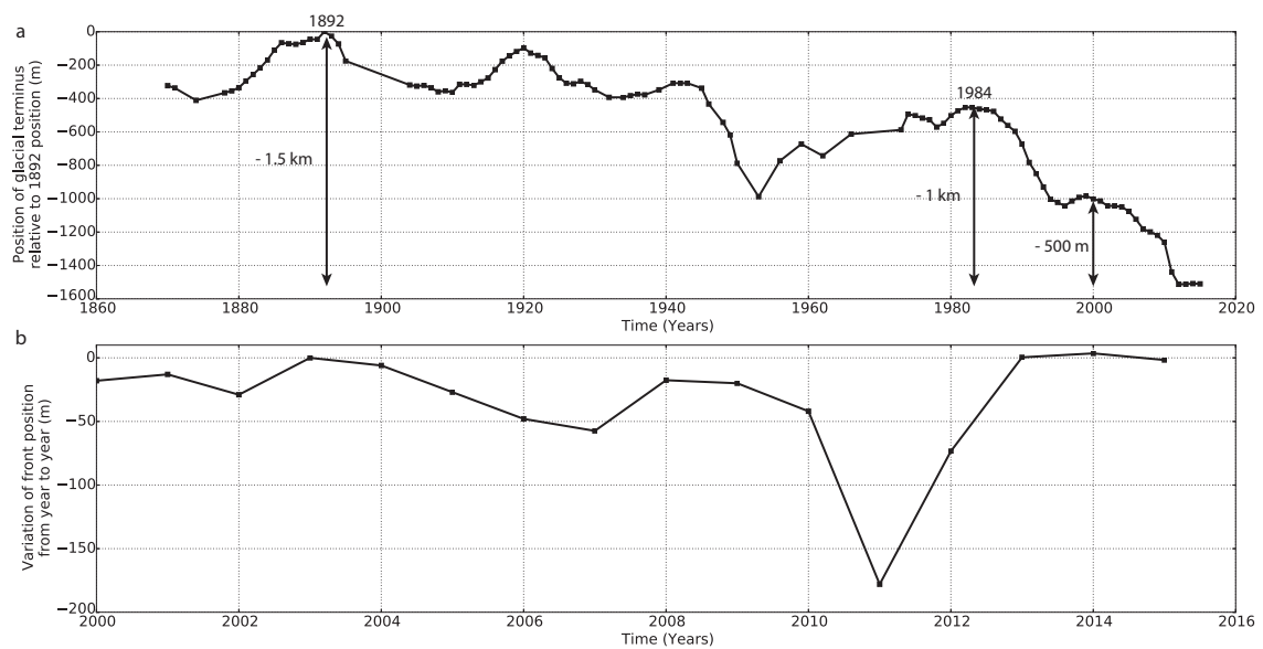
FIGURE 5.4 – Variations de la position du front du glacier des Bossons. a) Variations de la position du front du glacier des Bossons par rapport à l'avancée maximale de 1892 ; b) Variations inter-annuelles de la position du front du glacier des Bossons entre 2000 et 2015. Les données ont été produites et fournies par C. Vincent et D. Six du service d'observation GlacioClim.
