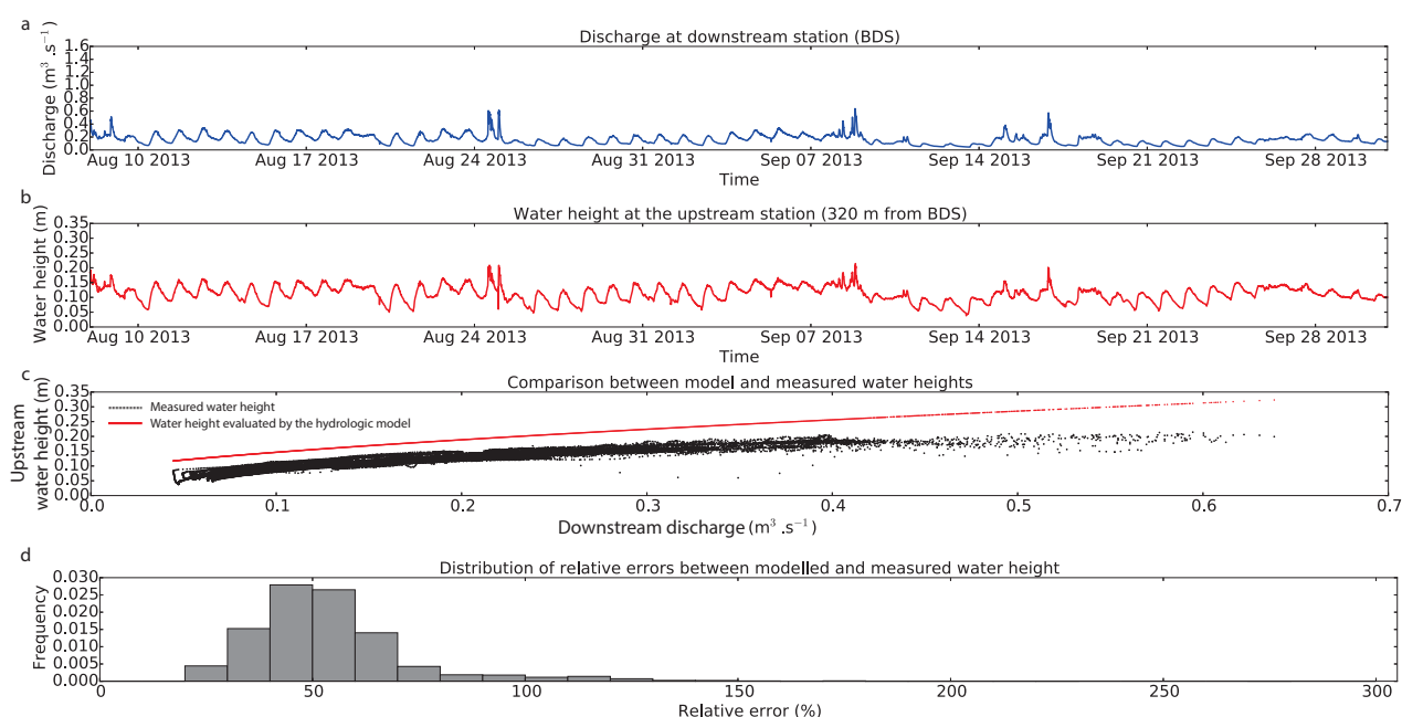
Figure 3.2 – Résultats du modèle hydraulique de la plaine alluviale. a) Débit mesuré à la station aval (BDS); b) Hauteur d'eau mesurée dans le chenal principal, 320 m à l'amont de la station aval; c) Relations entre débit et hauteur d'eau à la station amont et via la modélisation hydraulique (Annexe C.5). La densité des points souligne une hauteur d'eau variable pour un débit donné; d) Distribution des erreurs relatives entre hauteurs d'eau mesurées et modélisées.
