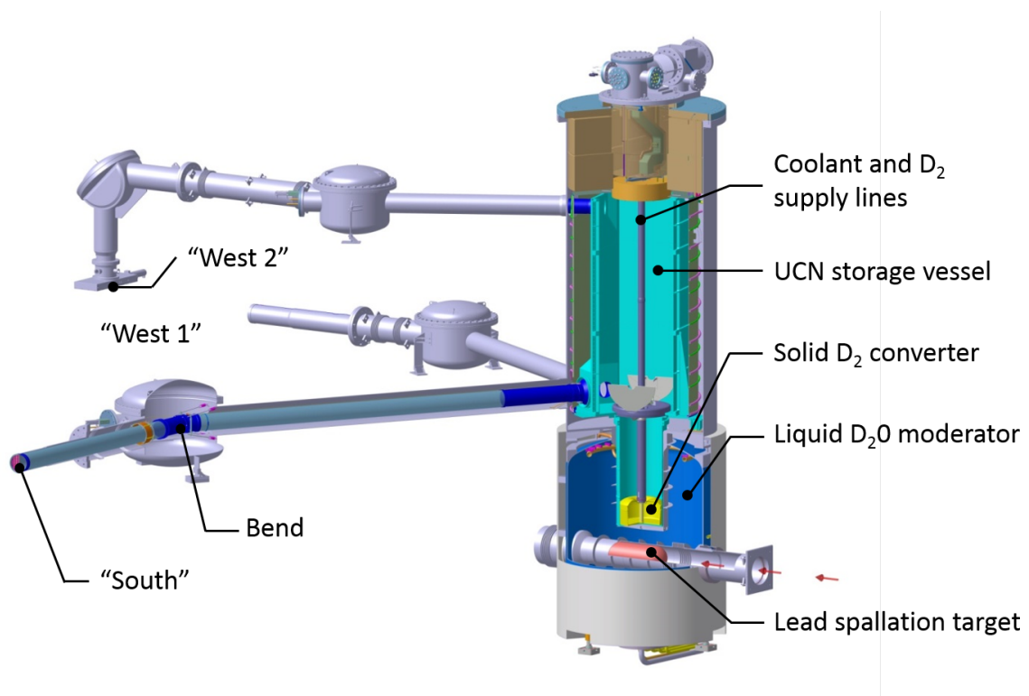
FIGURE 1.15 – Schéma détaillé de la source UCN de PSI. La hauteur de l'installation est de 7m. Le spectromètre nEDM est situé au bout de la sortie "South" de la source UCN.
