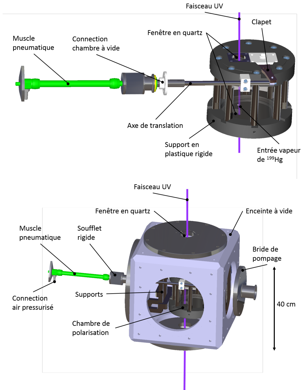
FIGURE 3.2 – En haut : Illustration du prototype de la chambre de polarisation conçue au LPSC pour l'expérience n2EDM, connecté à son système pneumatique d'ouverture/fermeture. En bas : Intégration du prototype dans une enceinte à vide permettant de tester dans des conditions réalistes la mécanique du clapet et du pompage optique.
