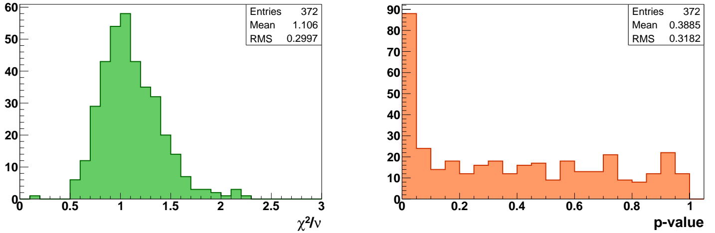
FIGURE 4.22 – À gauche : Distribution de \chi^2/\nu intégrant l'ensemble des ajustements de (Eq. 4.28) par \langle R \rangle^{\text{ssq}} . De même à droite : Distribution des p-value .
