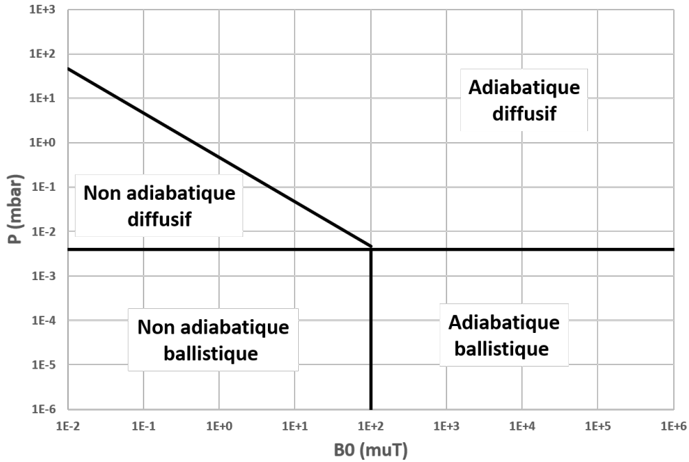
FIGURE 3.15 – Position des différents régimes de fonctionnement possible d'un magnétomètre atomique, ici dans le cas du ^{199}\text{Hg} , en fonction de la pression du gaz et du champ magnétique immergeant le volume de stockage.
