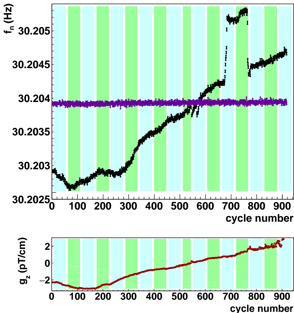
FIGURE 1.17 – Séquence de données #2 (run 10093-94-95) issue de la prise de données nEDM 2015. En haut, la fréquence neutron f_n avant ( \bullet ) et après ( \bullet ) correction des dérives de champ magnétique est tracé en fonction du numéro de cycle. Un cycle de mesure dure 300 s. Pour superposer ces deux quantités, le rapport des fréquences a été remis à l'échelle. Les bandes de couleur correspondent aux successives inversions de la direction du champ électrique espacées par 8 cycles à haute tension nulle. Le champ magnétique au bout de 3 jours de mesure a dérivé d'environ 100 pT. Après correction, les fluctuations observées proviennent uniquement de la statistique neutron (Eq. 1.56) et sont de l'ordre de 500 fT. En bas, évolution temporelle du gradient de champ magnétique vertical mesuré par l'ensemble des magnétomètres Cs.
