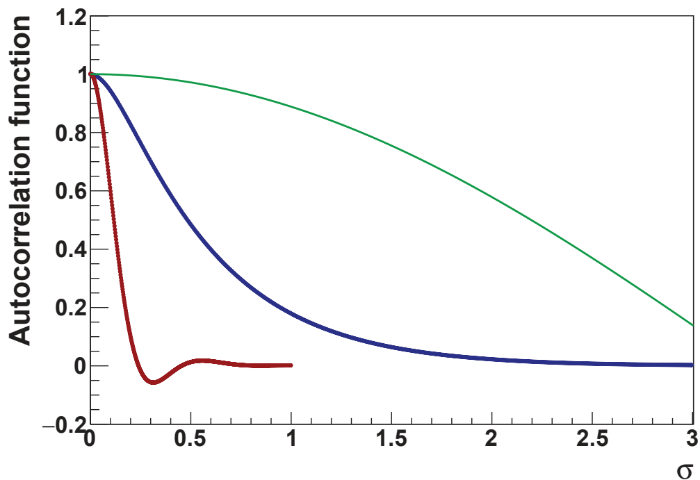
FIGURE 3.16 – En rouge(bleu) : fonction d’auto-corrélation R_\chi(R_\zeta) d’une particule balistique piégée dans un cylindre où a = 0.5 , dont le temps caractéristique de décroissance est \sigma_T^c(\sigma_L^c) . En vert : amplitude du terme \cos \omega_0 \tau .
