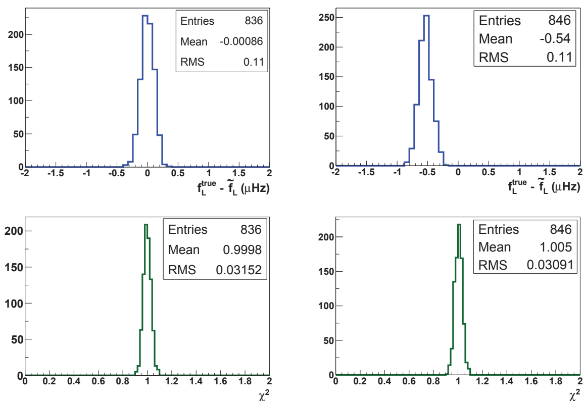
FIGURE 2.12 – Histogrammes représentant les distributions (en haut) : l'écart type de la distribution de l'écart de \tilde{f}_L à la valeur vraie ; (en bas) du \chi^2 réduit du dernier ajustement pour A = 20000 , \sigma_{\text{bruit}} = 30 , T_2 = 100 s, T_p = 180 s et T_{w1} = 20 s. A gauche, les résultats en l'absence de dérive de champ magnétique montrent que la procédure d'estimation de f_L est non biaisée, à droite, lorsque \delta B = 1 pT, l'estimateur est biaisé pour cette paramétrisation (il faudrait ici réduire la taille de la fenêtre d'ajustement T_{w1} ).
