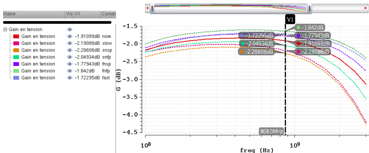
Figure VI-35 : Gain en tension en mode bypass pour les différents corners, V_{DD} = 1.1V
