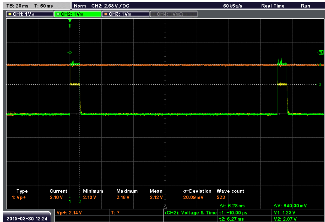
Figure VI-3 : Sorties des trois régulateurs de tension observées à l'oscilloscope, V_{bat} = 3.3V , T_{ambiente}
