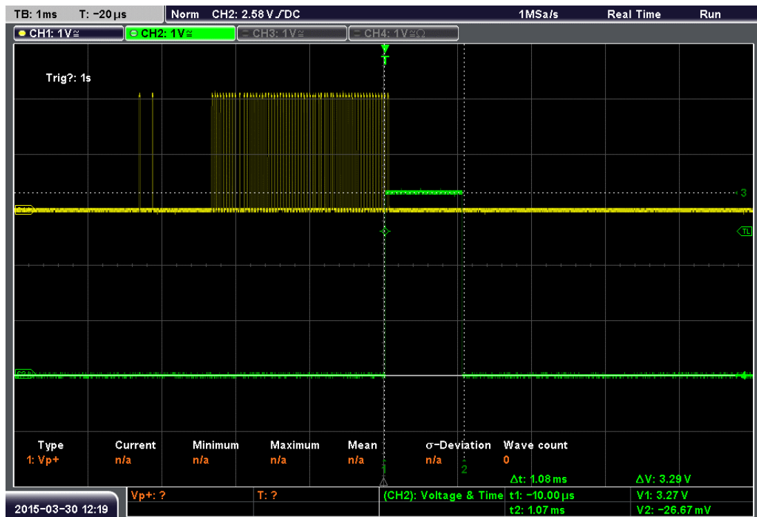
Figure VI-49 : Capture du signal démodulé retardé et du signal d'activation
