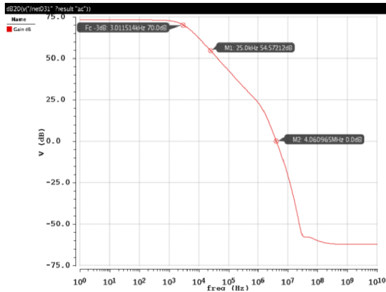
Figure VI-44 : Réponse en fréquence de l'amplificateur, cas nominal
