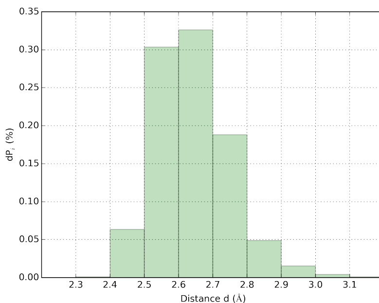
FIGURE III.27 : Distribution de distances de la liaison hydrogène entre Glu222/OE2 et Ser205/OG au cours de la dynamique de AvGFP (1W7S).
