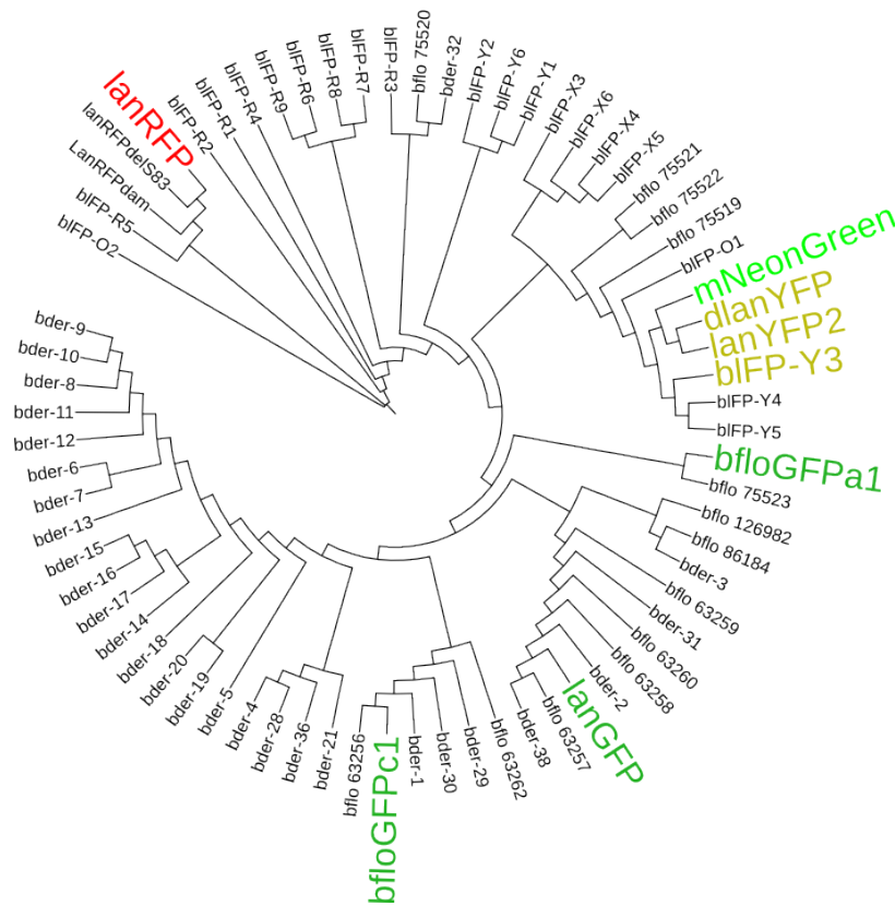
FIGURE II.23 : Arbre phylogénétique des séquences codantes pour de PF du genre Branchiostoma . bIFP : B. lanceolatum , bflo : B. floridae , bder : Branchiostoma [Mushegian et al., 2014, Israelsson, 2013, Putnam et al., 2008]
