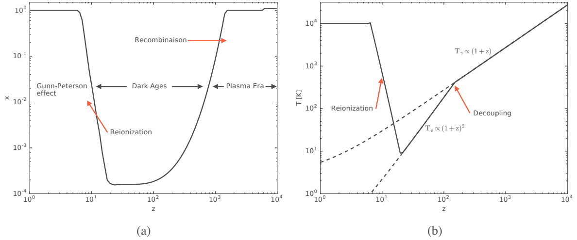
FIGURE 1.2 – Panneau (a) : Schéma de l’histoire d’ionisation de l’Univers à grand redshift. À très haut redshift l’Univers est complètement ionisé. Avec l’expansion la température diminue et provoque plusieurs recombinaisons ( H_e III \rightarrow H_e II à \sim 7000 et H_e II \rightarrow H_e I à \sim 2500 ), mais la principale est la recombinaison de l’hydrogène ( H II \rightarrow H I à \sim 1100 ). À bas redshift, l’Univers est réionisé par les sources UV ( z \leq 10 ). Cette figure est extraite (et simplifiée) de Sunyaev & Chluba (2009) . La fraction de neutre sur ce schéma est en fait le rapport de la densité d’électrons libres par la densité d’atome d’hydrogène. À très haut redshift, x > 1 car il faut compter les atomes hélium. Panneau (b) : Schéma de l’histoire de température de l’Univers à grand redshift. À très haut redshift, la température des électrons, T_e est couplée à la température des photons du CMB, T_\gamma . Au découplage, z \sim 150 , la densité résiduelle d’électrons libres est trop faible pour interagir avec les photons du CMB. Le gaz suit alors une expansion adiabatique. À la fin des Ages sombres, les premières étoiles chauffent et ionisent le gaz, à la fin de la Réionisation la température du gaz est T_e \sim 10^4 K. Cette figure est inspirée de Loeb & Furlanetto (2013) .
