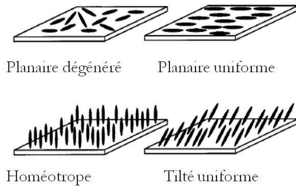
Figure 13 : types d'ancrages sur un substrat (Dierking, 2006)
