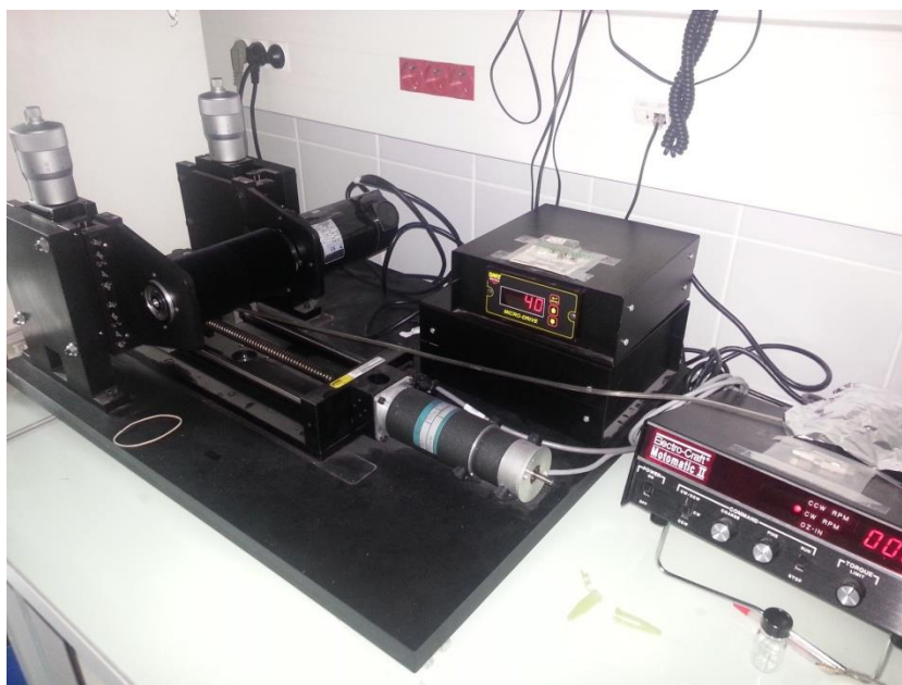
Figure 29 : machine à frotter utilisée pour orienter les surfaces de polymère
