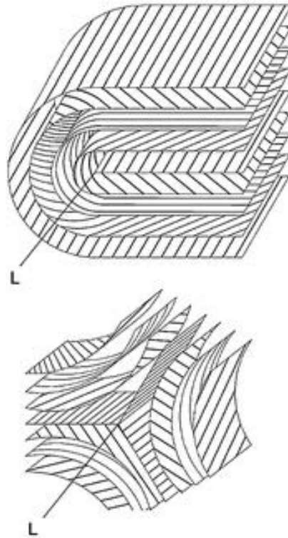
Figure 6 : défauts de type disinclinaison (Rey), disinclinaison à courbure positive (haut) et à courbure négative (bas)
