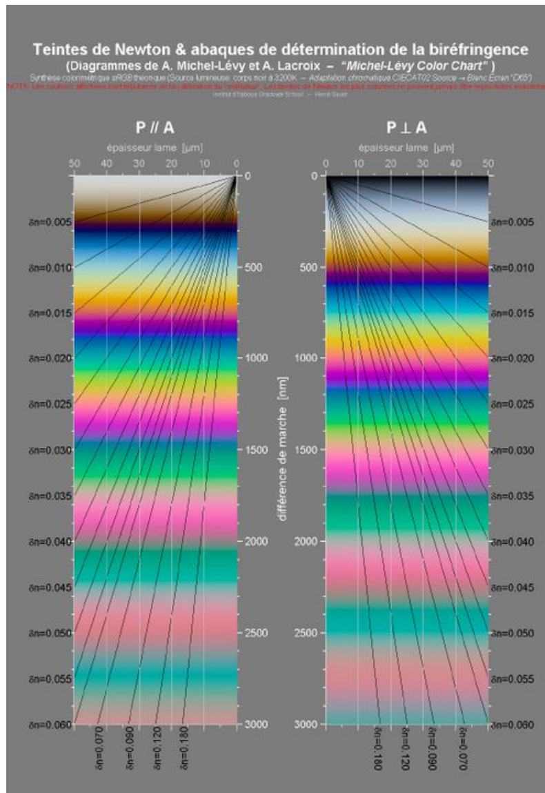
Figure 31 : abaque des teintes de Newton, présentant la couleur en fonction de la différence de marche (double de l'épaisseur du film fois son indice optique), suivant que l'analyseur est parallèle ou perpendiculaire au polariseur.
