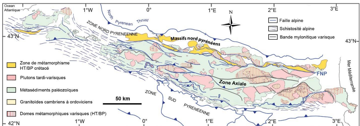
Figure 1-13: Carte géologique simplifiée des Pyrénées, avec localisation du socle varisque à l'affleurement et des zones affectées par les déformations alpinnes (d'après Choukroune & Séguret, 1973a et Izquierdo-Llavall et al., 2013b).
