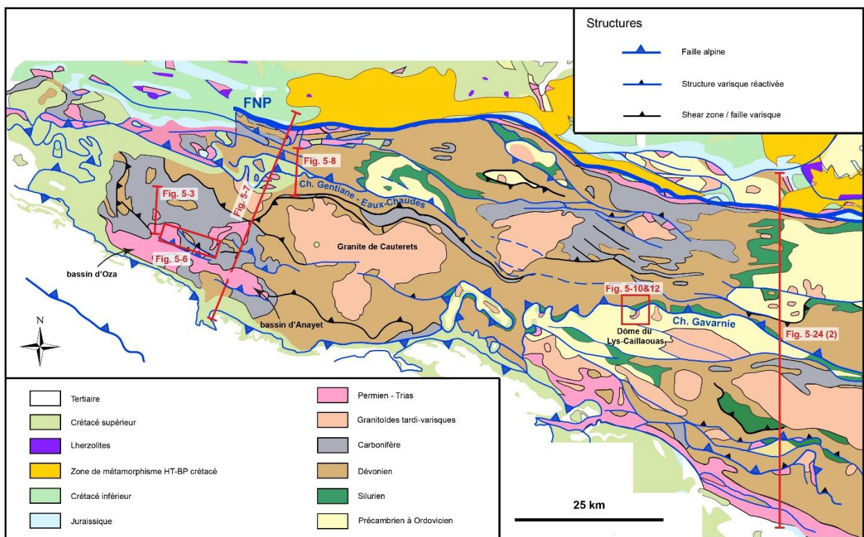
Figure 5-4: Carte géologique simplifiée de l'Ouest de la Zone Axiale avec localisation des coupes et cartes présentées et discutées dans le texte.
