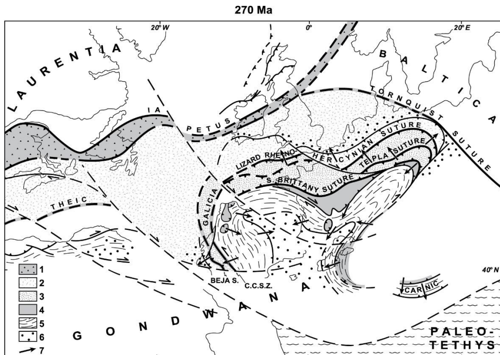
Figure 1-12: Configuration de la chaîne varisque ouest-européenne au Permien d'après ( Matte, 2001 ). 1- Suture de l'océan Iapetus ; 2- Avalonia, 3- Armorica, 4- Nappes ophiolitiques, 5-Nappes sud de la chaîne, 6- bassins d'avantpays carbonifères, 7- Vergence des nappes.
