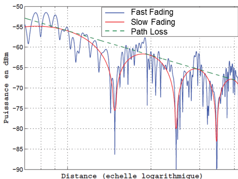
Figure III-14 : Les variations de la puissance reçue en fonction de la distance [82]
