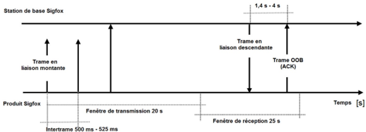
Figure II-37 : Communication en mode bidirectionnel
