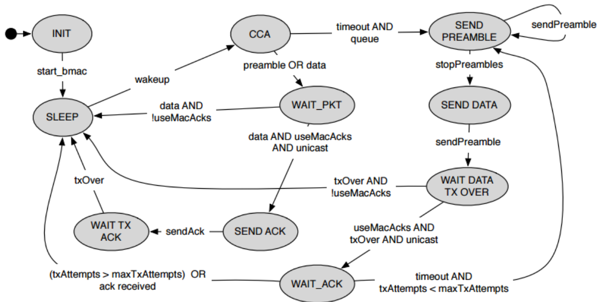
Figure V-7 : La machine à états du protocole B-MAC déjà existant sur MiXiM
