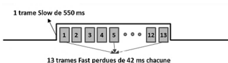
Figure IV-17 : Le nombre des trames Fast perdues lors d'une transmission Slow simultanée
