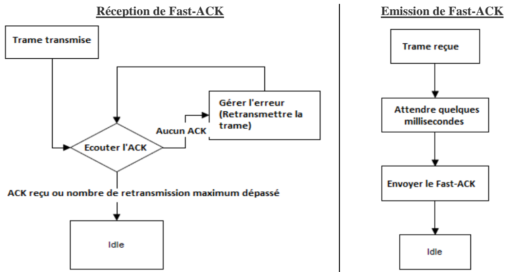
Figure II-6: Algorithmes d'acquittement KNX (Rx / Tx)
