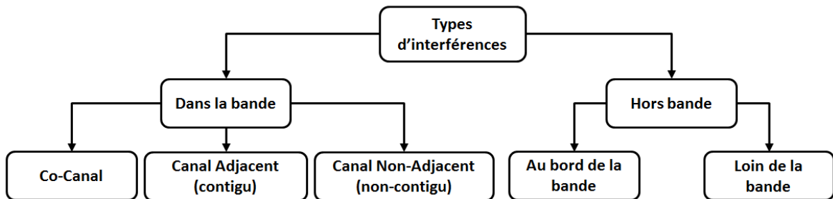
Figure I-4 : Les différents types d'interférences radio dans le domaine fréquentiel
