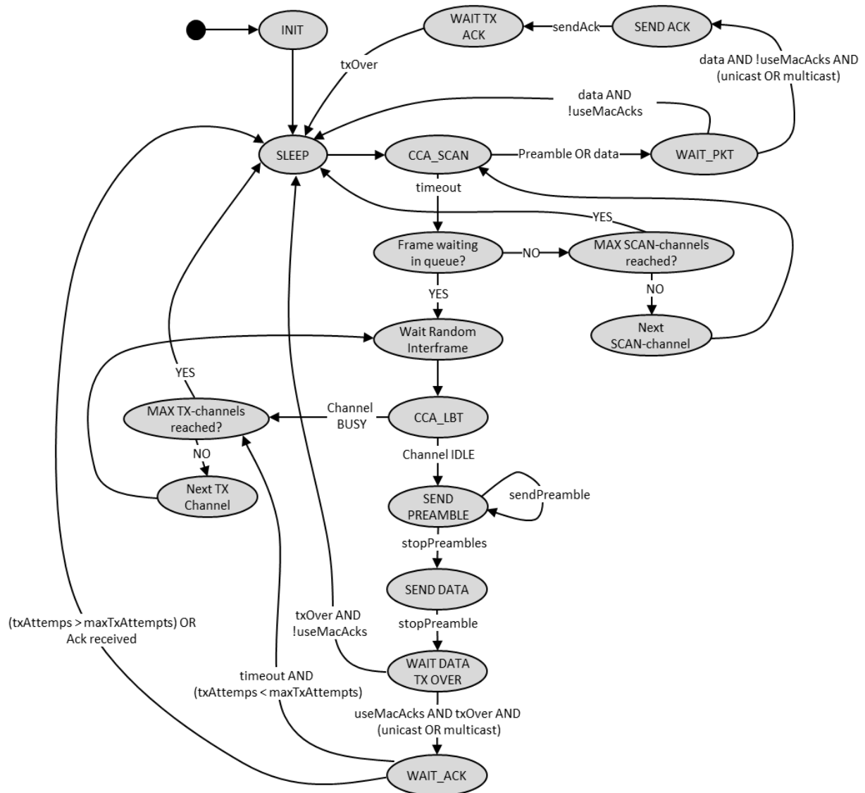
Figure V-9 : Machine à états de la couche MAC_KNX_RF implémenté sur MiXiM
