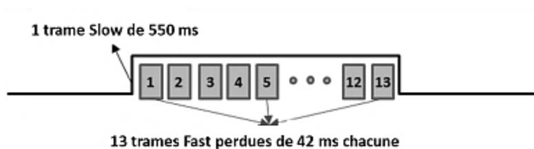
Figure IV-17 : Le nombre des trames Fast perdues lors d'une transmission Slow simultanée
