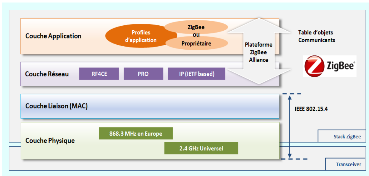
Figure II-11 : La stack du protocole ZigBee
