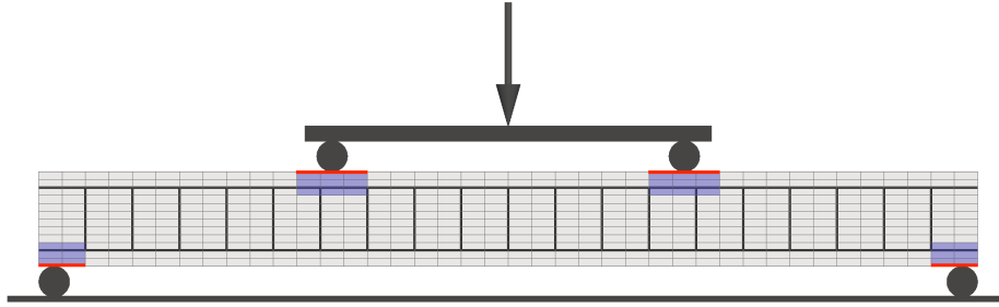
Figure E.8: Essai de flexion – zones d’applications des conditions aux limites (rouge)
