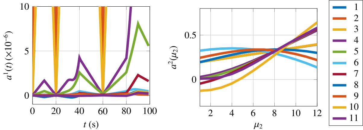
(a) Fonctions du temps \{a_i^1(t)\}_{i=1\dots 11}
