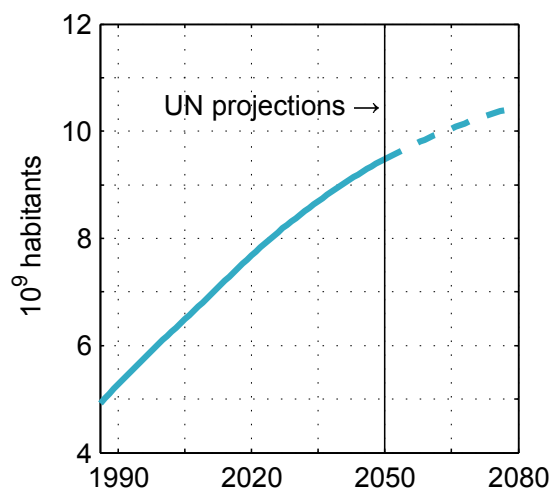
Figure 3.4 : Projection de la population mondiale selon le scénario moyen des Nations Unies.
