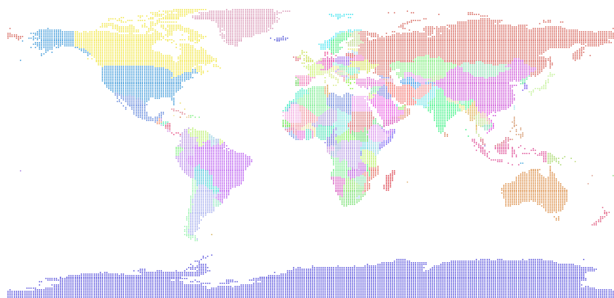
Figure 3.5 : Représentation des mailles du modèle CCSM4 correspondant à chaque pays.
