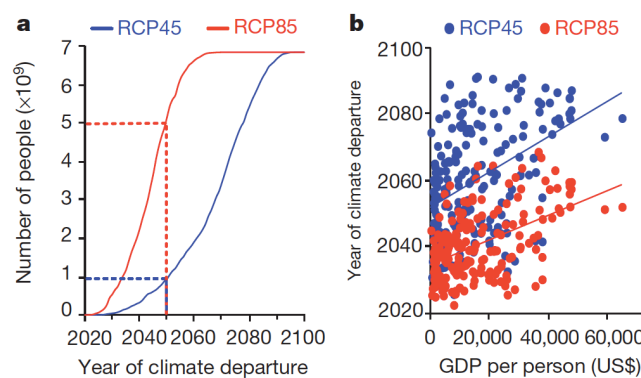
Figure 2.2 : (a) Cumul du nombre de personnes en fonction des années auxquelles la température globale annuelle de l'endroit où ils vivent dépassera l'enveloppe minimum-maximum de la période 1860-2005. Les pointillés correspondent à l'année 2050. (b) Relation entre le PIB par habitant et l'année moyenne de l'émergence du changement de température. Le RCP4.5 est représenté en bleu, alors que le RCP8.5 est représenté en rouge (tiré de Mora et al., 2013).
