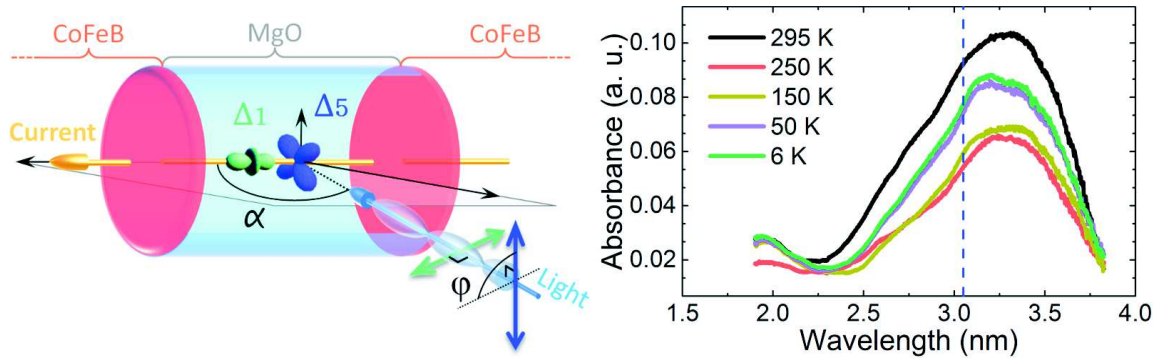
FIGURE AVI : Géométrie de l'excitation optique : (a) Un courant tunnel dominé par des états \Delta_1 ou \Delta_5 traverse la barrière de MgO (en bleu transparent). La direction de propagation de photons fait un angle \alpha par rapport à la normale à la surface de l'échantillon. L'angle entre la direction de propagation du courant I et le champ électrique de la lumière est dénoté \phi . (b) Dépendance en énergie de l'absorption optique d'une couche de MgO d'épaisseur 2.5 nm déposée par pulvérisation cathodique.
