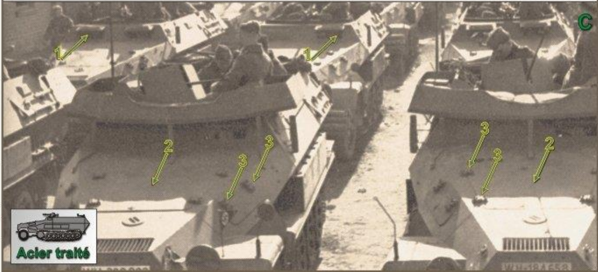
Planche AIV.001. Le Sd.Kfz. 251 en acier doux.
