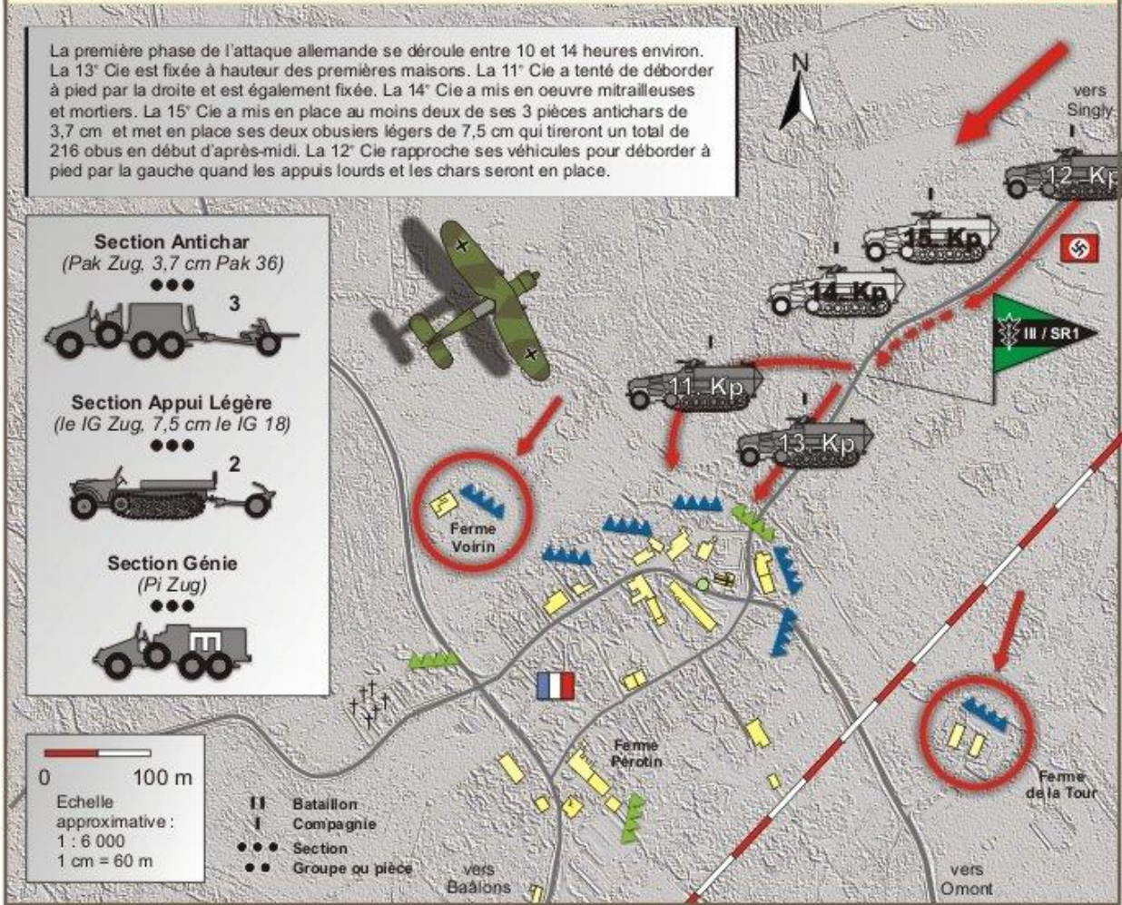
Planche C3.004. Portée des canons de la 3 e BS. Mode d'action allemand.
