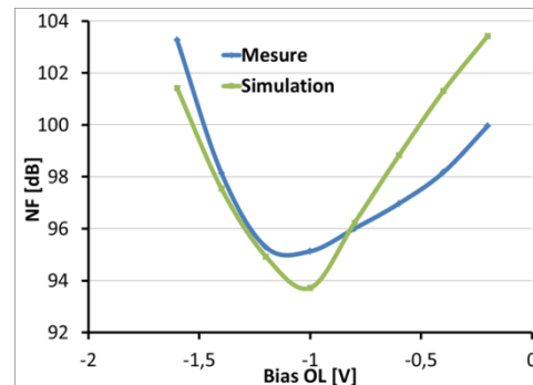
Figure 209 : NF en fonction du bias de l'EML (OL), architecture EML EAM série
