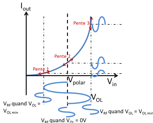
Figure 17 : Principe du mélangeur à diode
