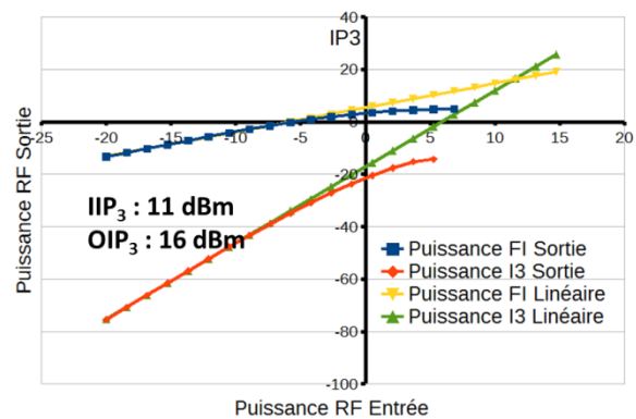
Figure 134 : IP_3 de l'architecture 4 avec EDFA
