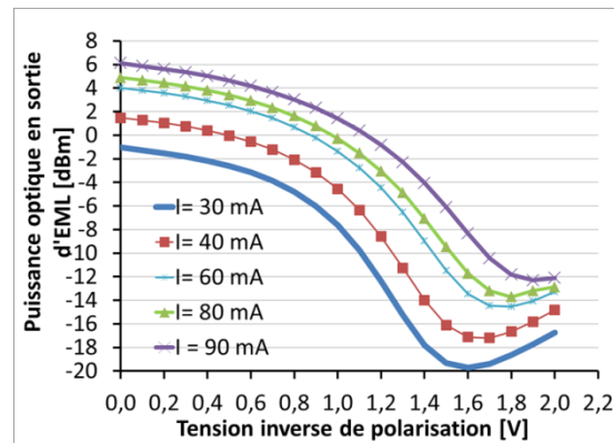
Figure 173 : Courbe d'absorption (statique) de l'EML pour plusieurs courants de polarisation
