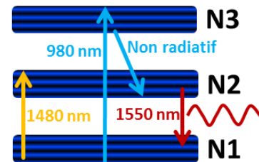
Figure 70 : Niveaux d'énergie dans la fibre dopée erbium
