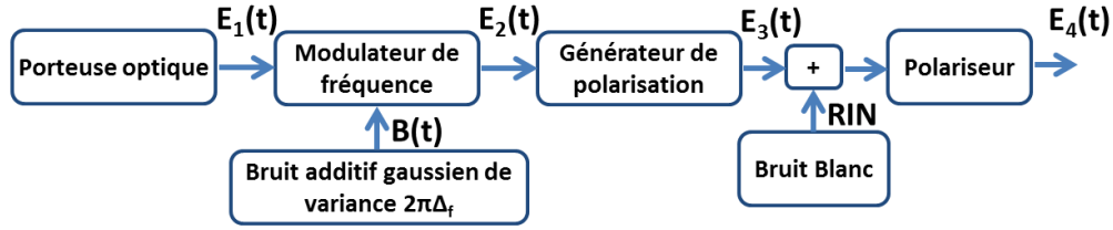
Figure 64 : Modélisation du laser DFB CW
