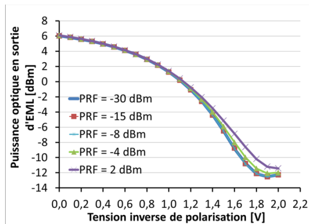
Figure 175 : Evolution de la courbe d'absorption d'un EML en fonction de la puissance électrique d'entrée, f = 8\text{ GHz} , I = 90\text{mA} , T = 25\text{ °C}
