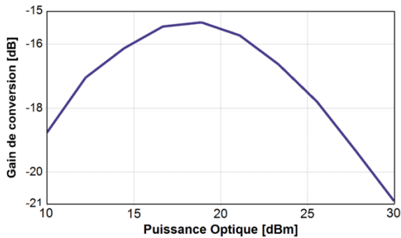
Figure 151 : Gain de conversion en fonction de la puissance optique, architecture SOA série
