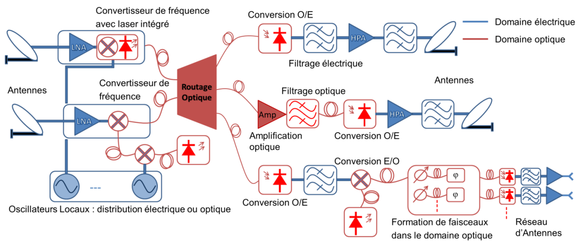
Figure 31 : La photonique au sein d'une charge utile transparente
