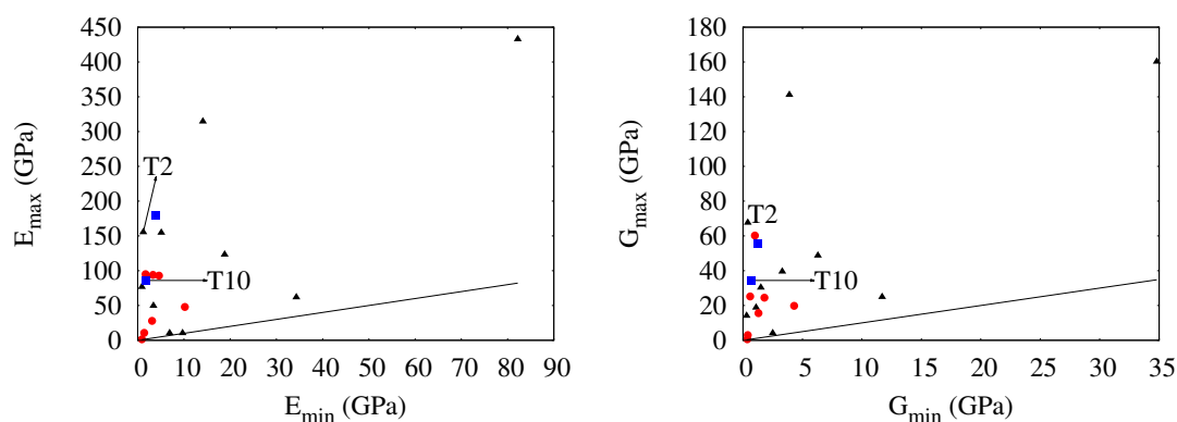
FIGURE 5.4 – Valeurs maximales des modules d’Young (à gauche) et de cisaillement (à droite), en fonction de leurs valeurs minimales. Les triangles noirs correspondent aux polymorphes ne contenant pas d’anneaux boroxol, les carrés bleus à ceux en contenant 50%, et les cercles rouges aux cristaux composés à 100% d’anneaux boroxol. La droite noire représente la première bissectrice y = x , et sert de guide pour l’oeil. Nous avons indiqué les polymorphes T2 et T10, sur lesquels nous reviendrons par la suite.
