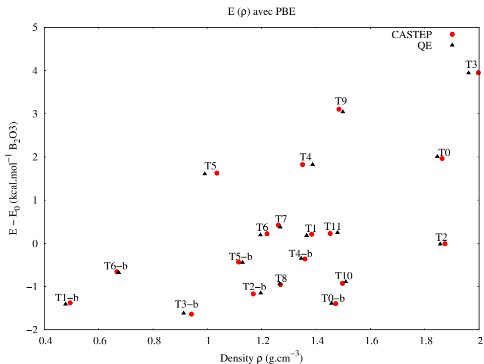
FIGURE A.1 – Energies de certains polymorphes de prédits de B_2O_3 (en kcal.mol -1 B 2 O 3 ) en fonction de leur densités, calculées avec la fonctionnelle PBE, et les pseudo-potentiels ultrasofts générés par CASTEP (triangles noirs) et Quantum Espresso (cercles rouges).
