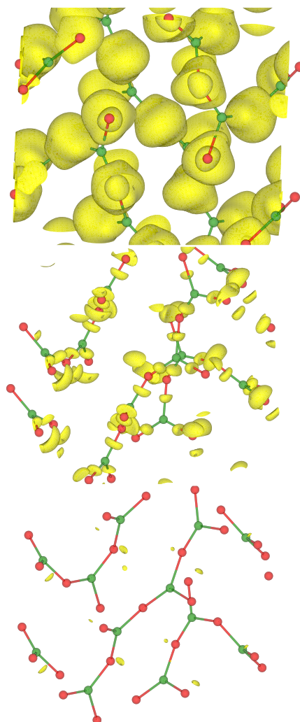
FIGURE 4.2 – Isosurfaces présentant l'ELF calculée en rVV10 sur le cristal B_2O_3 -I, pour une valeur de 0.75 (en haut), 0.85 (au milieu), et 0.91 (en bas). Les atomes de bore sont présentés en vert, ceux d'oxygène en rouge, et l'isosurface présentant l'ELF en jaune.
