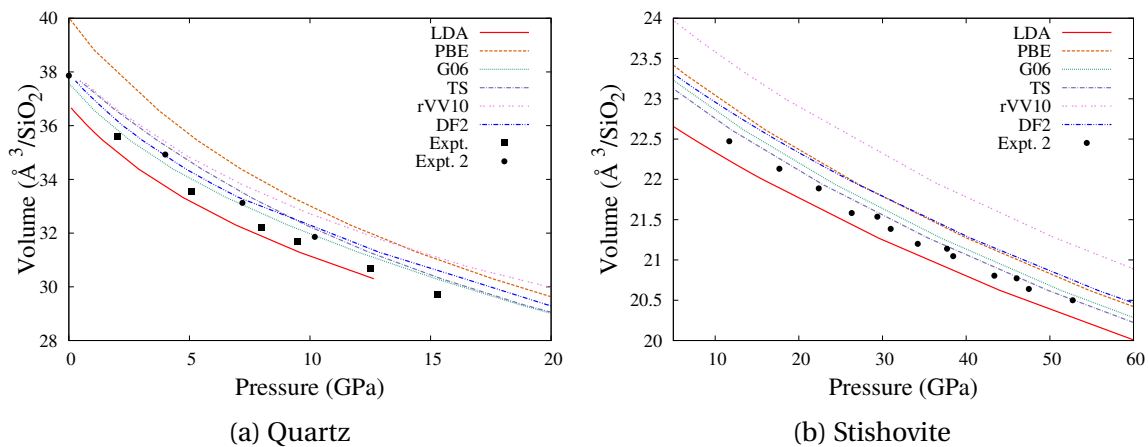
FIGURE 3.8 – Équations d'état du quartz et de la stishovite, calculées avec différentes fonctionnelles DFT. Les points notés « Expt. » sont issus de la référence [30] et ceux notés « Expt. 2 » de la référence [4].
