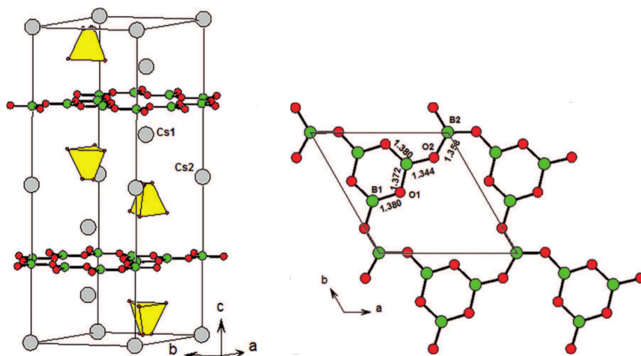
FIGURE 5.9 – A gauche, structure atomique du borosulfate Cs_3H(SO_4)_2(B_2O_3)_2 synthétisé par Daub et Hillebrecht, et a droite, structure du feuillet de B_2O_3 intercalé dans le cristal de Cs_3H(SO_4)_2(B_2O_3)_2 .
