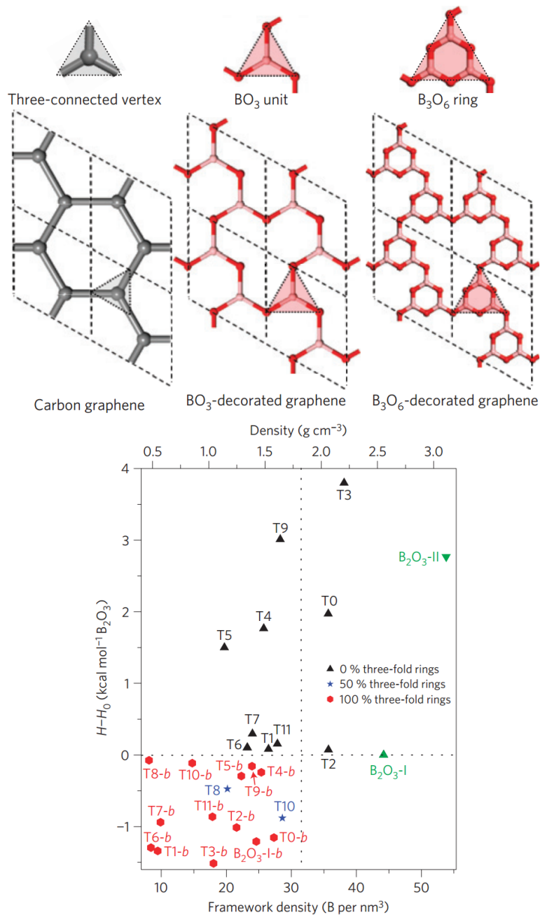
FIGURE 1.3 – En haut, illustration de la méthode utilisée pour généré de nouvelles structures cristallines de B 2 O 3 , et en bas, figure présentant les énergies relatives (calculées à T = 0 K et P = 0 Gpa) de ces nouveaux polymorphes et leur densités. Ces deux figures sont issues de la référence [5].
