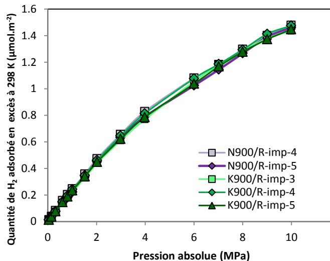
Figure 5.18 : Isothermes en quantité d'hydrogène adsorbées par unité de surface spécifique
