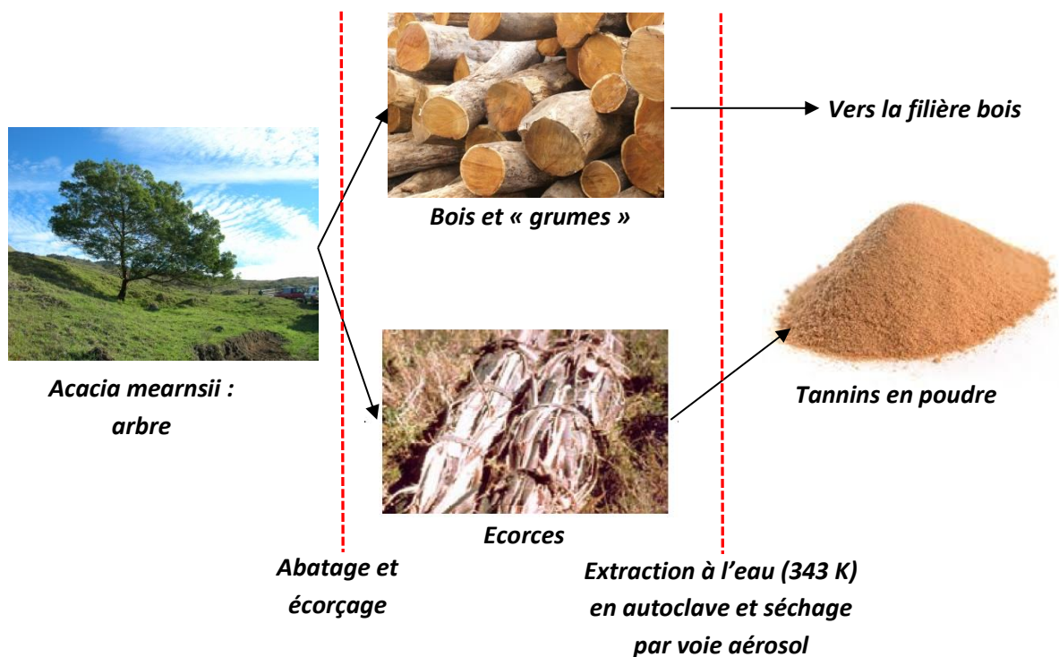
Figure 5.26 : Procédé d'obtention des tannins à partir de l'écorce d' Acacia mearnsii
