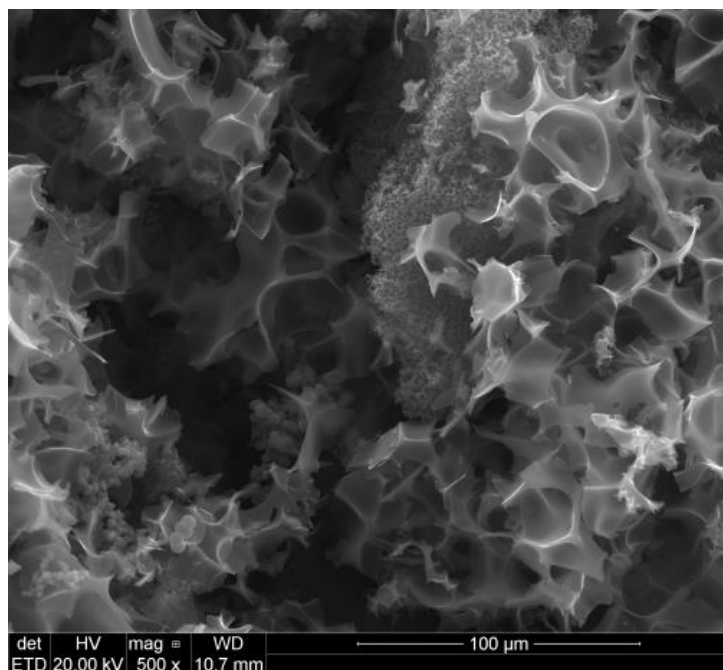
Figure 3.21 : Clichés de microscopie électronique à balayage du matériau AchTC_0.8_4
