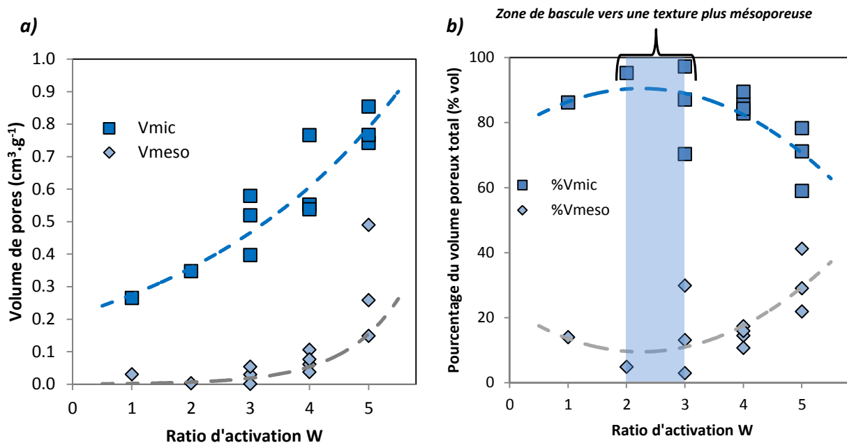
Figure 3.31 : Variation des volumes poreux (a) et de leurs pourcentages (b) pour tous les matériaux issus d'hydrochars en fonction du ratio d'activation W . Vmic et Vmeso sont respectivement les volumes des micropores et des mésopores.
