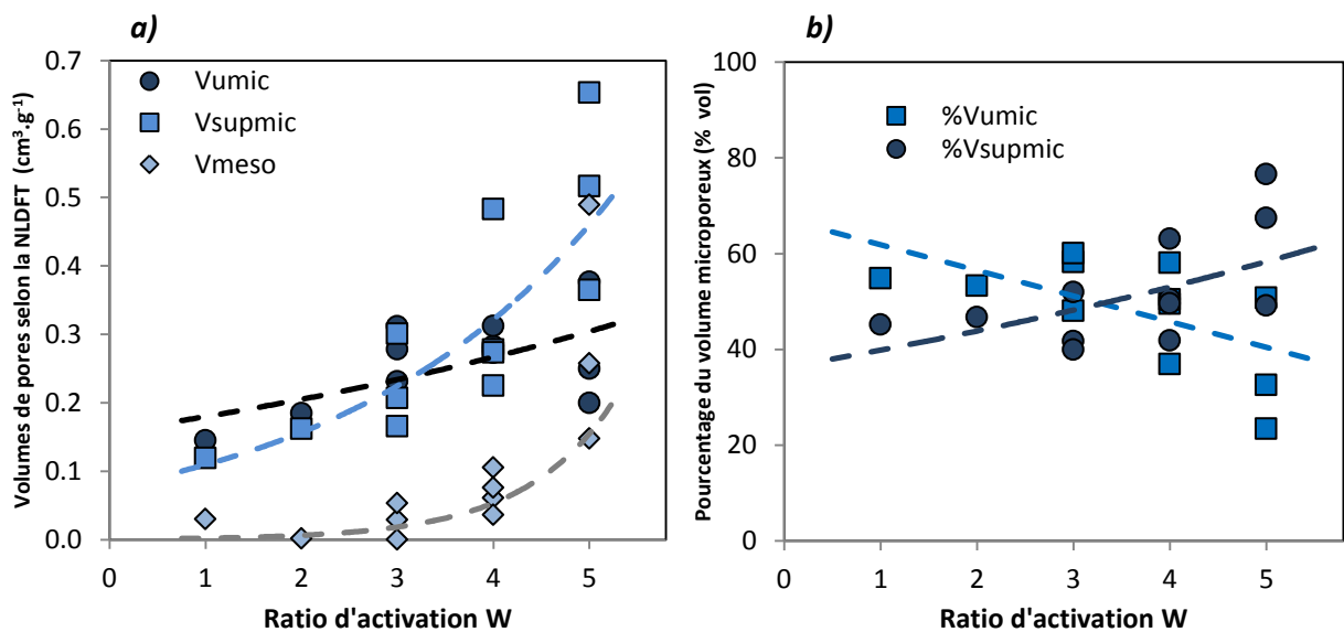
Figure 3.32 : (a) Volumes des ultramicropores, des supermicropores et des micropores ainsi que (b) leurs fractions respectives, en fonction du ratio d'activation W . V_{\text{mic}} , V_{\text{supmic}} et V_{\text{meso}} sont respectivement les volumes des supermicropores, des supermicropores et des mésopores.
