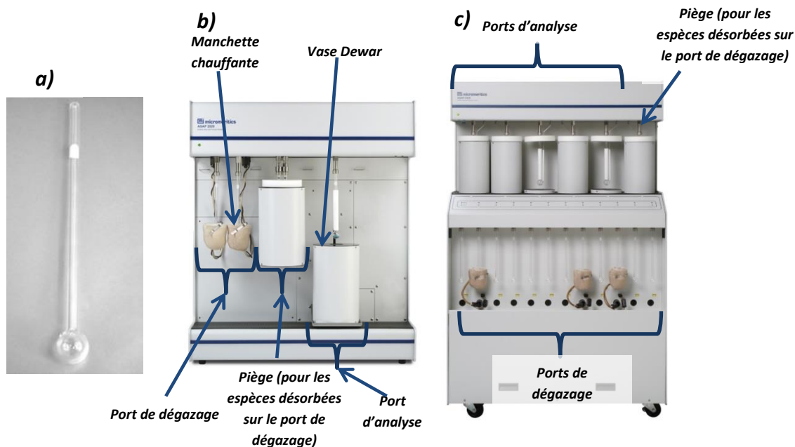
Figure 2.4 : Appareils d'adsorption manométriques utilisés pour la caractérisation au laboratoire : a) Porte échantillon (cellule d'analyse), b) ASAP 2020, c) ASAP 2420
