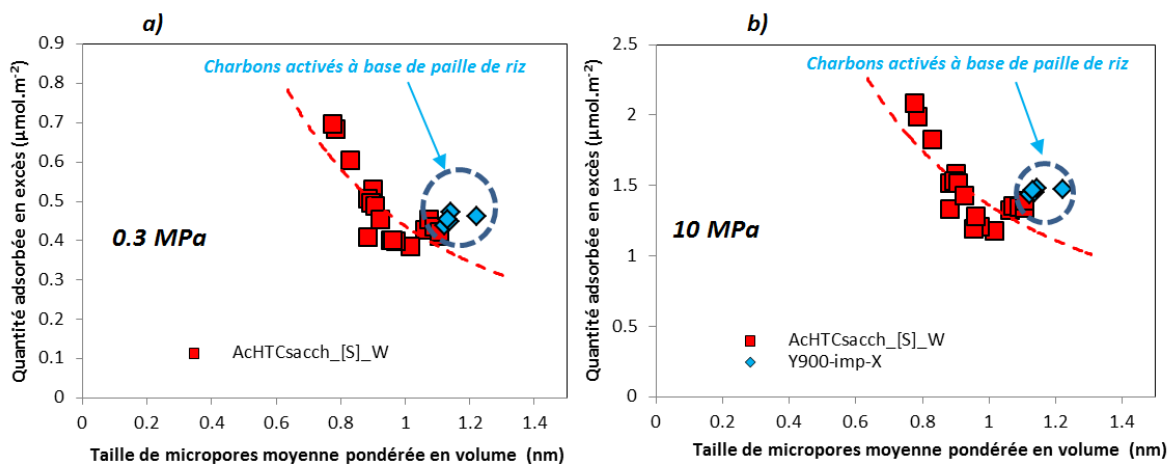
Figure 5.19 : Quantité d'hydrogène adsorbée par unité de surface en fonction de la taille moyenne des micropores : (a) à 0.03 MPa, (b) à 10 MPa.
