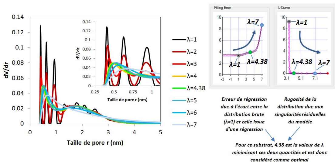
Figure 2.9 : Effet du paramètre de lissage \lambda sur une distribution de tailles de pores d’un charbon activé
