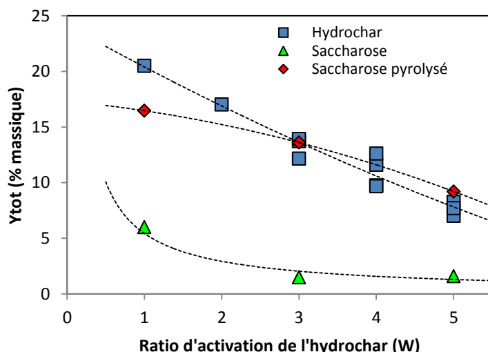
Figure 3.18 : Rendements totaux de synthèse pour les trois précurseurs des charbons activés
