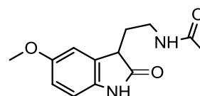
Oxindole (2-OMEL)
