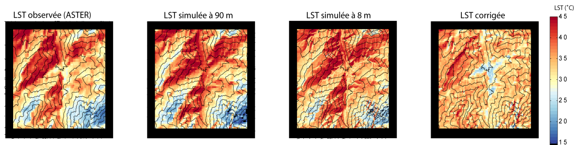
FIGURE 5.1 – Images de la LST observée par ASTER, simulée à 90 m, simulée à 8 m et corrigée des effets topographiques (éclairage, altitude) le 05 septembre 2014. Les lignes noires représentent les courbes de niveau entre 1800 et 3600 m avec un incrément de 200 m.
