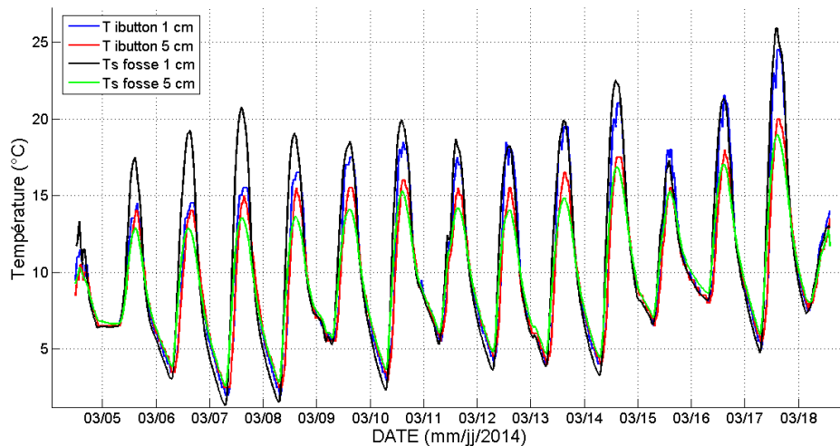
FIGURE 5.3 – Comparaison des thermochrons ibuttons avec les températures de fosse sur le site de Lamasquère, France
