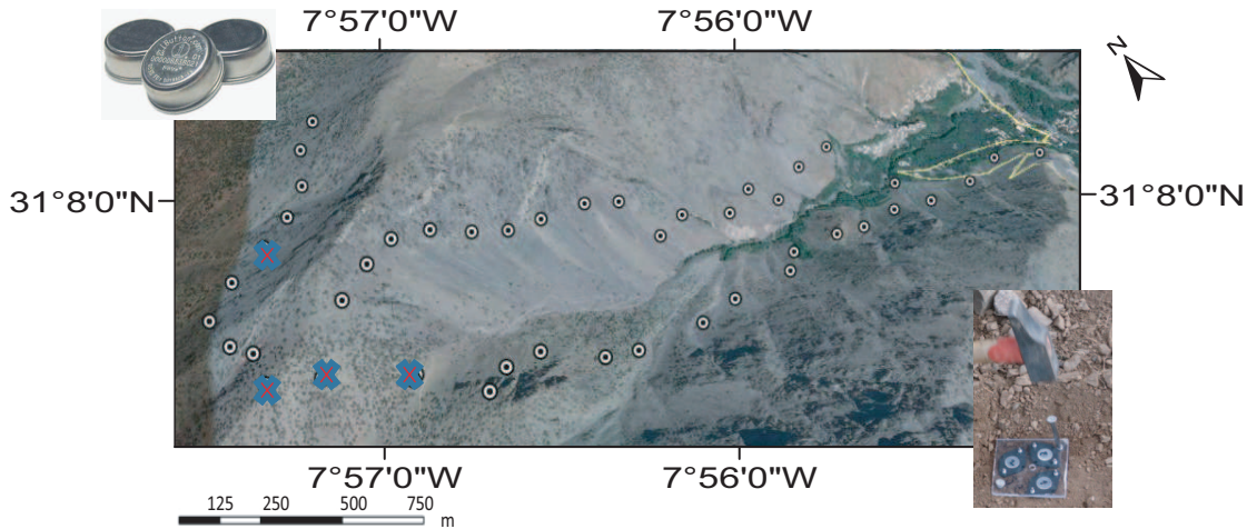
FIGURE 5.2 – Localisation des thermomètres dans la vallée d'Imlil.
