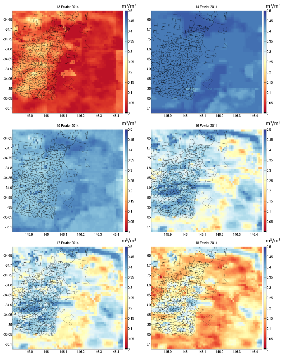
FIGURE 4.4 – Cartes des SSM désagrégées et assimilées sur la zone de Yancho, montrant la progression d'un événement pluvieux autour du 14 Février 2014.
