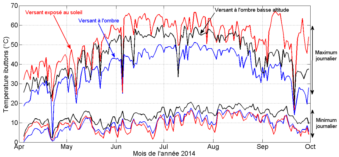
FIGURE 5.5 – Variations temporelles des maxima et minima journaliers de la température mesurée par les thermocrons ibuttons sur un versant exposé au soleil (rouge), à l'ombre (bleu) pour une même altitude (2450 m) et sur un versant à l'ombre à 1800 m d'altitude (noir).
