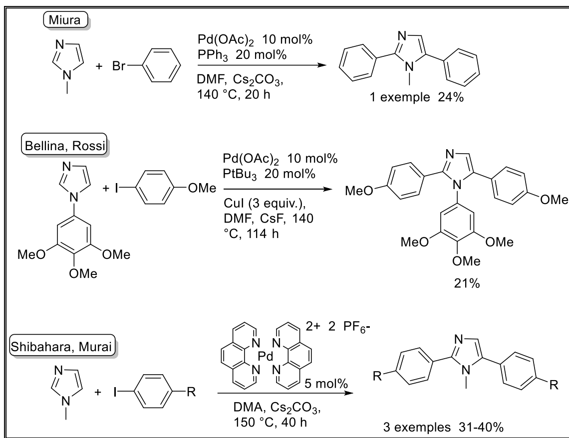
Schéma 32 : Exemples de diarylations d'imidazole Pd-catalysées en une seule étape
