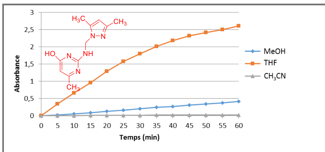
Figure 33 : Oxydation du catéchol en présence de L6 et \text{CuSO}_4 dans différents solvants
