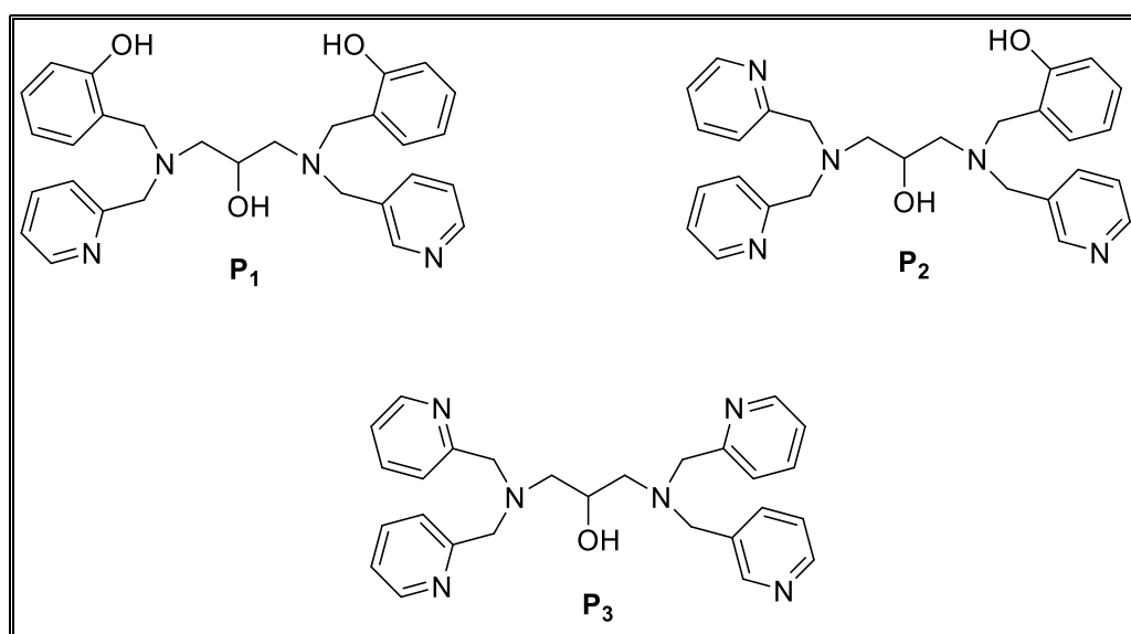
Schéma 56 : Structures des ligands P1-P3
