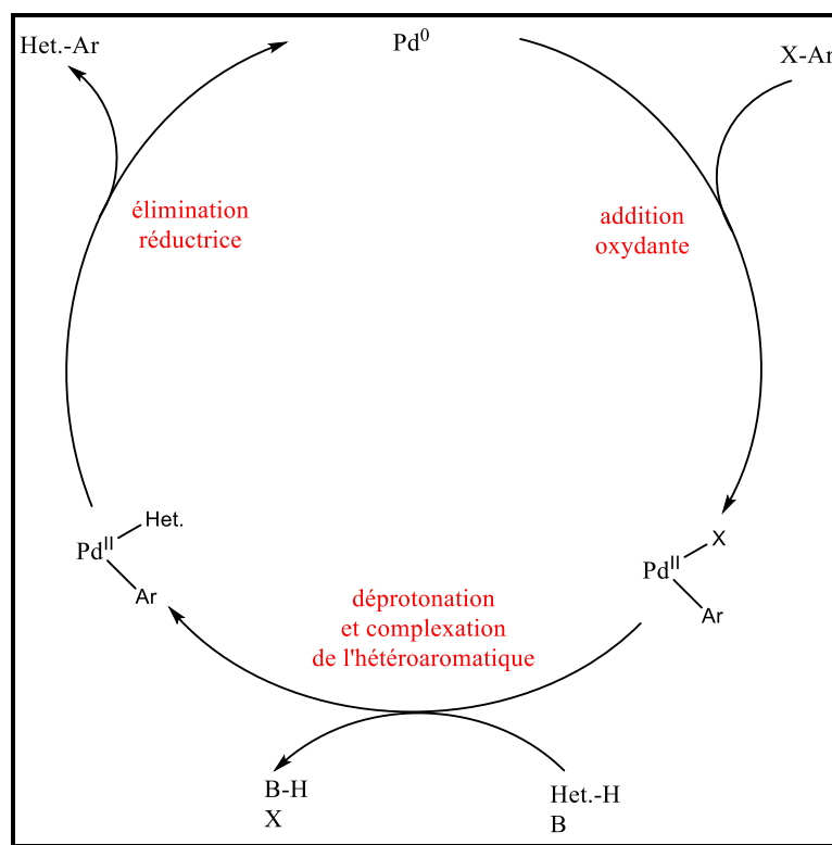
Schéma 11 : Cycle catalytique général
