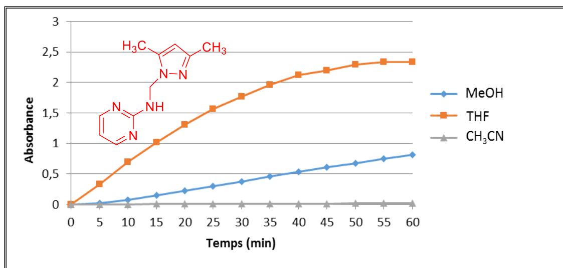
Figure 35 : Oxydation du catéchol en présence du ligand L 7 et CuSO 4 dans différents solvants
