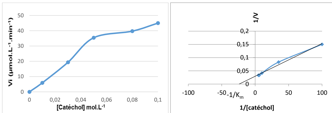
Figure 57 : Représentation graphique des V_i en fonction de la concentration du substrat pour la combinaison L_{12}/Cu(CH_3COO)_2
