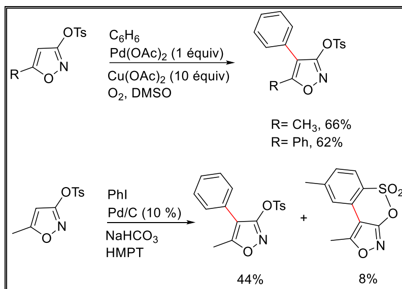
Schéma 1 : Exemple 1 de l'arylation directe Pd-catalysée
