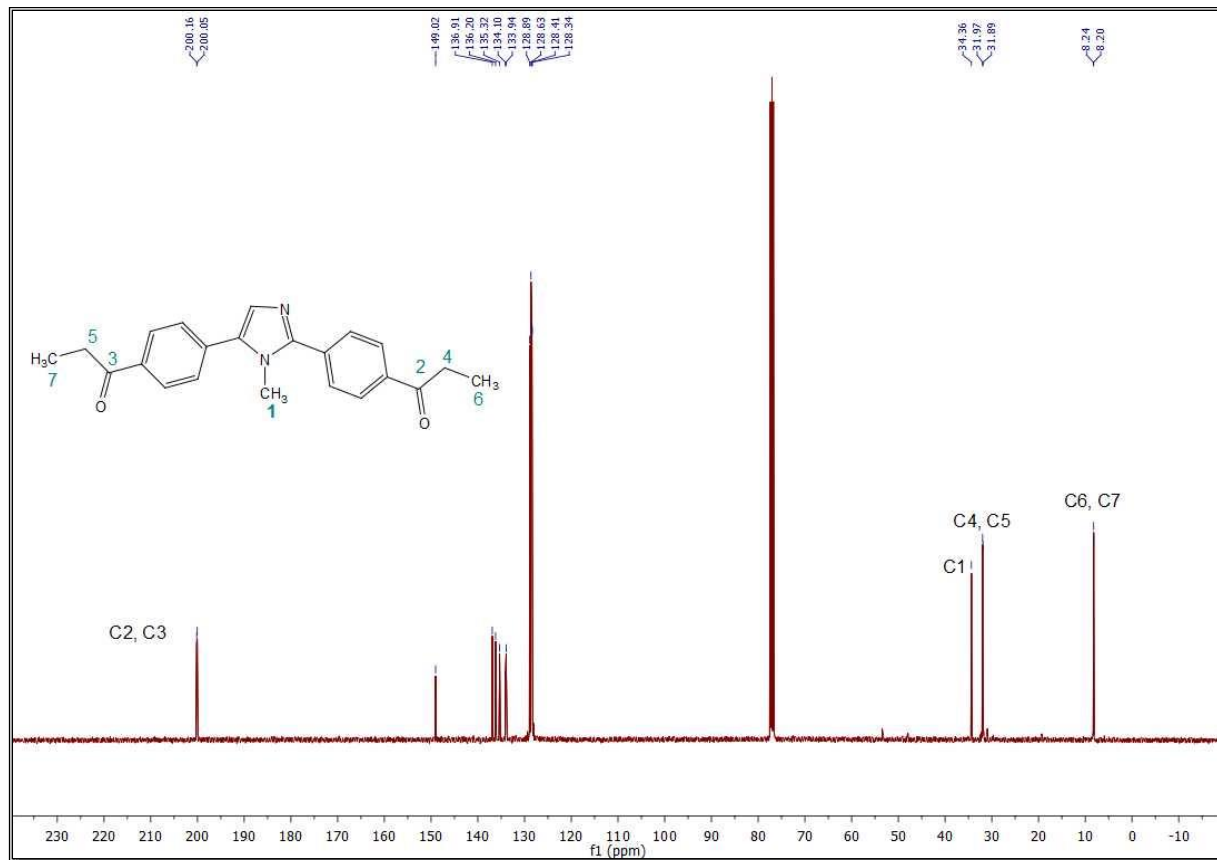
Figure 6 : Spectre RMN ^{13}\text{C} du composé 28 enregistré dans \text{CDCl}_3 à 100 MHz
