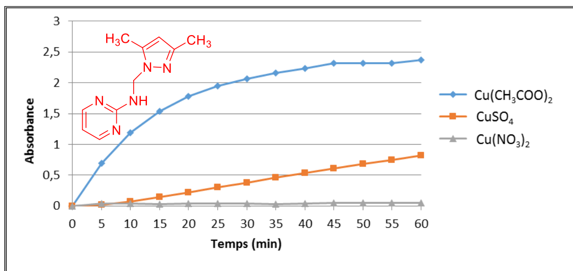
Figure 31 : Oxydation du catéchol en présence du ligand L7 (L/M : 1/2)
