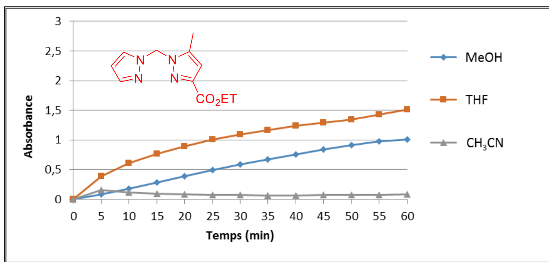
Figure 53 : Oxydation du catéchol en présence du ligand L 12 (L/M : 1/2) Cu(CH 3 COO) 2
