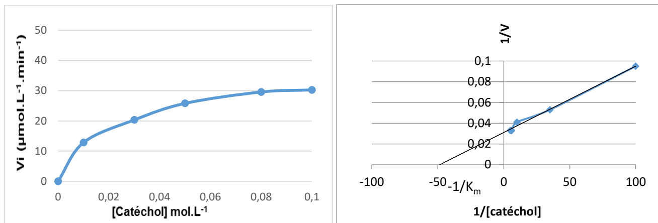
Figure 37 : Représentation graphique des V_i en fonction de la concentration du substrat pour la combinaison L_6/CuSO_4
