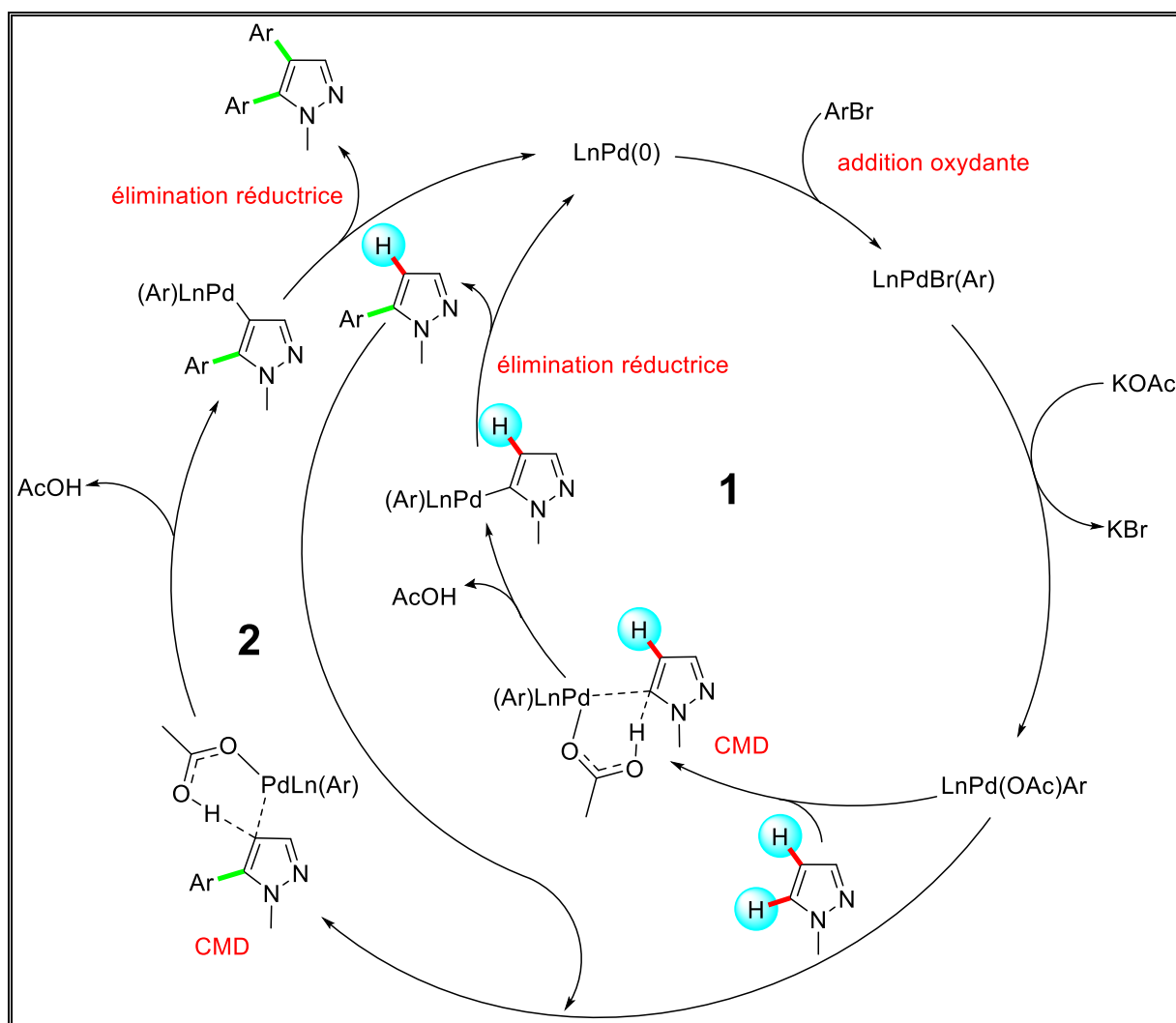
Schéma 30 : Mécanisme proposé pour la diarylation du 1-méthylpyrazole
