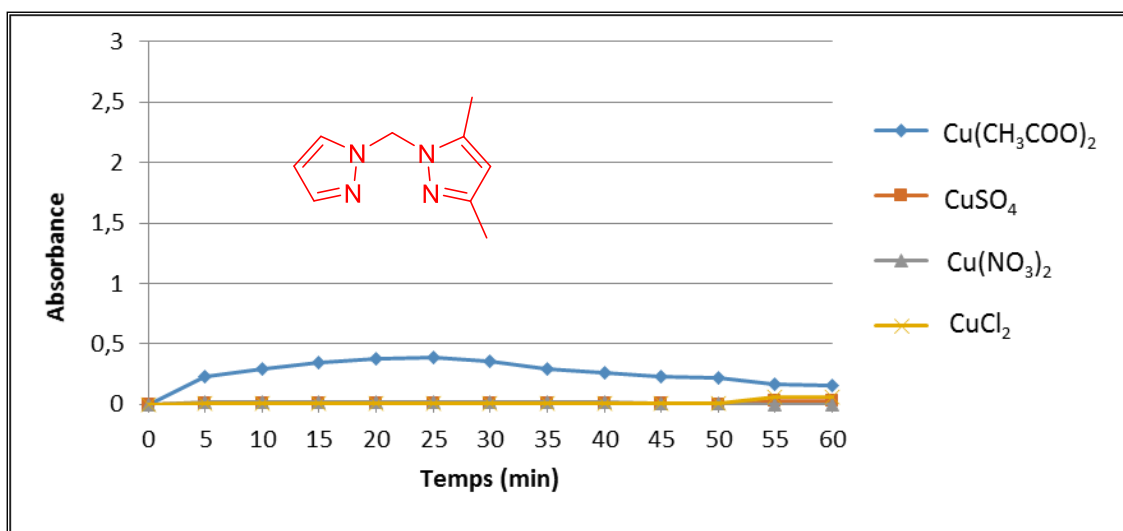
Figure 40 : Oxydation du catéchol en présence du ligand L 9
