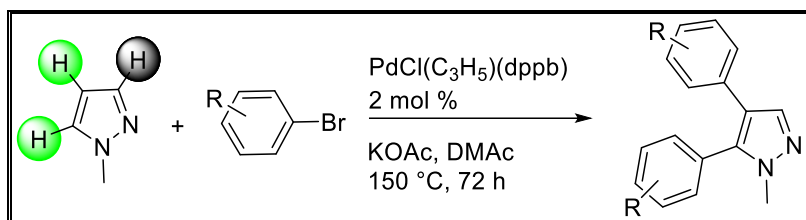
Schéma 27 : Diarylation pallado-catalysée du 1-méthylpyrazole avec des bromures d'aryle
