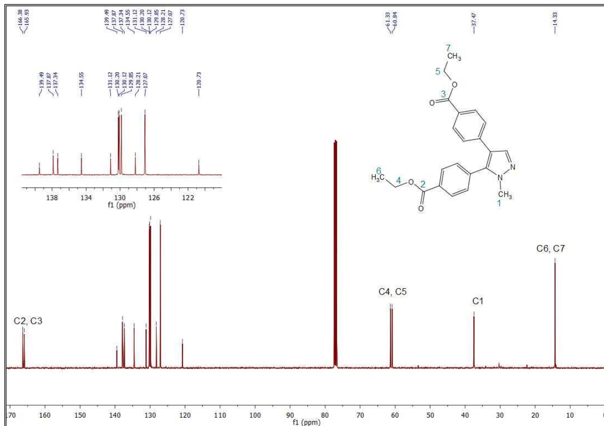
Figure 4 : Spectre RMN 13 C du composé 4 enregistré dans CDCl 3 à 100 MHz
