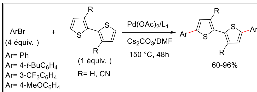
Schéma 17 : Utilisation des bromures d'aryle dans l'arylation directe
