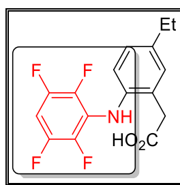
Schéma 39 : Robenacoxib, un dérivé bioactif poly-fluoroaniline.
