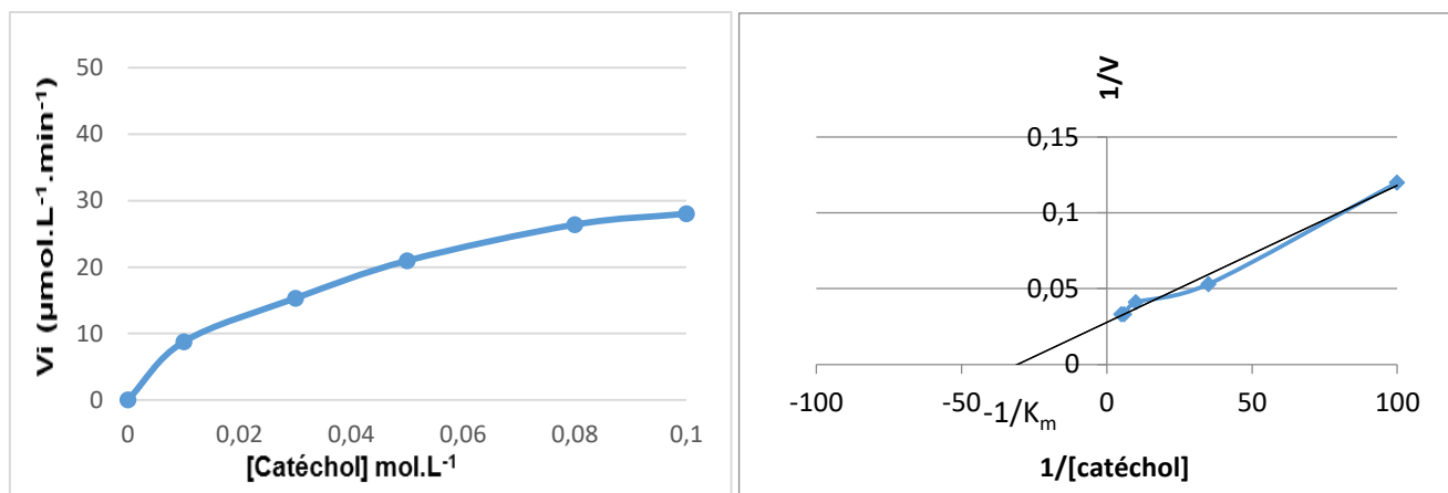
Figure 38 : Représentation graphique des V_i en fonction de la concentration du substrat pour la combinaison L_7/CuSO_4
