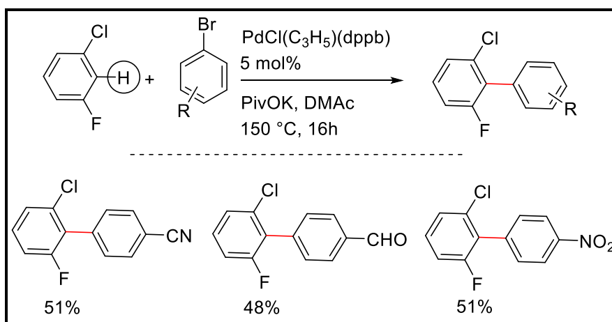
Schéma 10 : Arylation des polyfluorobenzènes
