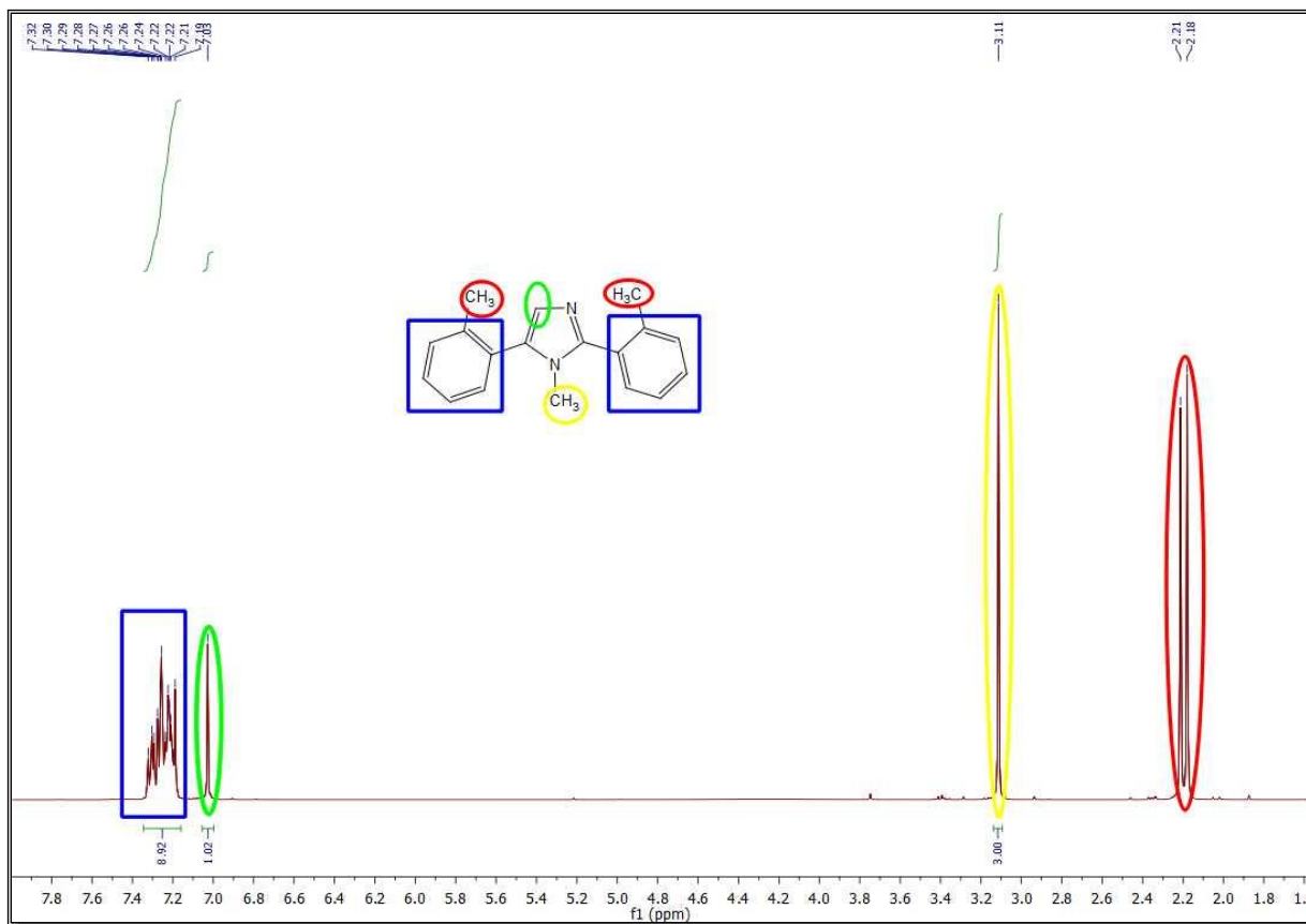
Figure 7 : Spectre RMN ^1\text{H} du composé 44 enregistré dans \text{CDCl}_3 à 400 MHz
