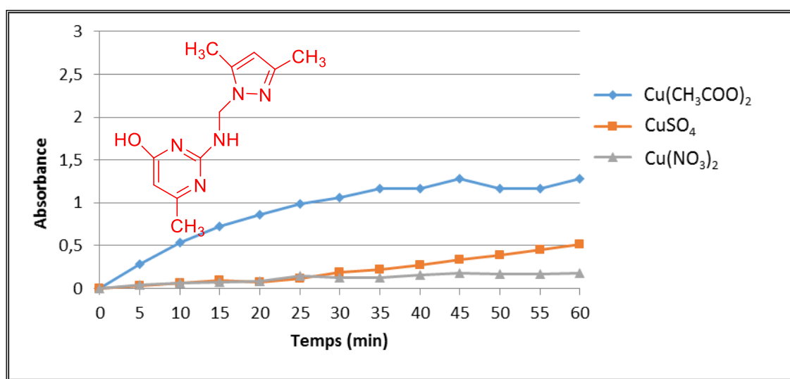
Figure 27 : Oxydation du catéchol en présence du ligand L6 (L/M : 2/1)
