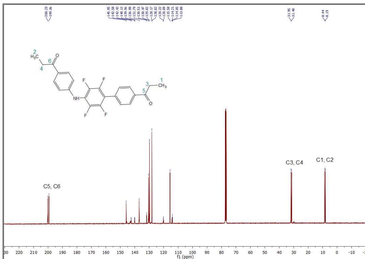
Figure 14 : Spectre RMN 13 C du composé 105 enregistré dans CDCl 3 à 100 MHz
