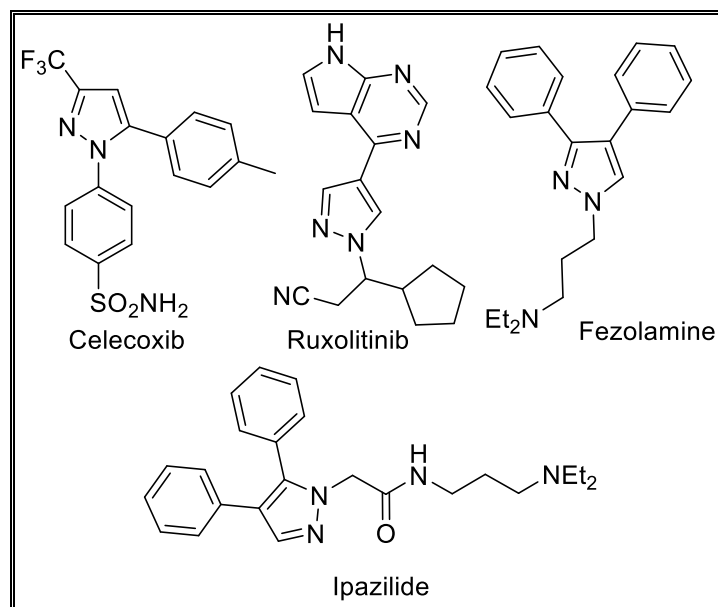
Schéma 20 : Exemples de pyrazoles bioactifs
