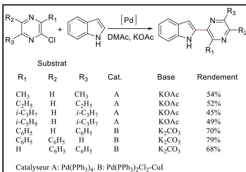
Schéma 2 : Exemple 2 de l'arylation directe Pd-catalysée
