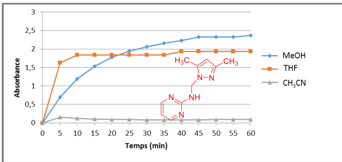
Figure 34 : Oxydation du catéchol en présence de L 7 et Cu(CH 3 COO) 2 dans différents solvants
