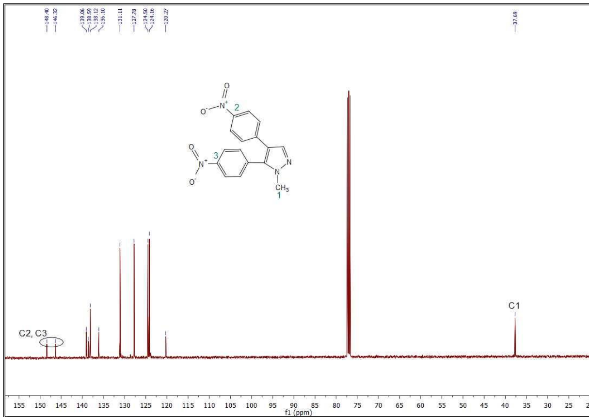
Figure 2 : Spectre RMN ^{13}\text{C} du composé 2 enregistré dans le \text{CDCl}_3 à 100 MHz
