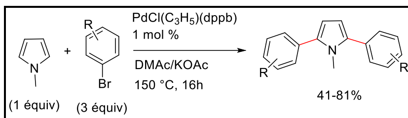
Schéma 18 : Utilisation des bromures d'aryle dans l'arylation directe
