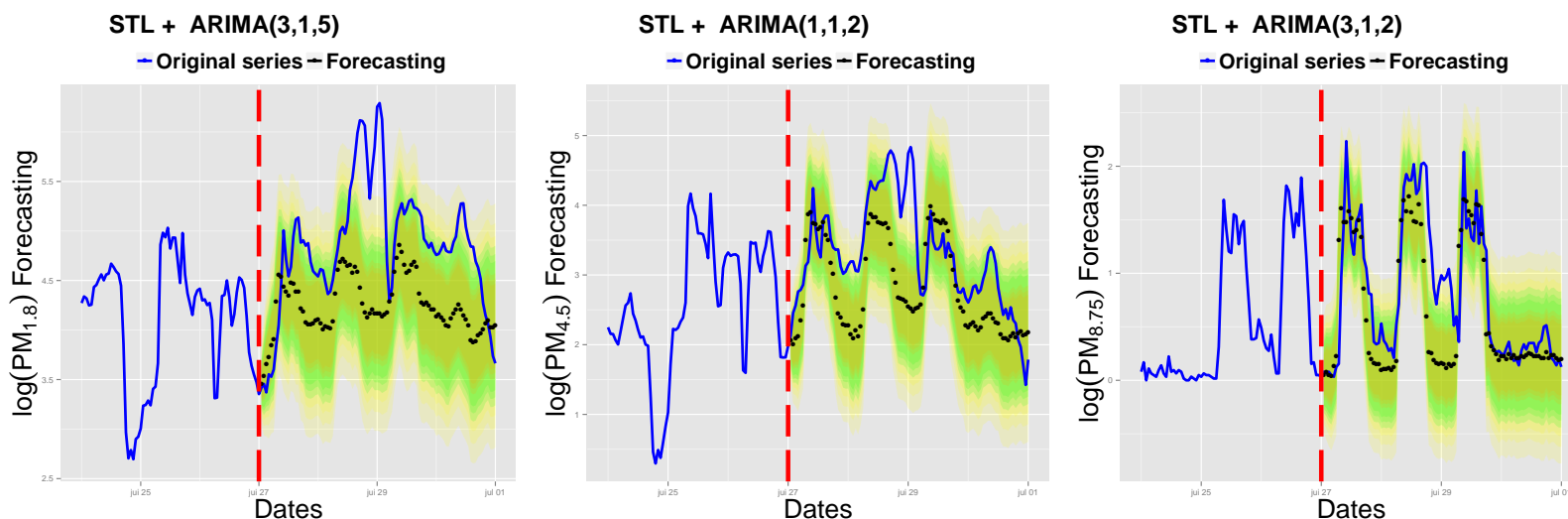
(a) Prévision des concentrations des particules de taille 1.8, 4.5, et 8.75 \mu\text{m} dans l'espace paysager par un modèle de décomposition de type STL combiné avec un modèle ARIMA. Trois jours avant la première prévision sont présentés. La ligne en pointillés rouge sépare la prévision de l'apprentissage.
