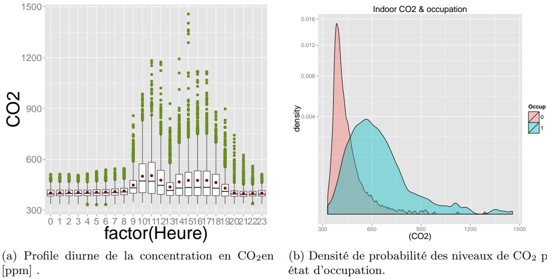
FIGURE 2.5.2 – Niveaux de CO_2 par heure sur une année (a) et densité de probabilité par l'état d'occupation dans un bureau individuel (b). Les points à l'intérieur des boîtes représentent la moyenne de tous les jours par heure et la taille de chaque boîte (coupé par la médiane) renseigne sur le niveau de variabilité diurne (a). L'inoccupation est codée par 0 et l'occupation par 1 (b).
