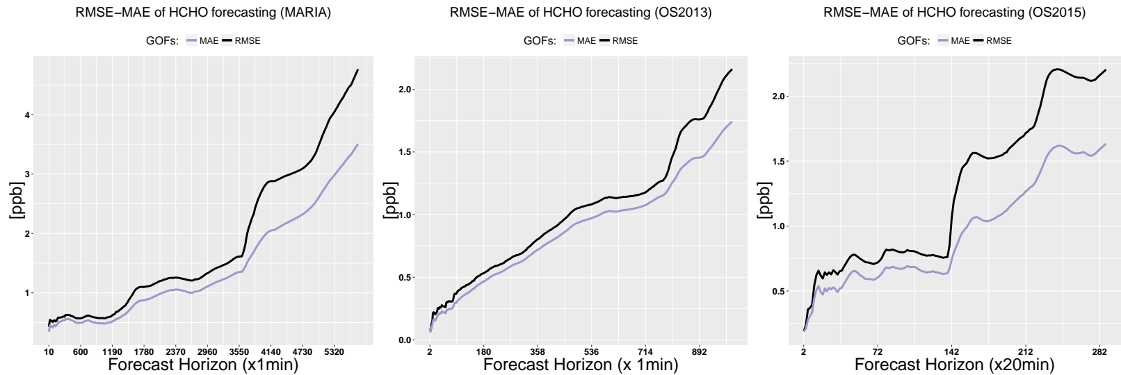
FIGURE 6.5.5 – Prédiction des concentrations du HCHO avec la méthode de HOLT-WINTERS en utilisant les paramètres : \alpha = 0.00033 , \beta^* = 0.003 et \gamma = 0.0095 . dans les environnements suivants : maison expérimentale (MARIA), espace paysager en 2013 (OS2013) et en 2015 (OS2015)
