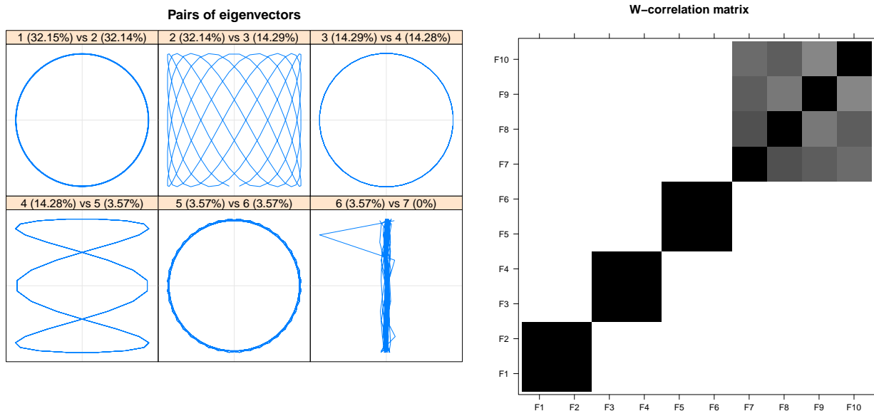
FIGURE 3.6.4 – La procédure SSA sur une série temporelle sinus avec trois fréquences. La taille de la série originale est de 9901 et la reconstitution est faite sur L = 200 . Les T.vertices sont localisés sur les combinaisons de vecteurs propres 1-2, 3-4 et 5-6. Le reconstitution avec 6 composantes représente 100% de la série originale (à gauche). La matrice w – corrélation donne la corrélation entre les 10 différentes composantes séries reconstruites ; la séparabilité est observée à partir de six composantes.
