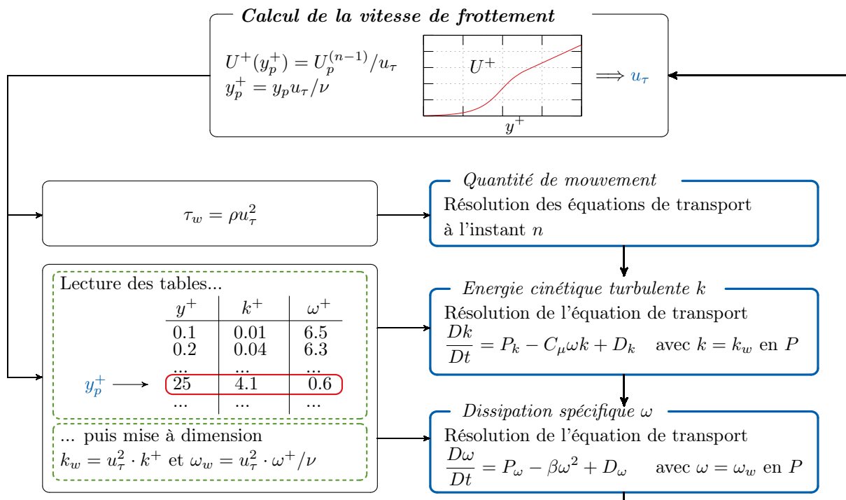
FIGURE 2.17 – Algorithme de paroi de Kalitzin et al. [Kalitzin 2004] pour un modèle k-\omega .
