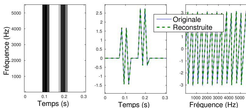
FIGURE 4.12 – Mélange d’impulsions : spectrogramme (gauche) et reconstruction de phase par déroulé linéaire en fonction du temps dans la bande de fréquences à 1800 Hz (centre) et en fonction des fréquences dans la première trame d’attaque (droite).
