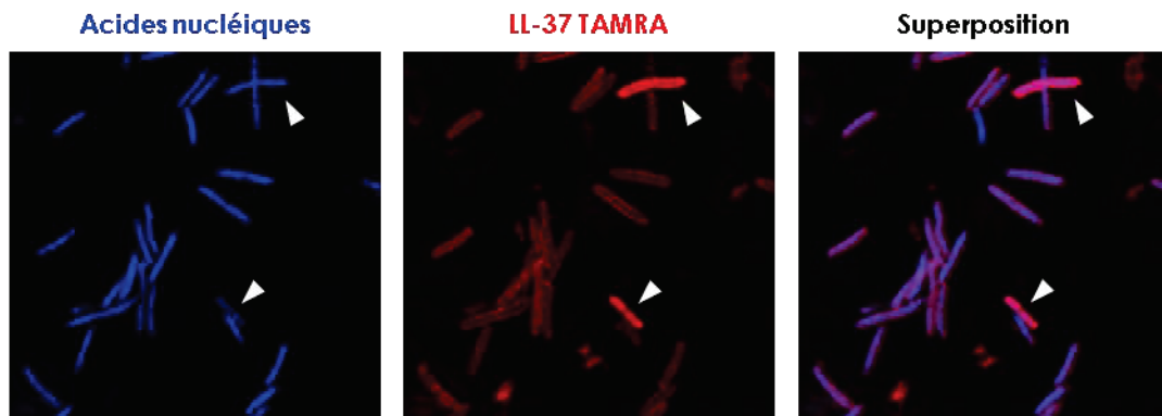
Figure 65. Fixation de LL-37 à la surface de L. pneumophila . La souche L. pneumophila Paris a été incubée avec 10 µg/mL de LL-37 TAMRA (rouge) et 2 µg/mL de DAPI (bleu) pendant 2h. Les bactéries ont ensuite été lavées puis observées par microscopie confocale. Les flèches blanches indiquent les bactéries en cours de division.
