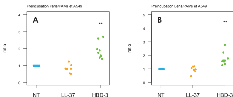
Figure 84. Test d'adhésion de L. pneumophila pré-incubée avec LL-37 ou HBD-3. Les pneumocytes A549 ont été infectés à une MOI=10 pendant 2h avec de la souche Paris (A) ou la souche Lens (B) pré-incubée en absence (NT) ou en présence de 10 µg/mL de LL-37 ou HBD-3. Les cellules ont été lavées puis lysées par choc osmotique. Le lysat a été ensemencé sur milieu BCYE et incubé 72h à 37°C. Les données représentent quatre expériences indépendantes. * p < 0.05 , ** p < 0.01 , *** p < 0.001 .
