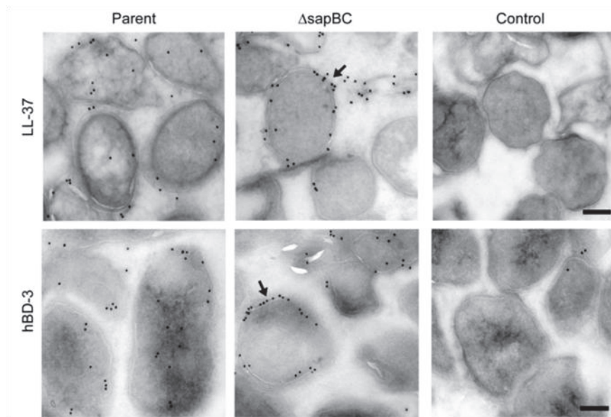
Figure 40. L'import des PAMs vers le cytoplasme requiert le transporteur Sap (Shelton et al. 2011). Les photos de microscopie électronique à transmission ont été réalisées après traitement des souches de Haemophilus influenzae sauvage et \Delta sapBC avec 0,25 \mu g/ml de LL-37 ou 1 \mu g/ml de HBD-3 pendant 30min. Les peptides ont ensuite été marqués par immunogold. Un contrôle a été réalisé avec la souche sauvage non exposée aux peptides.
