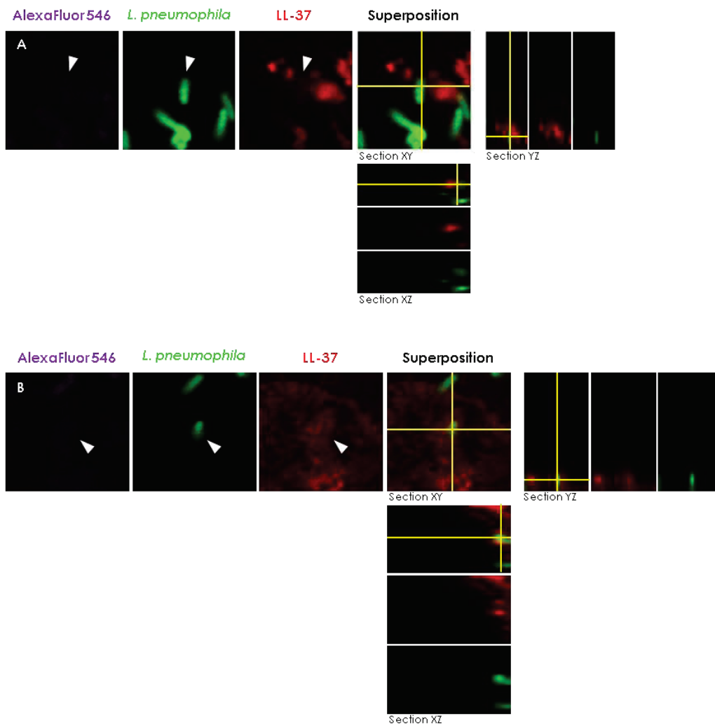
Figure 80. Colocalisation de LL-37 avec L. pneumophila dans les macrophages U937. (A) Les macrophages U937 ont été infectés pendant 2h avec la souche L. pneumophila Paris exprimant la GFP en présence de LL-37 marqué au TAMRA. (B) Les macrophages U937 ont été incubés pendant 2h avec le peptide LL-37 marqué au TAMRA, puis lavés et infectés pendant 2h avec souche L. pneumophila Paris exprimant la GFP. Suite à l'infection, les cellules ont été lavées puis les bactéries extracellulaires ont été marquées à l'aide d'un anticorps primaire anti- Legionella et d'un anticorps secondaire AlexaFluor® 647 afin de les distinguer des bactéries intracellulaires. Les flèches blanches indiquent la présence de bactéries intracellulaires colocalisant avec LL-37. Les droites jaunes représentent les sections orthogonales.
