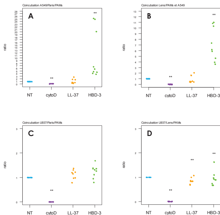
Figure 86. Test d'internalisation de L. pneumophila en coincubation avec LL-37 ou HBD-3. Les pneumocytes A549 (A et B) ou les macrophages U937 (C et D) ont été infectés pendant 2h avec de la souche Paris (A et C) ou la souche Lens (B et D) à une MOI=10 en absence (NT) ou en présence de 10 µg/mL de LL-37 ou HBD-3. Les cellules ont été lavées, traitées pendant 2h avec 200 µg/mL de Gentamycine puis lavées. Les cellules ont été lysées par choc osmotique et le lysat a été ensemencé sur milieu BCYE et incubé 72h à 37°C. Les données représentent trois expériences indépendantes. * p < 0.05 , ** p < 0.01 , *** p < 0.001 .
