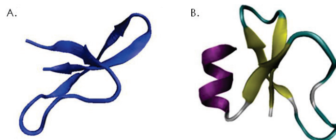
Figure 44. Structure cristallographique des \alpha - et \beta -défensines (Mattar et al. 2016). (A) Structure de l' \alpha -défensine 1 humaine (HNP-1), (B) Structure de la \beta -défensine 1 humaine (HBD-1).
