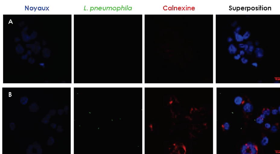
Figure 89. Immunomarquage de la calnexine dans les macrophages U937. Les macrophages U937 ont été incubés pendant 4h en absence (A) ou en présence (B) de la souche L. pneumophila exprimant la GFP. Les cellules ont ensuite été lavées puis la calnexine a été immunomarkuée (rouge) et le noyau des cellules a été marqué au DAPI (bleu).
