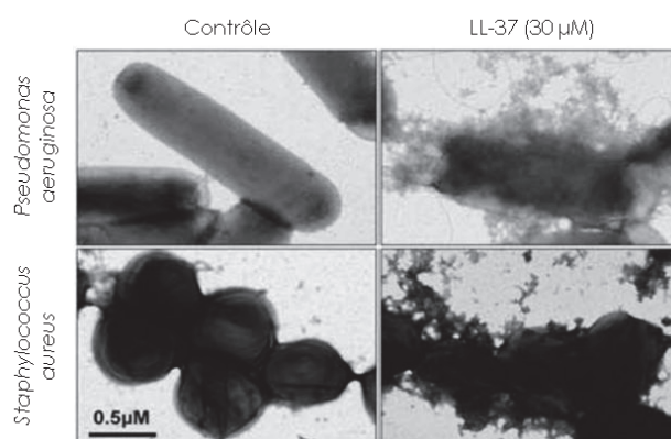
Figure 94. Effet de LL-37 sur la morphologie de P. aeruginosa et S. aureus (Papareddy et al. 2012).
