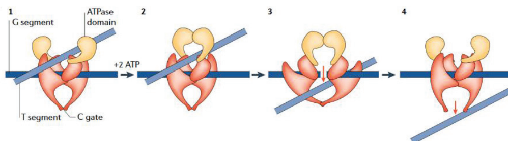
Figure 8. Schéma du mécanisme d'action des topoisomérases de type II (Cozzarelli et al. 2006). (1) La topoisomérase de type II (en rouge et jaune) se fixe au segment d'ADN G (bleu foncé) et au segment T (bleu clair), (2) Deux molécules d'ATP sont hydrolysées, puis le domaine ATPase (en jaune) se ferme, (3) Le segment G est clivé et le segment T est transporté de la première cavité à la seconde cavité à travers le segment G, (4) Le fragment T est libéré au niveau du domaine C.
