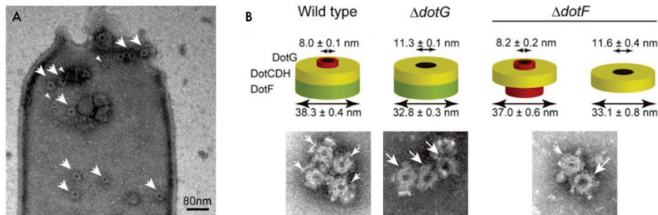
Figure 12. Structure du core du système de sécrétion de type IV Dot/Icm de L. pneumophila (Kubori et al. 2014). (A) Photo de microscopie électronique à transmission de la surface de L. pneumophila . Les grandes et les petites flèches indiquent les cores de grande et de petite taille, respectivement. (B) Schémas du core du système de sécrétion de type IV Dot/Icm observé chez une souche de L. pneumophila sauvage, \Delta dotG ou \Delta dotF . La moyenne des diamètres interne et externe du core, ainsi qu'une photo de microscopie électronique à transmission de la surface bactérienne sont associées à chaque type de structure. Les petites et les grandes flèches indiquent les pores de petit et de grand diamètre, respectivement.
