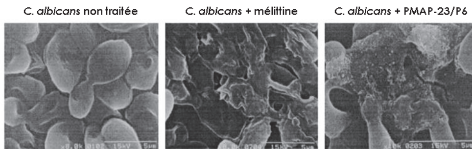
Figure 31. Le traitement avec le la mélittine ou le PMAP-23/P6 induit des changements morphologiques chez C. albicans (d'après Lee et al. 2002). Les photos de microscopie électronique à balayage ont été réalisées après traitement des levures avec 12,5 µM de mélittine ou 12,5 µM pendant 4h à 28°C.
