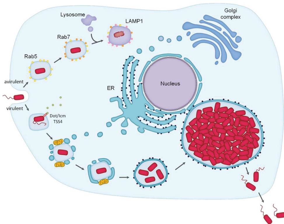
Figure 9. Cycle infectieux de Legionella pneumophila . L. pneumophila est internalisée par la cellule hôte eucaryote dans un phagosome. Les bactéries virulentes bloquent la voie de maturation du phagosome et injectent des effecteurs via leur système de sécrétion de type 4 (TSS4) pour créer une vacuole de réplication (LCV). L. pneumophila recrute rapidement des mitochondries et des vésicules de réticulum endoplasmique (ER) à la surface de sa LCV, puis des ribosomes avant d'entamer sa réplication. Une fois les ressources de la cellule hôte épuisées, les bactéries lyse leur LCV et la cellule pour être libérées dans le milieu extracellulaire afin d'infecter les cellules avoisinantes.
