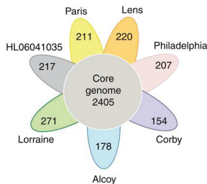
Figure 3. Schéma de la composition du génome de 7 souches de L. pneumophila (Gomez-Valero & Buchrieser 2013). Chaque couleur de pétale représente le génome d'une souche de L. pneumophila . Le nombre au centre du diagramme représente les gènes orthologues partagés par tous les génomes. Le nombre inscrit dans chacun des pétales correspond aux gènes spécifiques à chaque génome.
