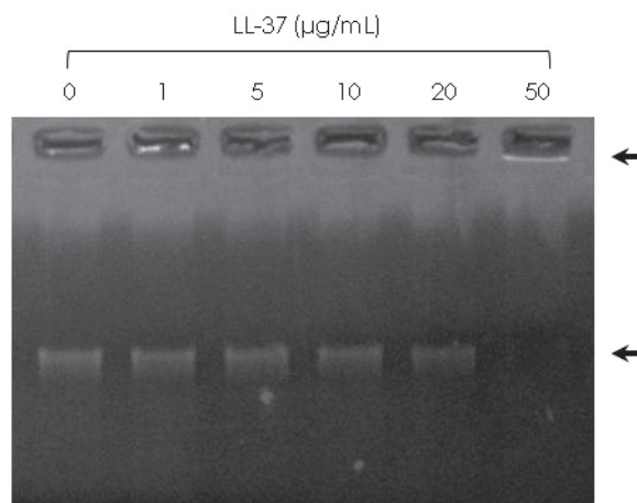
Figure 67. Gel de retard de migration électrophorétique de l'ADN de L. pneumophila . L'interaction ADN/LL-37 a été évaluée par l'effet inhibiteur du peptide sur la migration de l'ADN. Une quantité fixe d'ADN génomique (250 ng) de L. pneumophila Paris a été incubée avec différentes concentrations de LL-37 (de 0 à 50 µg/mL) pendant 1h à 37°C. Le mélange a ensuite été déposé sur un gel d'agarose à 1% afin d'évaluer la migration de l'ADN par électrophorèse. La concentration de peptide est indiquée au dessus des puits de dépôt. Les flèches indiquent la présence de bandes correspondant à l'ADN génomique.
