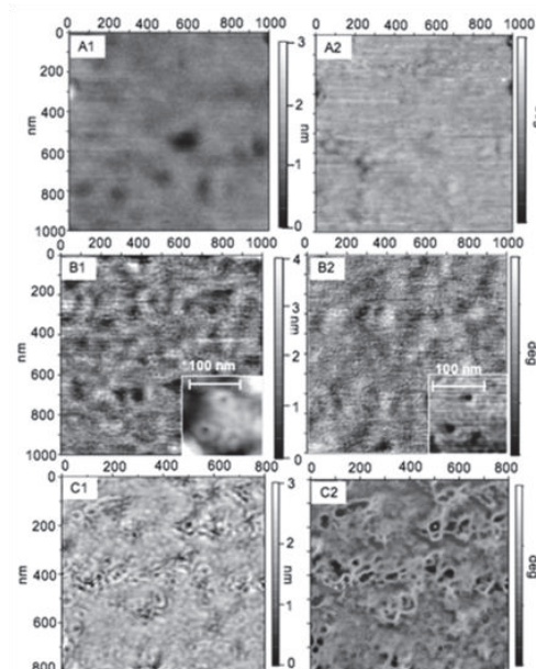
Figure 45. Effet des peptides LL-37 et mmuRL-37 sur des liposomes composés de phospholipides anioniques (Morgera et al. 2009). Les photos de microscopie à force atomique ont été réalisées après traitement des liposomes avec 20 \mu M de peptides pendant 1h. Les images topographiques (A1, B1 et C1) et à contraste de phase (A2, B2 et C2) des liposomes ont été non traitées (A1 et A2) ou traitées avec LL-37 (B1 et B2) ou mmuRL-37 (C1 et C2).
