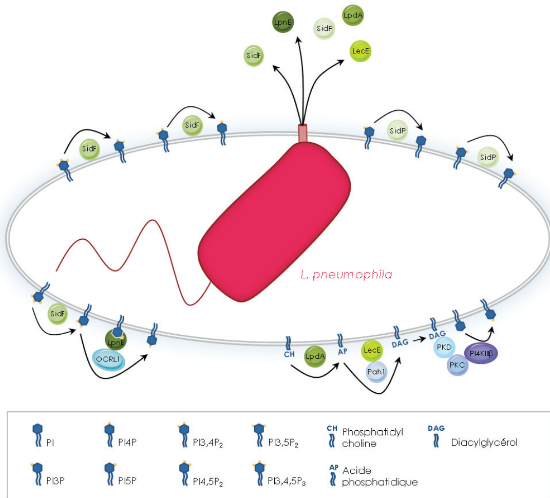
Figure 17. Modification des phosphoinositides de la LCV de L. pneumophila . Depuis sa vacuole, L. pneumophila sécrète des effecteurs (vert), qui en combinaison avec certaines protéines de l'hôte (bleu) sont impliqués dans le remodelage de lipides de la LCV : SidF, SidP, LpnE, LpdA et LecE. L'effecteur SidF hydrolyse le phosphatidylinositol-3,4,5-trisphosphate (PI3,4,5P 3 ) et le phosphatidylinositol-3,4-bisphosphate (PI3,4P 2 ) en phosphatidylinositol-4,5-bisphosphate (PI4,5P 2 ) et en phosphatidylinositol-4-phosphate (PI4P), respectivement. L'effecteur SidP hydrolyse quant à lui le phosphatidylinositol-3-phosphate (PI3P) et le phosphatidylinositol-3,5-bisphosphate (PI3,5P 2 ) en PI et en phosphatidylinositol-5-phosphate (PI5P), respectivement. La protéine OCRL1 recrutée par l'effecteur LpnE hydrolyse le PI4,5P 2 produit par SidF en PI4P. L'effecteur LpdA, ancré dans la LCV, hydrolyse la phosphatidylcholine (PC) en acide phosphatidique (AP), lui-même converti en diacylglycérol (DAG) par l'action combinée de l'effecteur LecE et de la phosphatase eucaryote Pah1. Le DAG recrute ensuite la protéine kinase D (PKD) et son activateur, la protéine kinase C (PKC). La PKC activée recrute à son tour la phosphatidylinositol 4-kinase (PI4K) IIIβ (PI4KIIIβ), qui phosphoryle le PI afin de produire du PI4P à la surface de la LCV.
