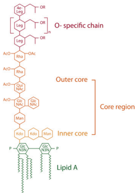
Figure 5. Structure du LPS de L. pneumophila (Shevchuk et al. 2011). Le LPS de L. pneumophila comprend différentes régions : la chaîne O (rouge), le core comprenant le core externe (orange) et le core interne (jaune), ainsi que le lipide A (vert). Leg : dérivé de l'acide légionaminique ; 4e-Leg : dérivé de l'acide 4-épilégionaminique ; Rha : rhamnose ; Man : mannose ; QuiNAc : acétylquinovosamine ; GlcNAc : acétylglucosamine ; Kdo : acide 3-deoxy-d-manno-oct-2-ulosonique ; P : phosphate ; OAc : O-acétyle.
