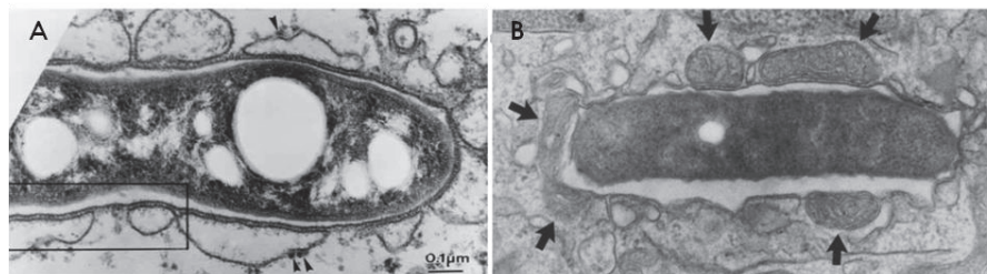
Figure 10. Recrutement des vésicules de réticulum endoplasmique (RE) et de mitochondries sur la LCV (Tilney et al. 2001 ; Horwitz 1983). (A) La photo de microscopie électronique a été réalisée après 15 min d'infection de macrophages par L. pneumophila . Le cliché montre une légionelle dans un phagosome, entouré de vésicules de RE. Les flèches indiquent la présence de ribosomes attachés aux vésicules de RE. (B) La photo de microscopie électronique a été réalisée après 1h d'infection de monocytes par L. pneumophila . Le cliché montre une légionelle dans un phagosome entouré de vésicules et de 5 mitochondries (flèches).
