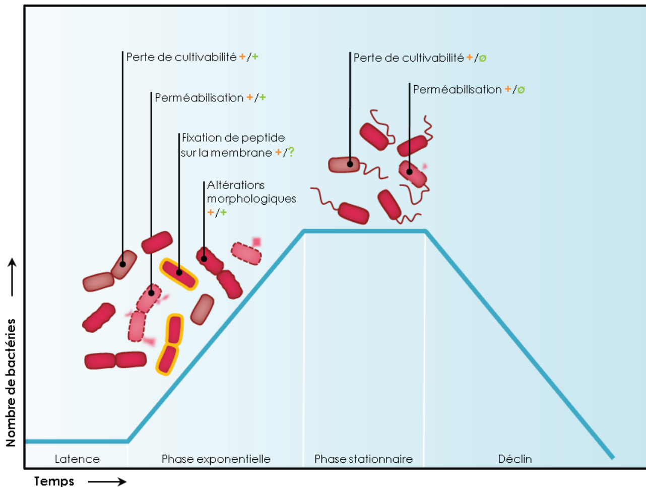
Figure 90. Bilan des activités antimicrobiennes directes des peptides LL-37 et HBD-3 contre L. pneumophila en milieu extracellulaire.
