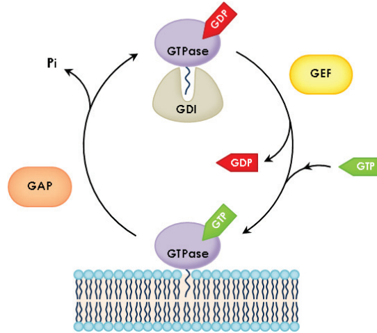
Figure 18. Schéma de régulation des petites GTPases. Les petites GTPases alternent entre une forme membranaire active liée au GTP et une forme cytoplasmique inactive liée au GDP. Certaines formes de GTPases sont liées à des protéines GDI ( Guanine Dissociation Inhibitor ) qui les maintiennent sous forme inactives. Les GTPases sont activées par des protéines GEF ( Guanine nucleotide Exchange Factor ) par échange du GDP par une molécule de GTP. Les protéines GAP ( GTPase Activating Protein ) inactivent les GTPases par hydrolyse du GTP.
