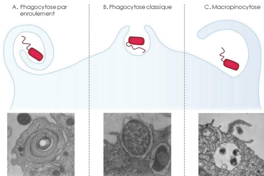
Figure 15. Schéma des différents modes d'internalisation des bactéries (d'après Horwitz 1984 et Schneider et al. 2007). (A) Phagocytose par enroulement. Photo : L. pneumophila phagocytée par un monocyte. (B) Phagocytose classique. Photo : L. pneumophila phagocytée par un monocyte. (C) Macropinocytose. Photo : Afipia felis phagocytée par un monocyte.
