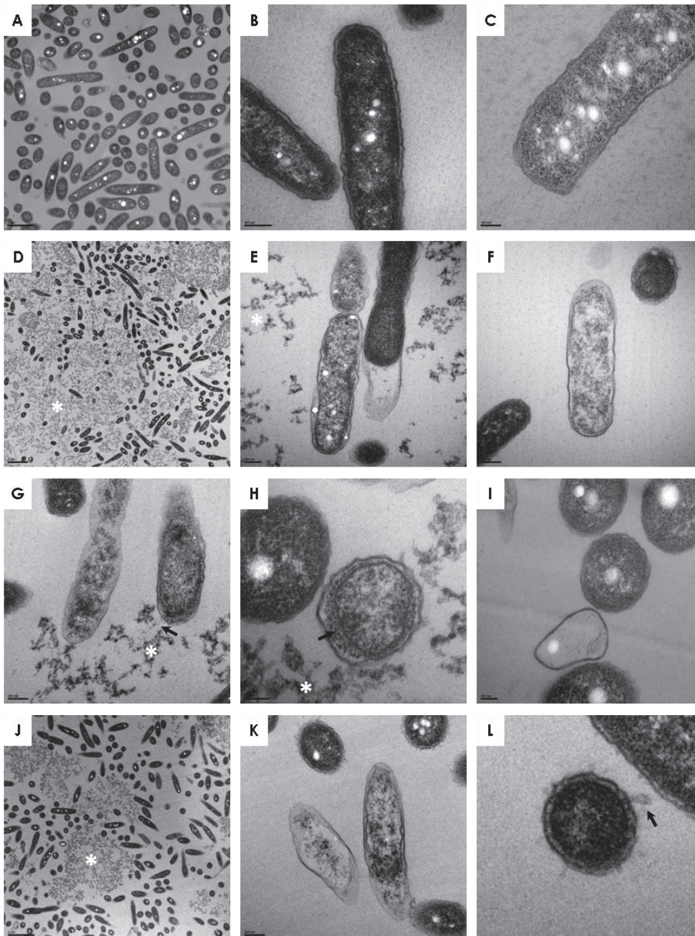
Figure 68. Effet de LL-37 et HBD-3 sur l'ultrastructure de L. pneumophila . La souche Paris WT cultivée en phase exponentielle a été incubée en absence (A-C) ou en présence des peptides LL-37 (10 µg/mL) (D-I) ou HBD-3 (10 µg/mL) (J-L) pendant 2h à 37°C sous agitation. Les bactéries ont été lavées, fixées puis marquées et observées par microscopie électronique à transmission. Les astérisques blancs indiquent la présence de contenu cytoplasmique hors des bactéries.
