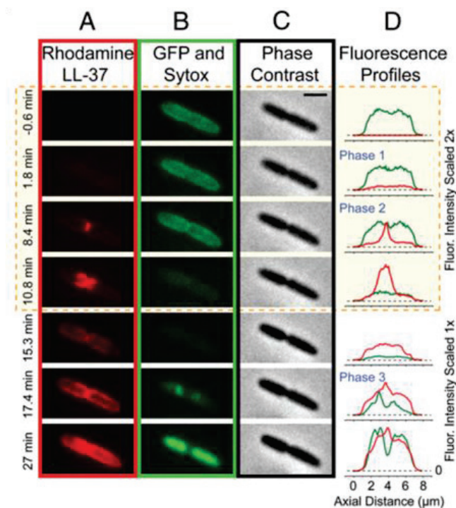
Figure 93. Cinétique de fixation de LL-37 marqué à la rhodamine sur E. coli (Sochacki et al. 2011). Les bactéries expriment une GFP périplasmique et le milieu contient le marqueur d'ADN Sytox Green. Chaque image est issue d'une même vidéo au temps indiqué à gauche. (A) LL-37 marqué à la rhodamine, (B) GFP périplasmique puis marqueur d'ADN Sytox Green, (C) contraste de phase et (D) profils d'intensité des signaux de fluorescence rouge et verts.
