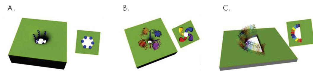
Figure 28. Représentation schématique des différents types de pores toriques (Gilbert et al. 2014). (A) et (B) Pores toriques de type « matrice » ; (C) Pore torique de type « arc ».
