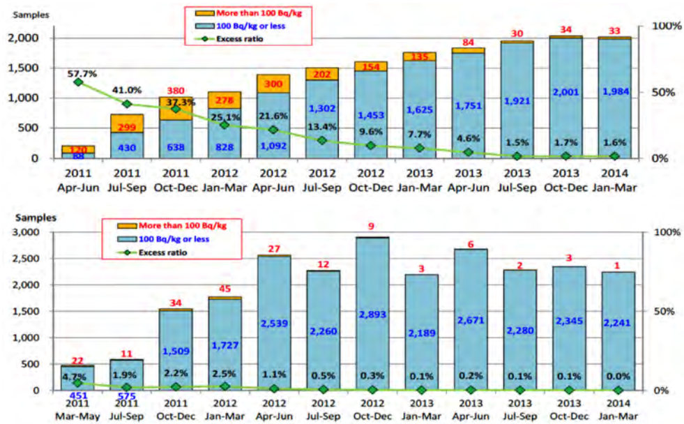
FIGURE 3.7 – Les proportions relatives du nombre de poissons dont la concentration est supérieure à la norme de consommation et de commercialisation ( 100 \text{ Bq kg}^{-1} \text{ ww} ). En haut les données relatives à la préfecture de Fukushima, en bas celles relatives aux préfectures autre que Fukushima (Source : MEXT [2014])
