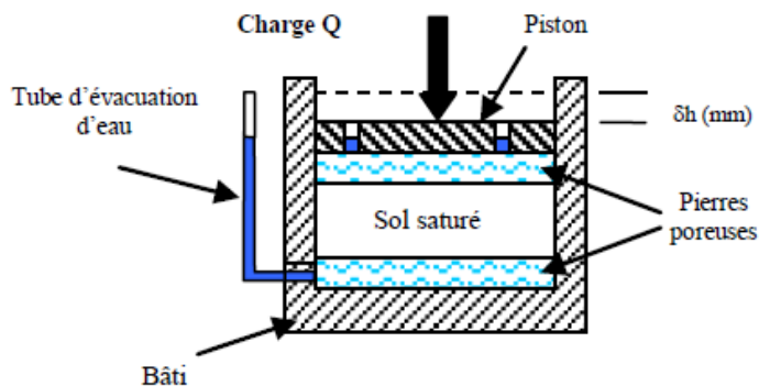
Figure 2-20: Cellule œdométrique
