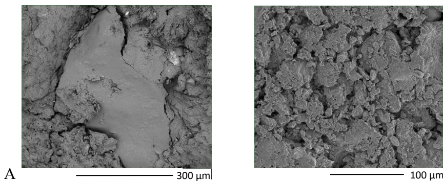
Figure 4-23: Images MEB de AT traité à 6%
