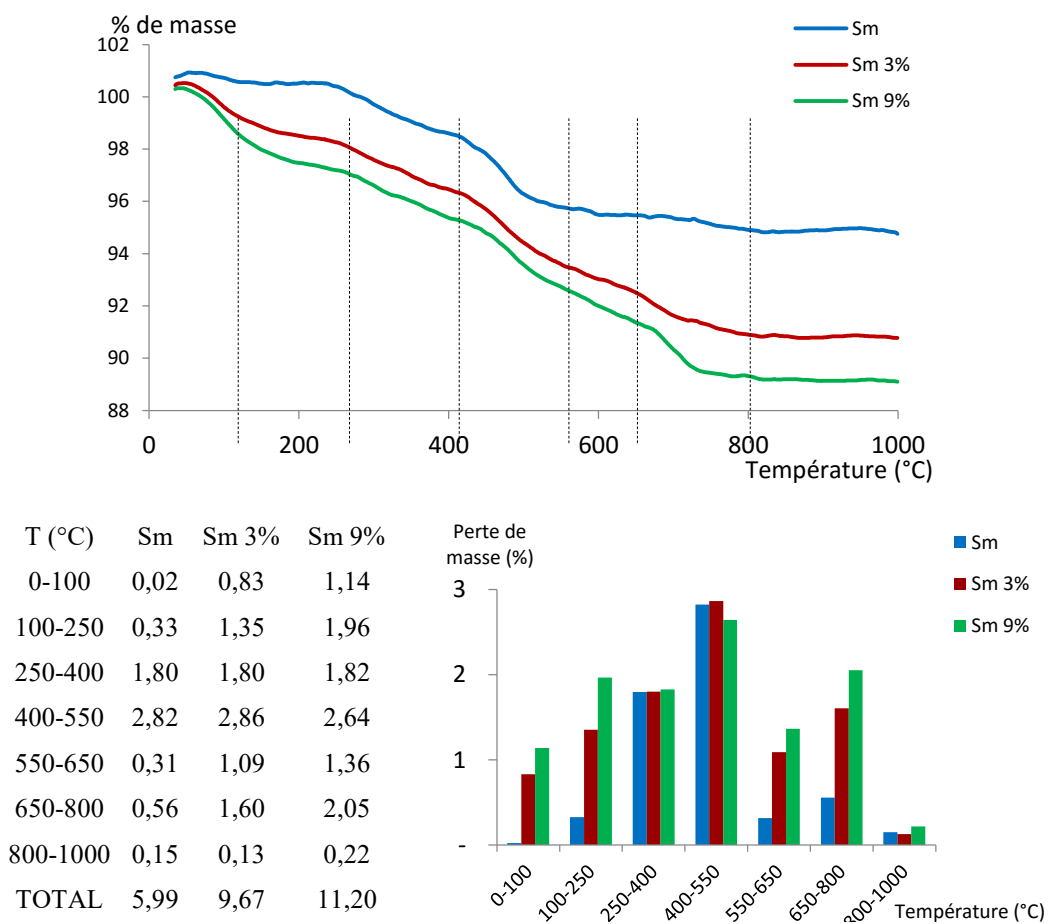
Figure 4-15: Evolution de la perte de masse de Sm
