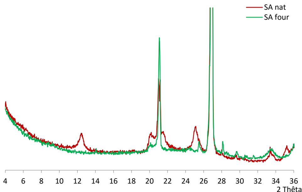
Figure 3-30 : DRX sur lames orientées (naturel – four à 550°C) de SA
