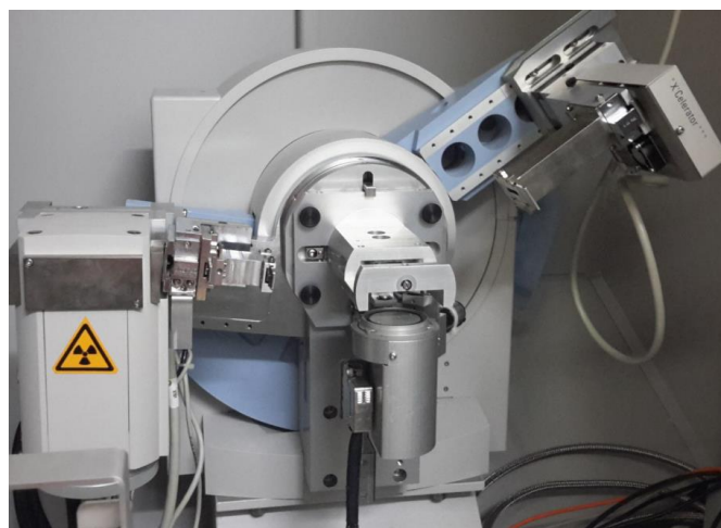
Figure 2-12: Diffractomètre utilisé
