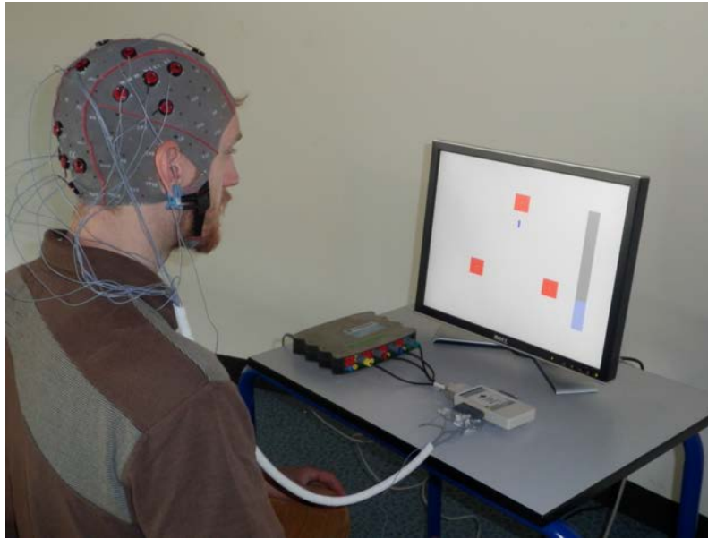
Figure 1: Utilisateur d'une ICO basée sur SSVEP, portant un casque EEG, et regardant un stimulus clignotant (ici des carrés rouges).
