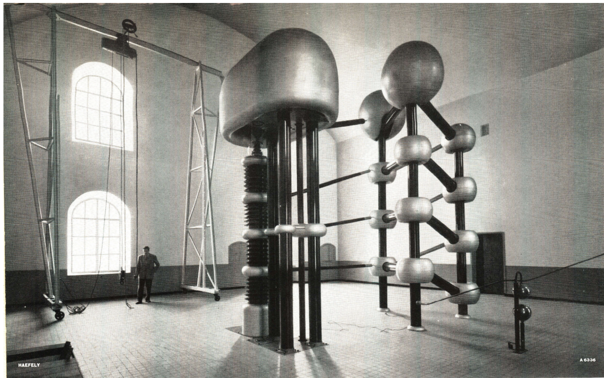
Figure 30. La partie haute du générateur de Cockroft-Walton, installé dans le bâtiment A du fort de la Vitriolerie, telle qu'elle apparaît dans une brochure publicitaire du fabricant HAEFELY que nous avons pu consulter.
