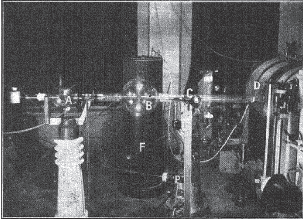
Fig. 1. — Dispositif monté par Jean Thibaud pour reproduire les expériences de Cockroft et Walton sur la désintégration du lithium par un flux de protons.
