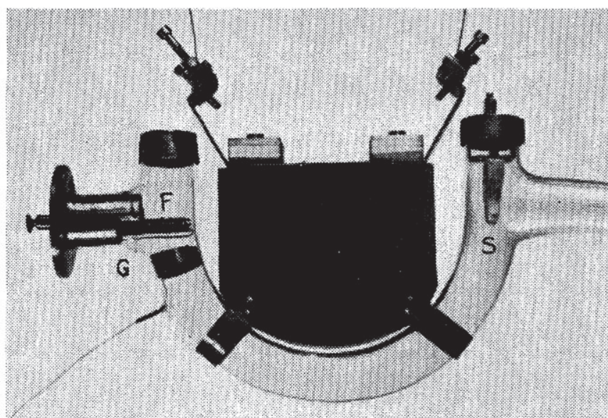
Figure 17. Photographie du dispositif utilisé par Thibaud en 1933 pour l'étude des positrons 169 .
