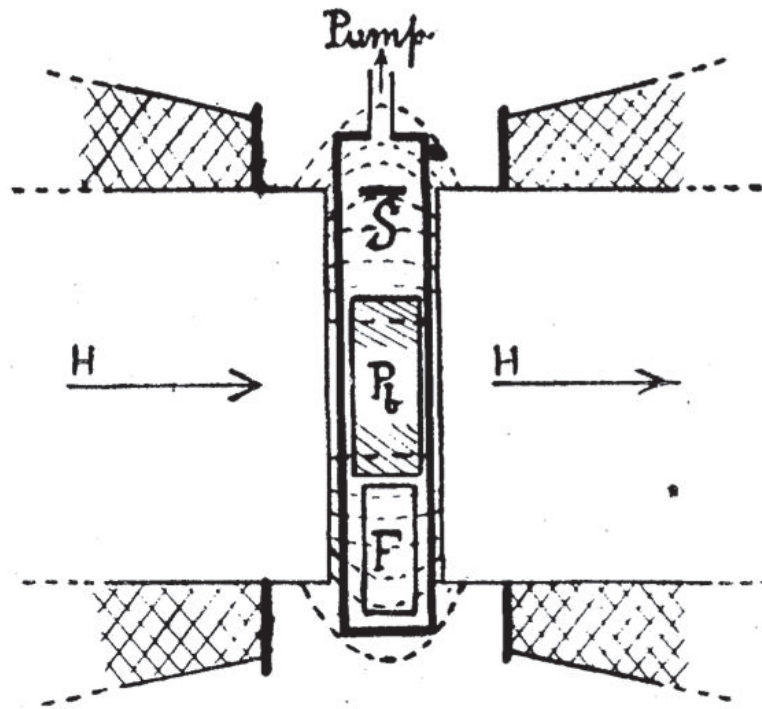
FIG. 1. Longitudinal section of apparatus.
