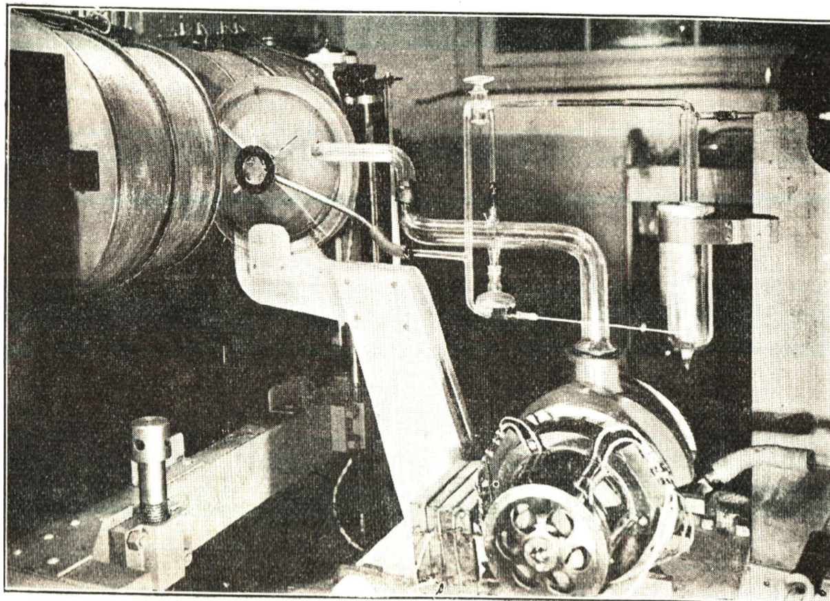
Figure 12. Dispositif générateur d'ions rapides par accélération en haute fréquence avec électroaimant. Comptes rendus Congrès de Paris.
