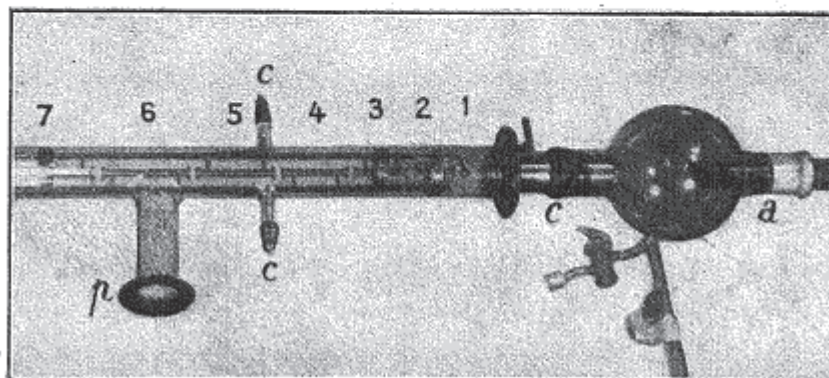
Figure 10. Schéma du dispositif Thibaud d'accélération des ions positifs par tension variable 118 .
