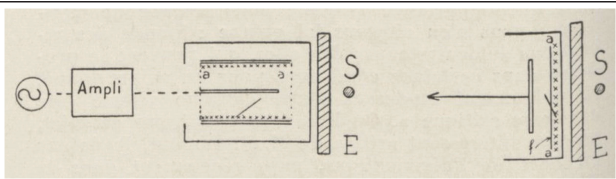
Figure 18. Schéma du dispositif utilisé par J. Thibaud et A. Moussa pour l'étude des produits de fission 205 .
