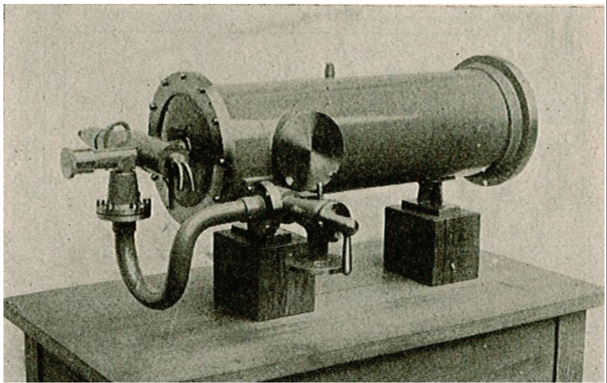
Figure 4. Spectrographe à diffraction de rayons X. Thibaud, J. [1942]. Vie et transmutations des atomes . Paris, France : A. Michel, 1942, planche V.
