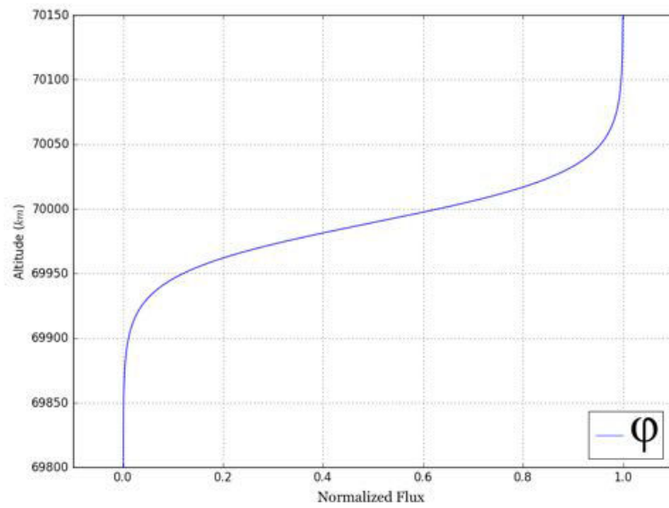
(c) Le flux normalisé \phi (Eq. 3.22) correspondant à la dispersion géométrique des rayons lumineux par la réfraction différentielle.
