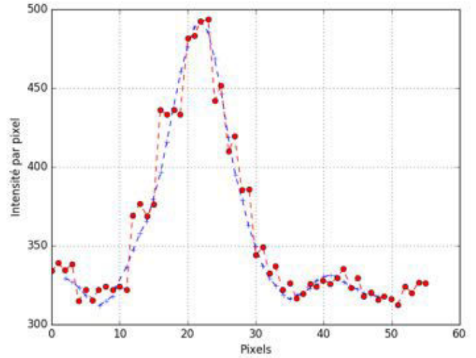
(b) Extraction du flux et interpolation (stade 2 et 3). Latitude +80^{\circ}_W pour f = 0.5 . Un point représente 1/4 de pixel.
