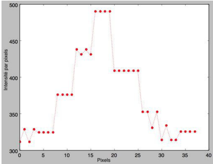
(a) Extraction du flux de manière radiale sans interpolation (stade 1). Latitude +80^{\circ}_W pour f = 0.5 . Un point représente 1/4 de pixel.
