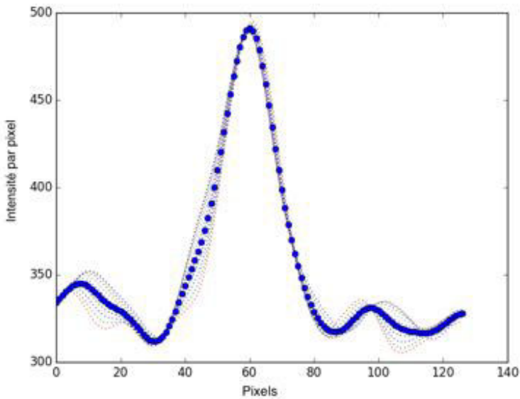
(c) Extraction du flux (stade 4). Latitude +80^{\circ}_W pour f = 0.5 , 1 point pour 1/10 de pixel.
