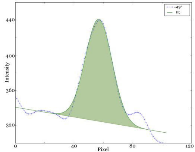
(d) Extraction du flux (stade 4). Latitude +49^{\circ}_W pour f = 0.5 .
