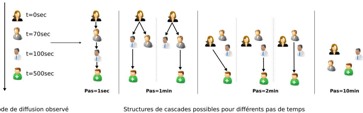
FIGURE 3.2 – Importance du choix du pas de temps
