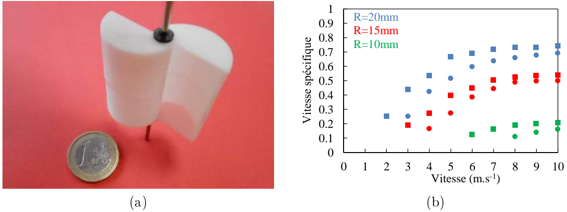
FIGURE 3.22 – (a) Exemple de micro-turbines Savonius. (b) Evolution de la vitesse spécifique à vide (couple de frottement du roulement uniquement) de plusieurs micro-turbines Savonius, voir section 4.3.2.1.
