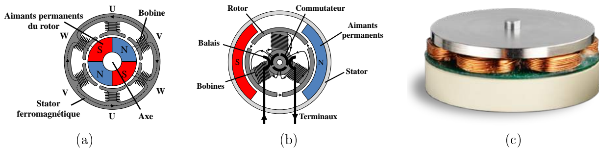
FIGURE 1.8 – (a) Servomoteur DC sans balai   aimants permanents mobiles (4 p les au rotor et 6 p les au stator). (b) Servomoteur DC   balais   aimants permanents fixes (3 p les au rotor et 2 p les au stator). (c) Moteur utilis  par [FMSS10].
