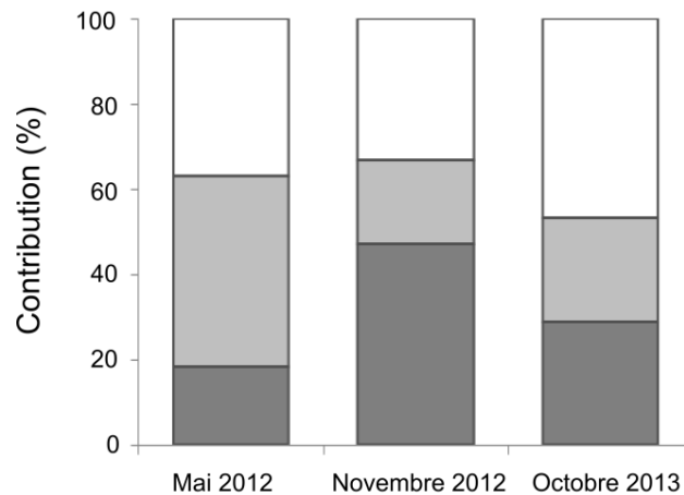
Figure 3.5. Proportion relative des 3 taxons de phytoplancton (-●-cyanobactéries; -●-picoeucaryotes; -●-nanophytoplancton) en terme de biomasse carbonée dans le milieu pour les 3 dates d'expérience.
