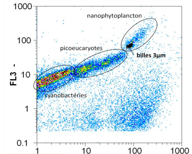
Fig. 3.4. Cytogramme représentant les 3 taxons de phytoplancton identifiés par cytométrie en flux. FL3 correspond à la fluorescence rouge (chlorophylle) et FSC à la taille des particules. Les billes permettent de situer les tailles des différentes particules.
