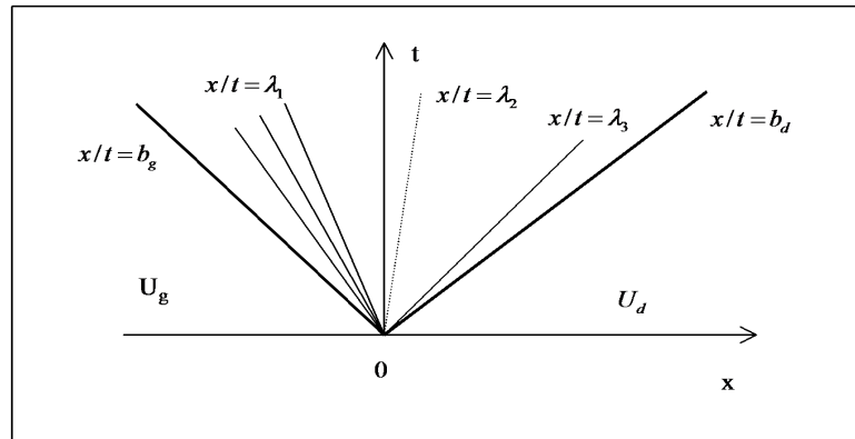
FIGURE 6.5 – Solution approchée du problème de Riemann
