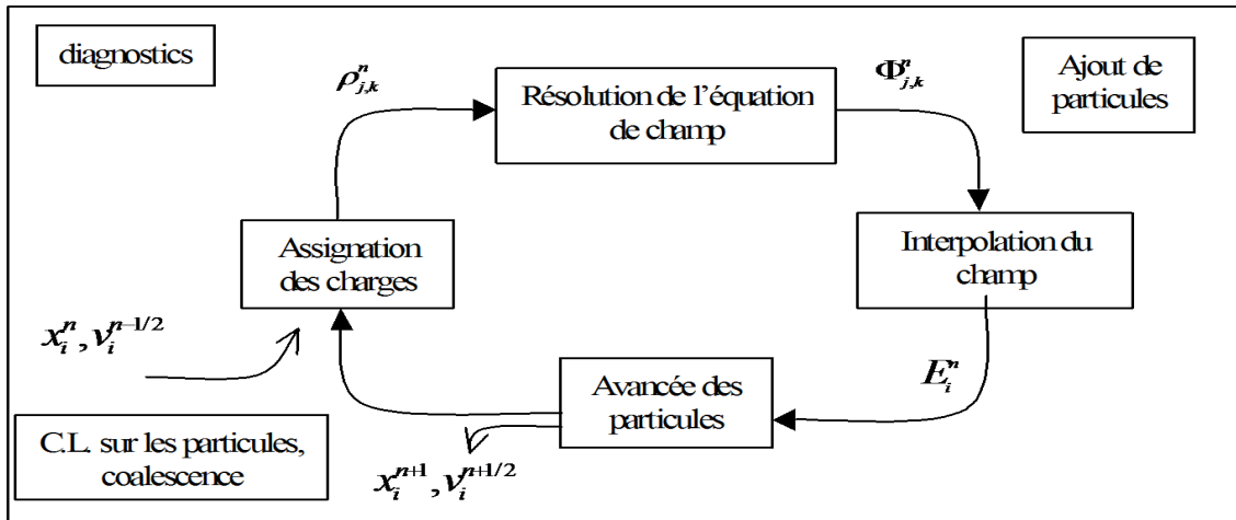
FIGURE 3.2 – Cycle d'une méthode PIC sur une itération.
