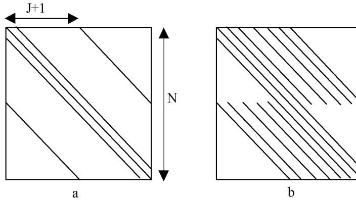
FIGURE 3.7 – Profil des matrices A (a) et L (b).
