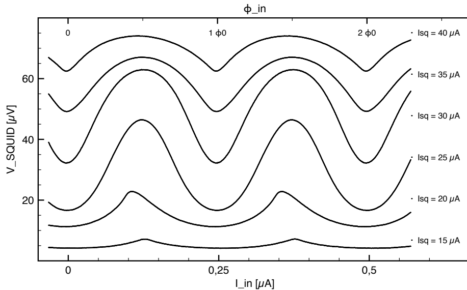
FIGURE 6.5 – Caractéristique de tension d'un SQUID V_{SQUID} en fonction d'un flux magnétique extérieur \phi_{in} (abscisse du haut) et du courant à l'origine de ce flux I_{in} (abscisse du bas). Les différentes lignes sont obtenues pour différents courants de polarisation I_{sq} . On remarque le comportement approximativement sinusoïdal et la périodicité en \phi_0 , le minimum atteint pour des valeurs entières de \phi_0 et le maximum pour des demi-entiers de \phi_0 .
