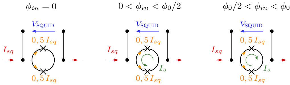
FIGURE 6.3 – Répartition du courant dans les jonctions Josephson d'un SQUID traversé par un courant de polarisation I_{sq} et auquel on applique un flux magnétique extérieur \phi_{in} .
