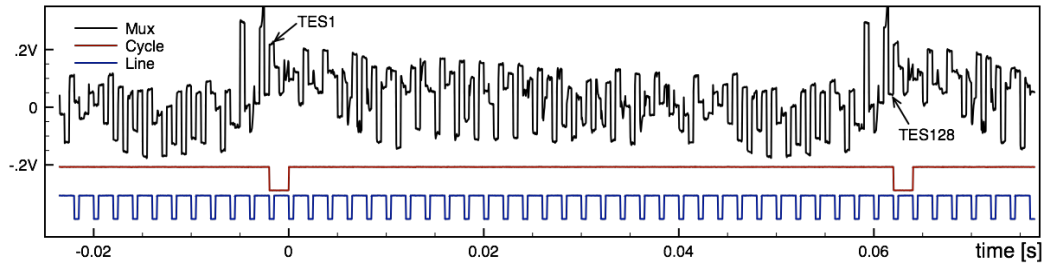
FIGURE 6.24 – En noir, signal unique multiplexé temporellement à partir des signaux issus de 128 TESs/SQUIDS. Les deux signaux en dessous sont synchronisés et générés simultanément pour repérer la fin de la lecture complète d'un cycle de 128 TESs (en rouge) et la lecture d'une ligne de quatre SQUIDS (en bleu). Les excursions entre les différents créneaux temporels du signal multiplexé témoignent d'une différence d' offset entre les pixels, bien qu'elle soit déjà en partie compensée. La fréquence d'échantillonnage est de l'ordre de 15 Hz et la fréquence de multiplexage de 2 kHz.
