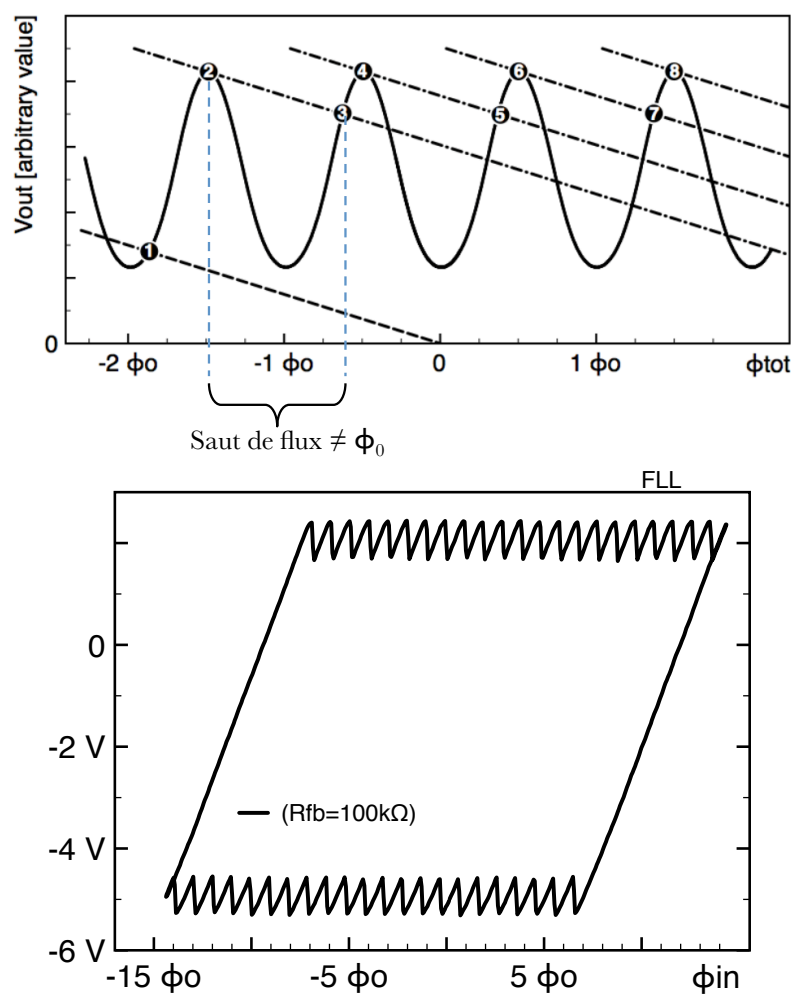
FIGURE 6.10 – Haut : Évolution schématique de la droite de charge traduisant la réponse de la FLL générée par l'augmentation linéaire d'un flux extérieur \phi_{in} (fonction rampe). La FLL se situe initialement sur un point de fonctionnement stable (en 1) par rapport à la fonction de transfert amplifiée du SQUID en boucle ouverte V_{out} . Puis avec l'augmentation linéaire de \phi_{in} , la droite de charge est translatée jusqu'à atteindre le point 2. Au sommet, le gain de boucle de la FLL devient nul ce qui engendre son déblocage et un saut de flux pour atteindre le prochain point stable, au point 3. En continuant à augmenter \phi_{in} , on atteint de nouveau très vite le sommet qui provoque un nouveau saut de flux. Dans cette configuration, on constate donc qu'à partir d'un certain seuil de \phi_{in} , on atteint un régime où la dynamique est limitée par des sauts de flux. Bas : V_{out}(\phi_{in}) en FLL mesurée pour un signal \phi_{in} triangulaire. On remarque une longue partie linéaire correspondant à la translation de la droite de charge sur la partie croissante de la fonction de transfert du SQUID, puis le régime où la dynamique est limitée par les sauts de flux au voisinage des maxima de la sinusoïde. On ne sort de cette zone que lorsqu'on baisse le flux extérieur (partie décroissante du signal triangulaire) où on retrouve une partie linéaire avant d'atteindre une nouvelle zone de dynamique restreinte, cette fois au voisinage des minima de la sinusoïde. L'idéal est donc de pouvoir travailler au milieu de la partie linéaire de la réponse en FLL du SQUID. Crédit [121] .
