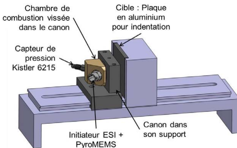
Figure III.24 : Schéma du banc d’essais de propulsion de paillet par nanohermite par indentation sur plaque d’aluminium.
