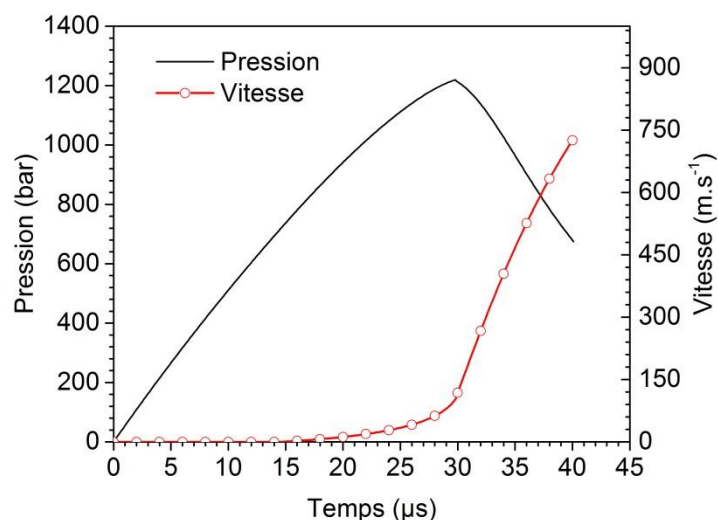
Figure III.22 : Evolution temporelle de la pression et de la vitesse théorique lors de la propulsion du paillet.
