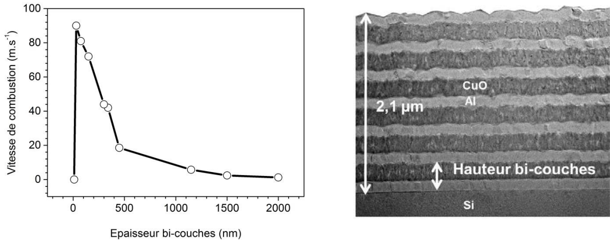
Figure II.19 : (à gauche) Courbe de la vitesse de combustion en fonction de l'épaisseur d'un bi-couches pour une hauteur de nanothermite de 2,1 µm constante ; (à droite) illustration d'un bi-couches sur un dépôt de 2,1 µm.
