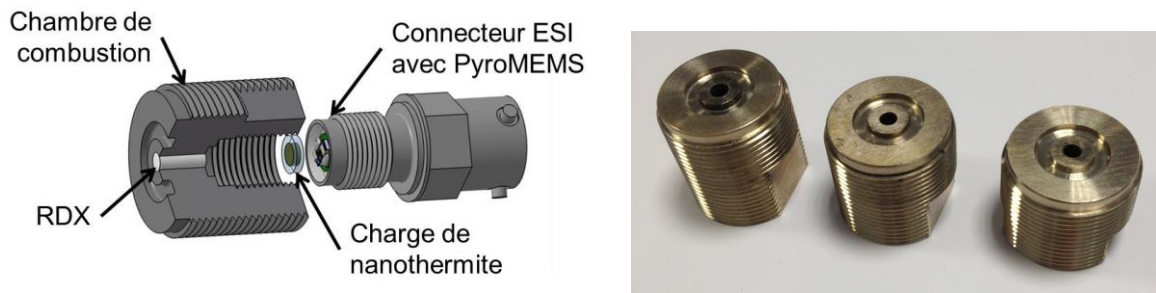
Figure IV.4 : (à gauche) Schématisation éclaté 3D en coupe d'une chambre non instrumentée avec les substances pyrotechniques et le PyroMEMS ; (à droite) Photo des chambres de combustion non instrumentées [IV.1].
