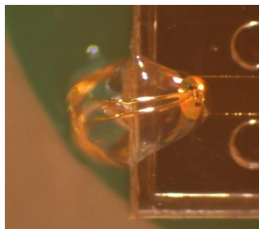
Figure I.23 : Photo d'une connexion par wire bonding entre le PyroMEMS et le PCB.
