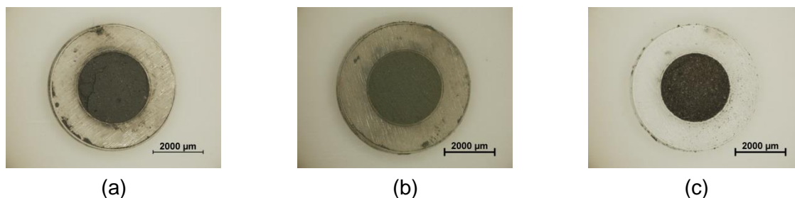
Figure IV.8 : (a) Porte charge Al / CuO ; (b) Porte charge Al / Bi 2 O 3 ; (c) Porte charge ZPP [IV.1].
