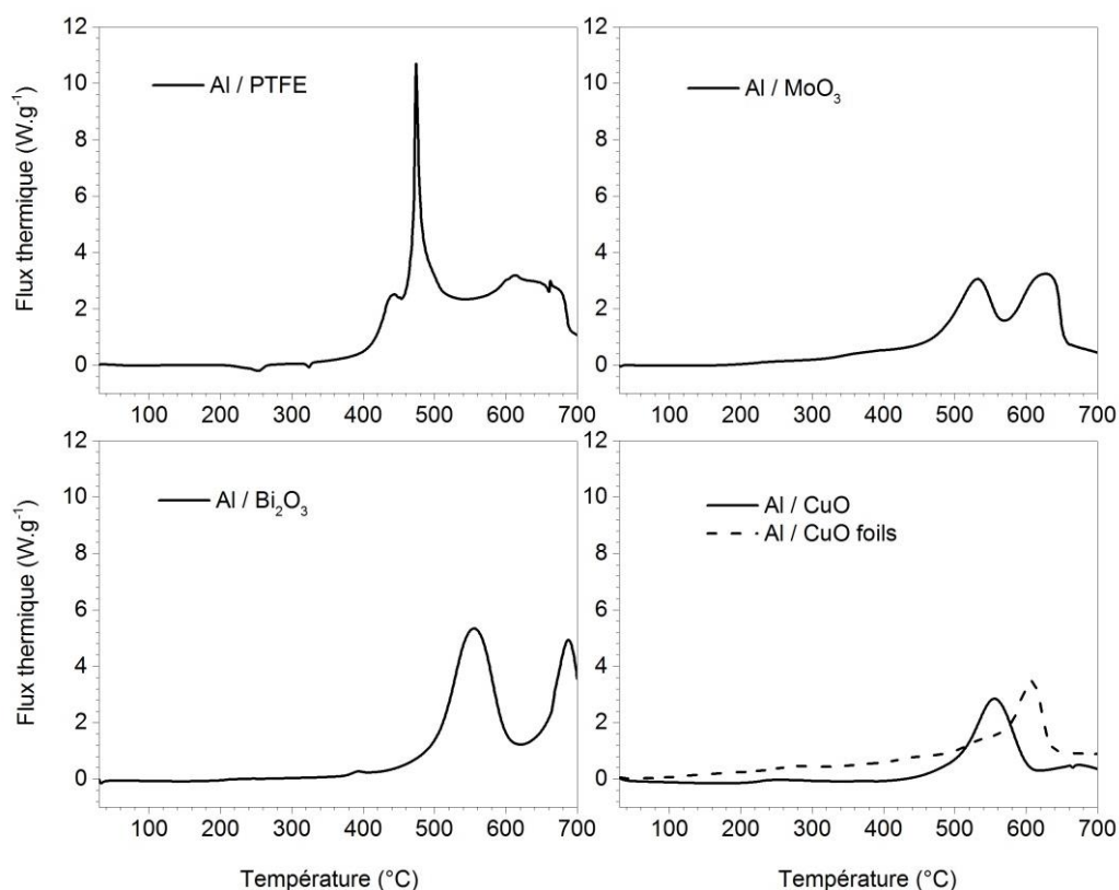
Figure III.8 : Courbes de mesure DSC des nanothermites Al / PTFE ; Al / MoO 3 ; Al / Bi 2 O 3 ; Al / CuO à 10 °C.min -1 .
