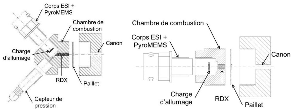
Figure IV.2 : Vue 2D éclatée de la conception : (à gauche) banc d'essai instrumenté d'un capteur de pression et (à droite) chambre de combustion sans capteur de pression.
