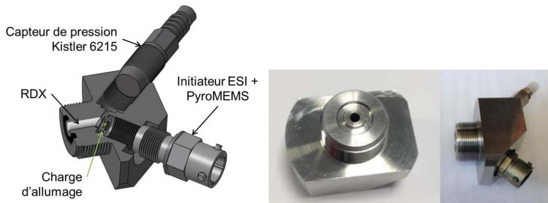
Figure IV.3 : (Gauche) Vue 3D en coupe éclatée de la chambre de combustion instrumentée avec les différents composants du système : l'initiateur, la charge d'allumage, le capteur de pression et le générateur de gaz (RDX). (Droite) Photos de la chambre instrumentée [IV.1].
