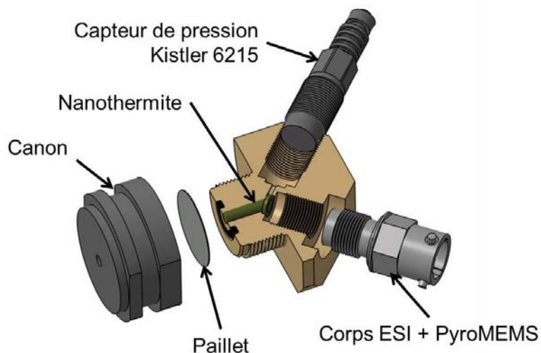
Figure III.23 : Vue éclatée en 3D du canon, du paillet et de la chambre de combustion (en coupe) intégrant de la nanohermite, un initiateur et un capteur de pression Kistler 6215.
