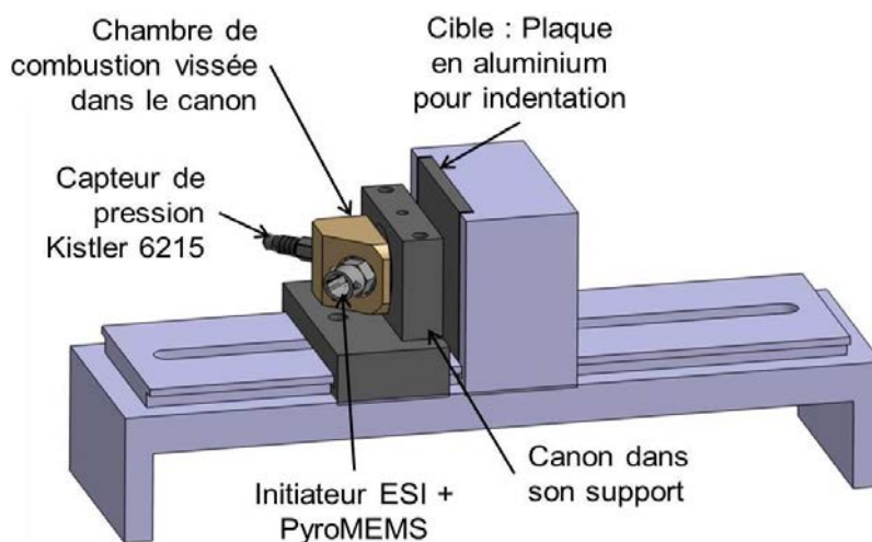
Figure III.24 : Schéma du banc d'essais de propulsion de paillet par nanohermite par indentation sur plaque d'aluminium.
