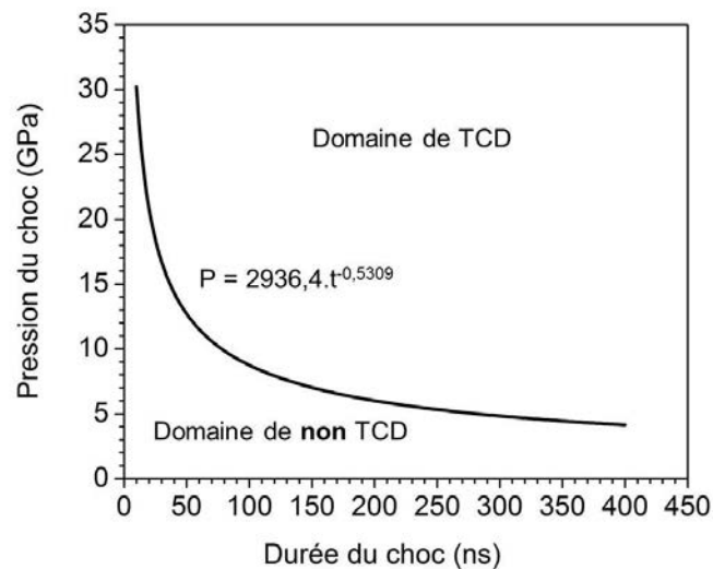
Figure II.8 : Courbe seuil d'amorçage en détonation avec une loi empirique P = f(t) liant la pression du choc P en fonction de la durée du choc t réglée par l'épaisseur du projectile pour de l'octogène (HMX) en composition X1 [II.2].
