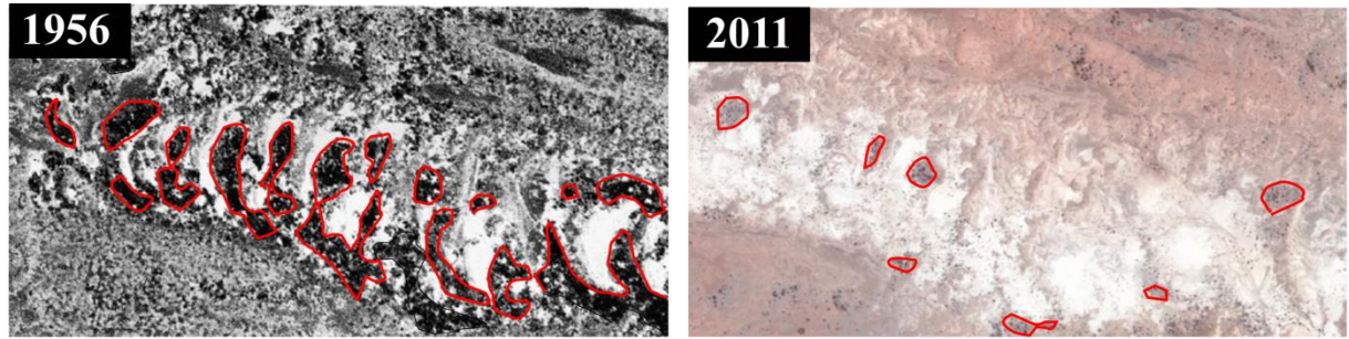
Figure 33: Exemples de changements observés sur les affleurements et les glacis d'érosion (identifiés en rouge) entre 1956 et 2011. De haut en bas, l'extension des placages limoneux et la dégradation (disparition) de la brousse tigrée.
